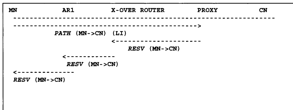
Figure 2.9 Réserve lors d'une relève avec réparation locale (transfert montant)
