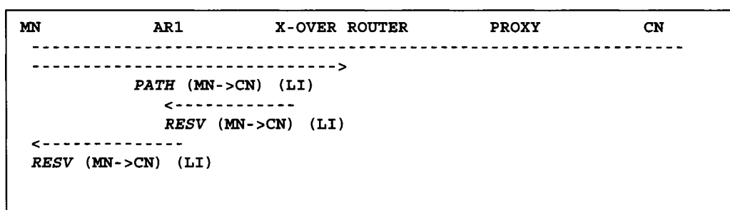
Figure 2.8 Réserve lors d'une relève avec réparation locale (transfert montant)
