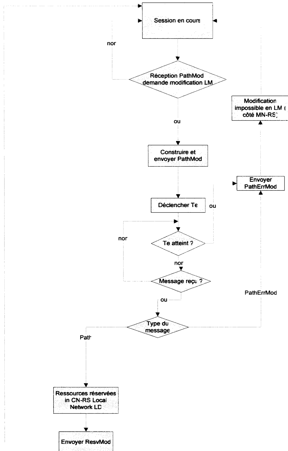
Figure 4.7 Algorithme de modification unidirectionnelle niveau CN_R
