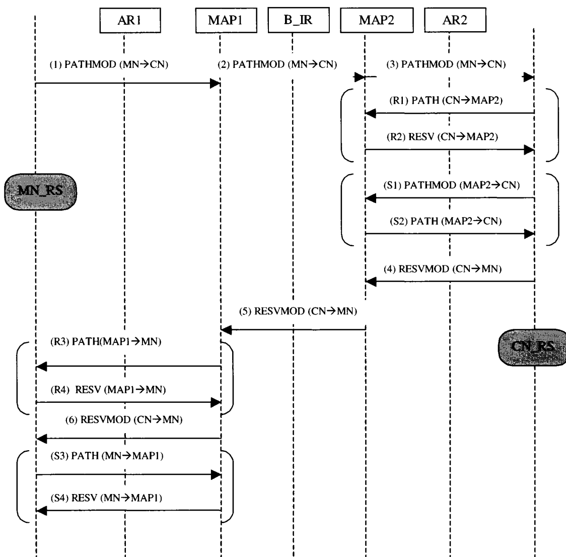
Figure 3.4 Modification de réservation
