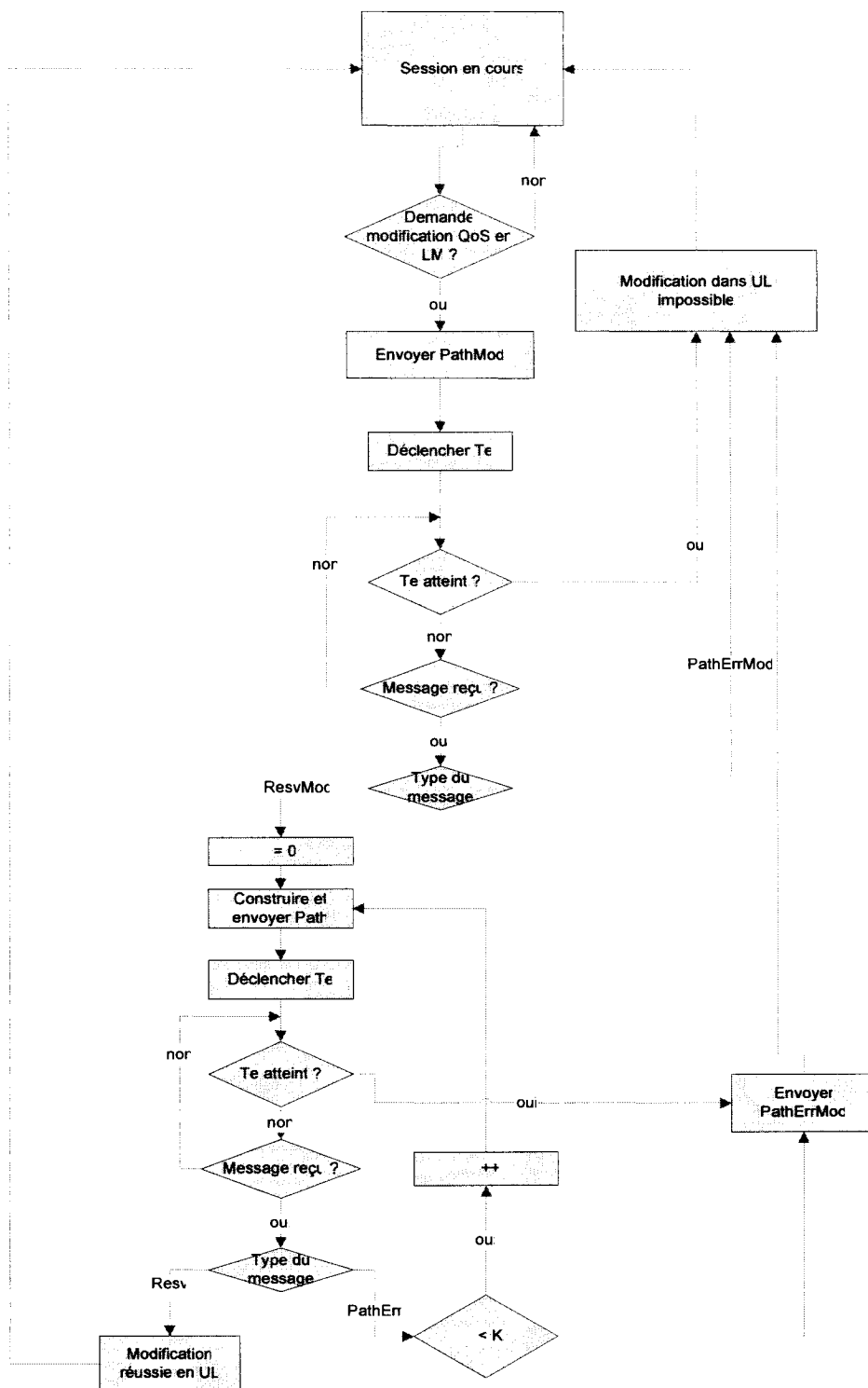
Figure 4.5 Algorithme de modification unidirectionnelle niveau MN_S
