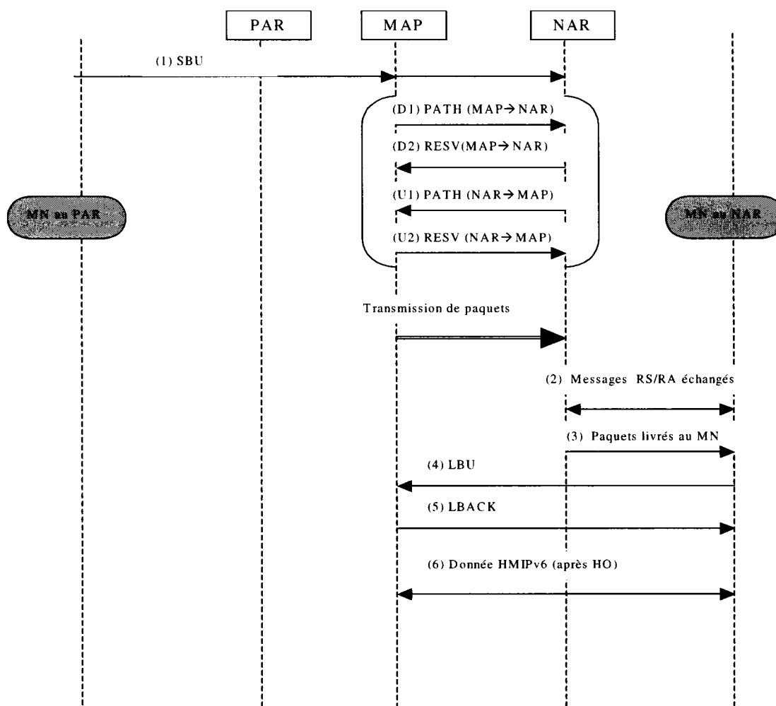
Figure 3.8 SUPER relève intra-domain MAP initié par le réseau sans multicasting
