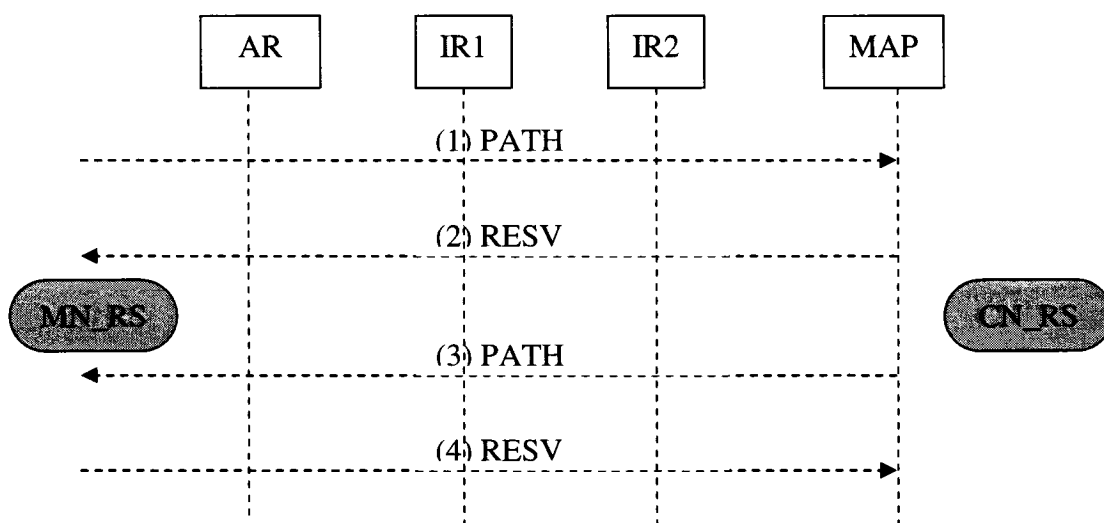
Figure 3.2 Réservation initiale inter-domaine
