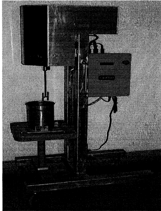
Fig. 3.3 IBB rheometer
