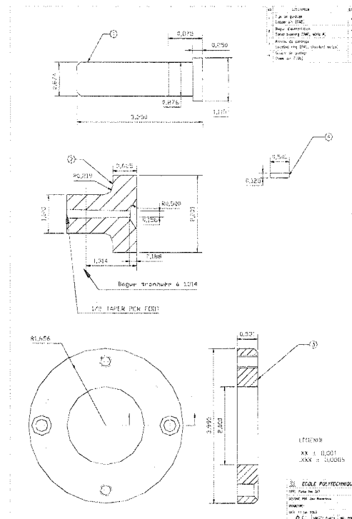
Figure A - 5: Plan des composantes de la nouvelle partie fixe achetées chez DME.
