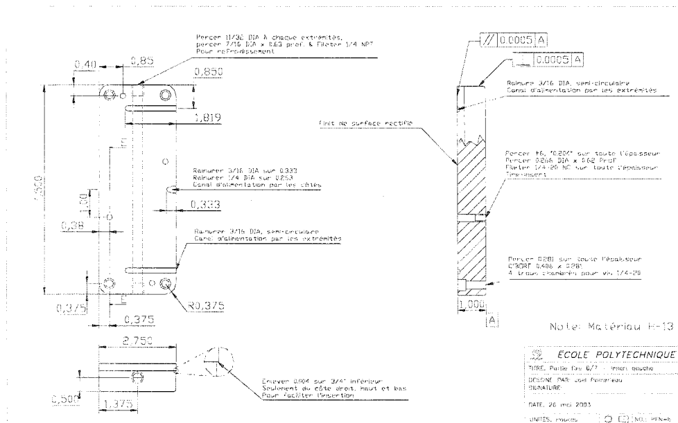
Figure A - 6: Insert plein (gauche) pour la nouvelle partie fixe.
