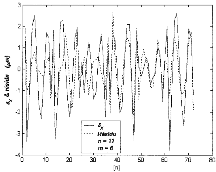
Figure A.7.21 - Mesure filtrée et résidu pour m=6 ( \delta_X )
