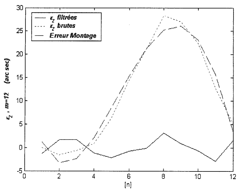
Figure A.2.12 - Filtrage des mesures \varepsilon_z pour m=12
