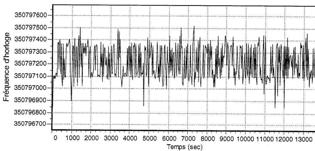
FIGURE 4.3 : Fréquence d'horloge du microprocesseur sur une durée de 4 heures.
