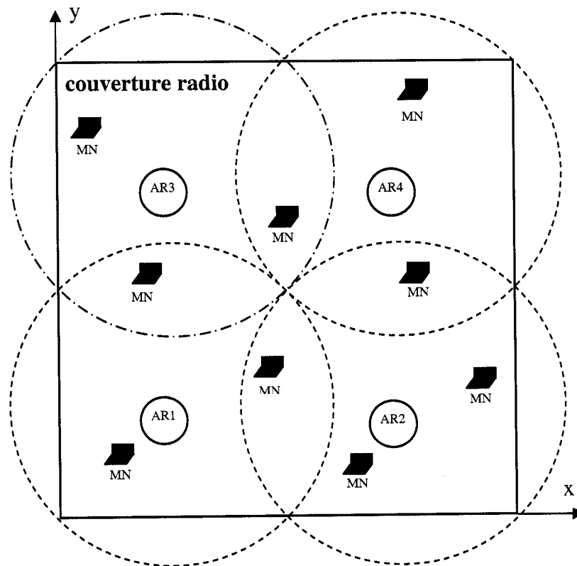
Figure 4.8 Couverture radio des routeurs d'accès
