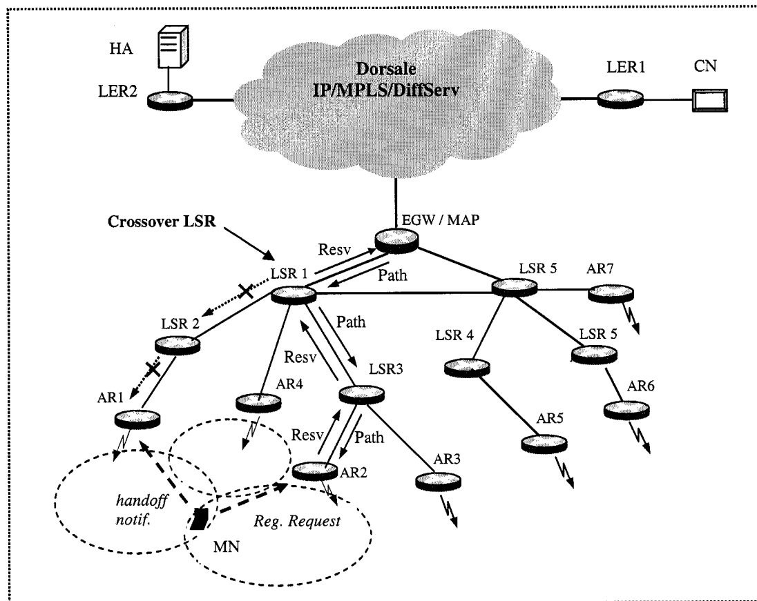
Figure 3.3 Relève intra-RAN
