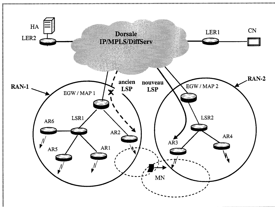
Figure 3.6 Relève inter-RAN
