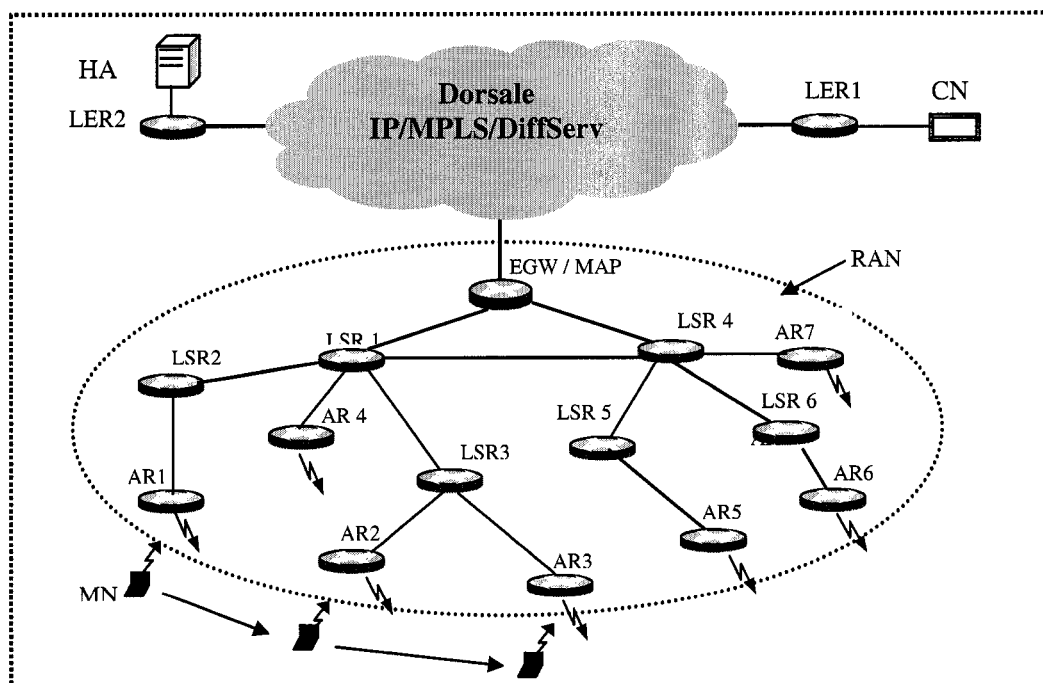
Figure 3.1 Réseau de référence
