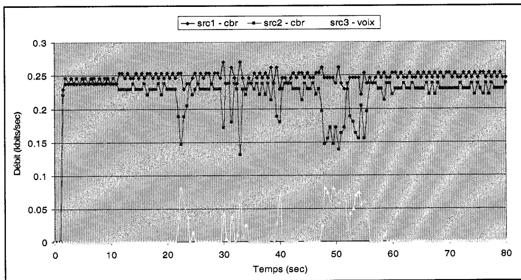
Figure 4.15 Débit reçu par MN – cas de BE-HMIP
