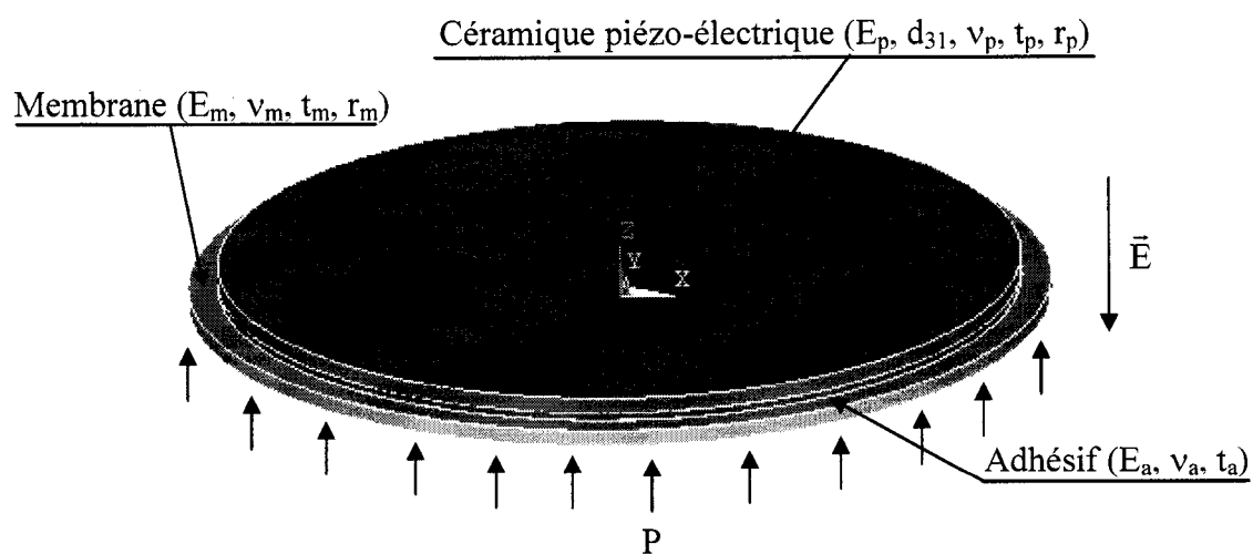
Figure 4.1 : Modèle pour la simulation de la membrane
