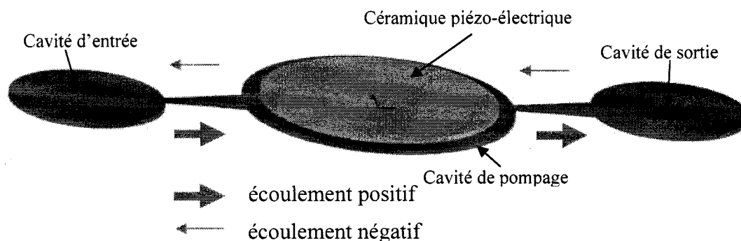
Figure 3.3 : Schéma du dispositif de pompe
