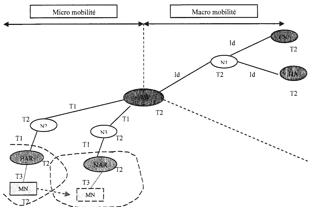
Figure 3.7 Modèle proposé pour l'étude du délai dans un réseau HMIPv6
