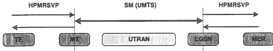
Figure 3.7 Signalisation de qualité de service dans l'architecture UMTS évoluée
