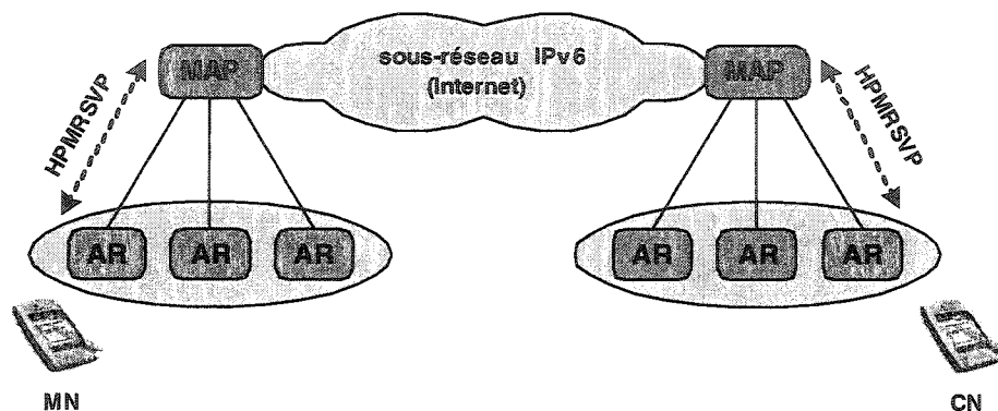
Figure 2.24 Réserveation de ressource inter-domaine avec HPMRSVP
