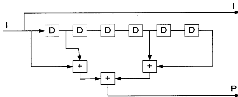
Figure 2.2 Exemple de codeur CSO2C J=4
