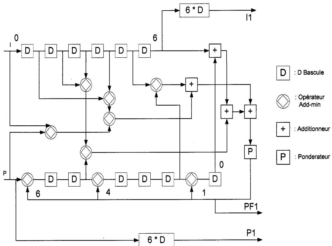
Figure 2.3 Décodeur à seuil avec J=4
