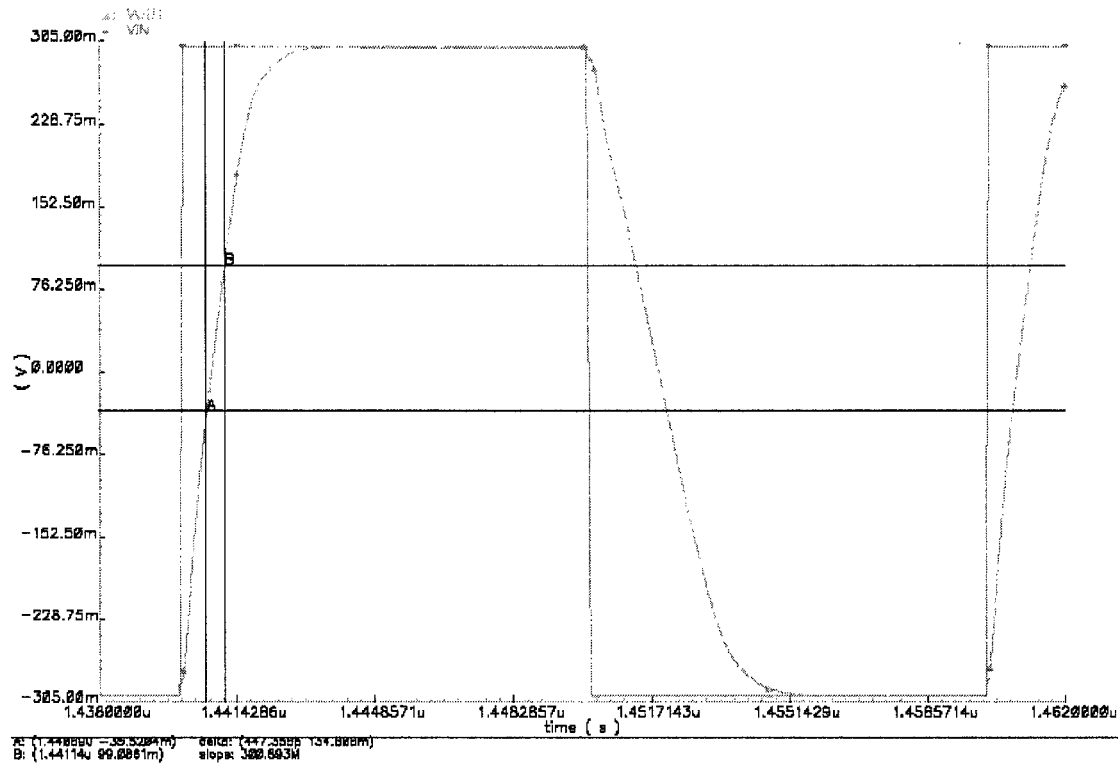
Figure 4-5. Taux de réaction de l'amplificateur.
