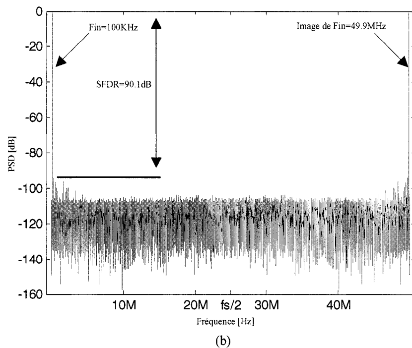
Figure 5-10. FFT du signal de sortie de l'EB avec un commutateur à double amorçage pour, (a) une fréquence d'entrée de 20MHz, (b) une fréquence d'entrée de 100KHz.
