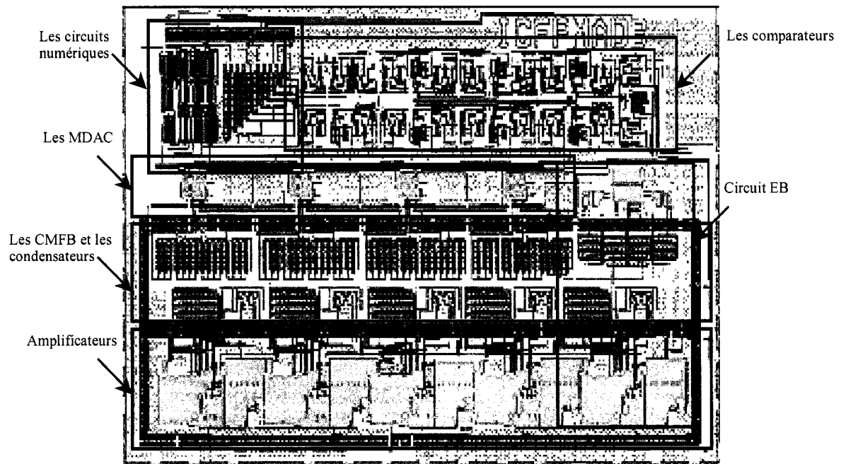
Figure 5-12. La puce du CAN envoyée pour fabrication.
