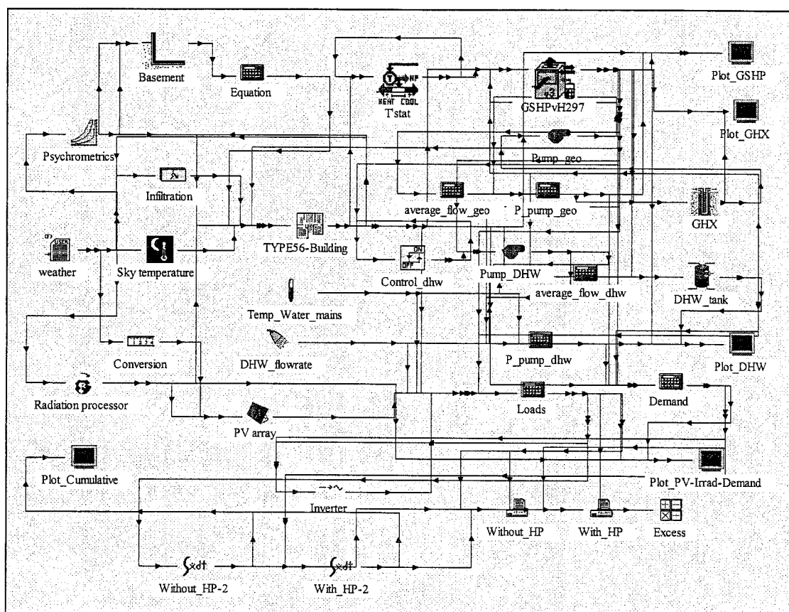
Figure 4.3: Fenêtre d'assemblage du projet dans IISiBat
