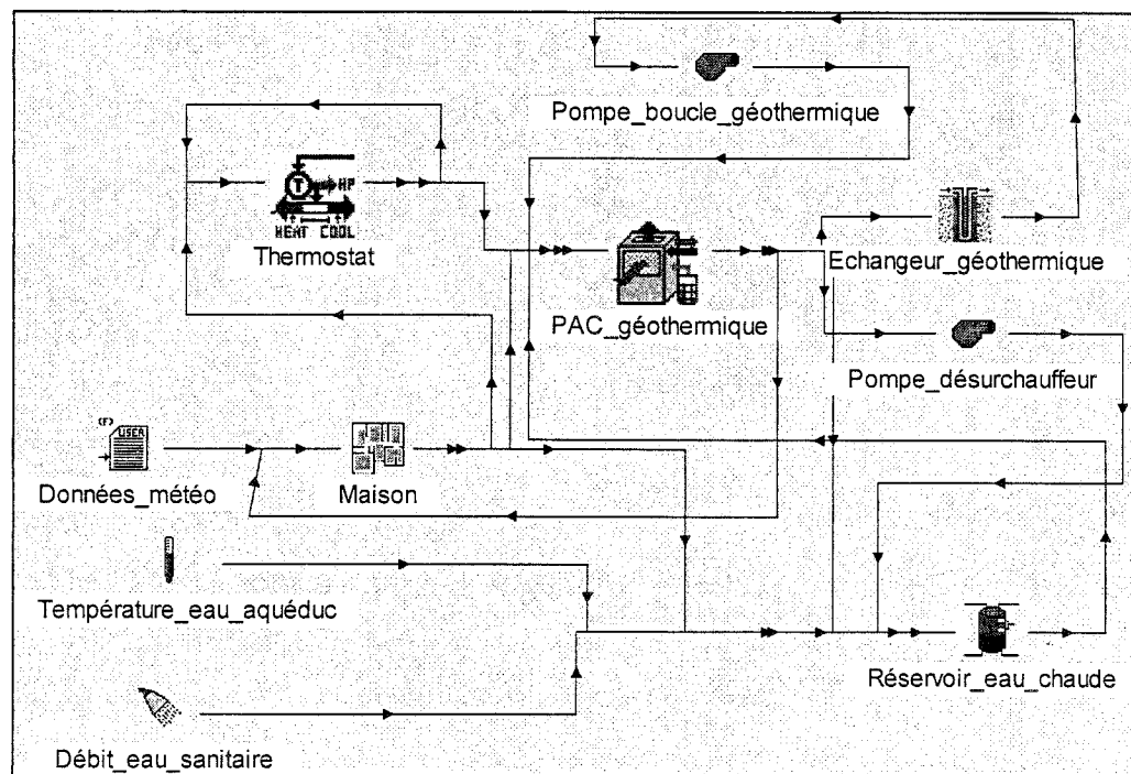
Figure 5.1: Représentation du système de chauffage/climatisation dans IISiBat
