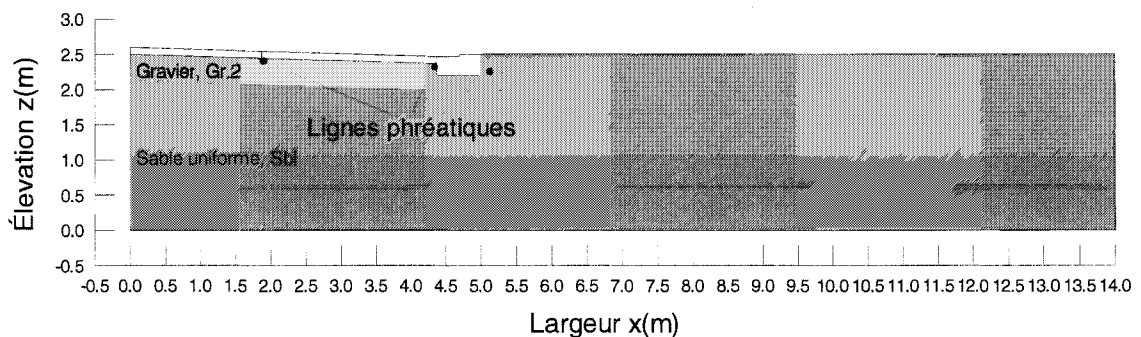
Figure 5-47 Variation de la ligne phréatique en fonction du temps (h) suite à 24 heures de précipitation. Cas de la simulation S-23.
