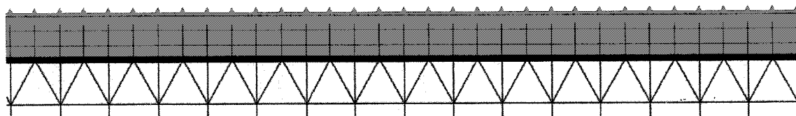
Figure 5-5 Maillage des éléments utilisé pour la modélisation numérique au voisinage de la surface du terrain avoisinant. Cas de base.
