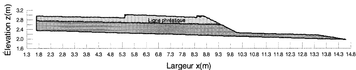
Figure 6-12 Position de la ligne phréatique à 24 heures. Cas de la simulation S-32.
