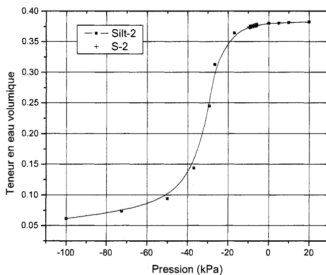
Figure 5-9 Comparaison entre la courbe de rétention d'eau du silt.2 rentrée dans le modèle et les résultats obtenus suite à une heure de précipitation. Cas de la simulation S-2.
