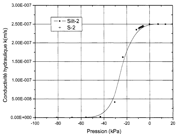
Figure 5-8 Comparaison entre la courbe de conductivité hydraulique du silt.2 rentrée dans le modèle et les résultats obtenus suite à une heure de précipitation. Cas de la simulation S-2.
