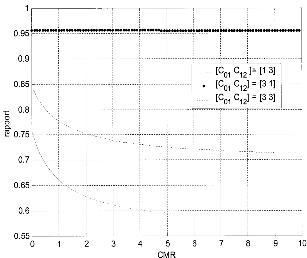
Figure 4.1 Rapport des coûts des procédures de gestion de localisation en fonction du CMR (coûts d'accès aux bases de données nuls avec p = 0.3 )
