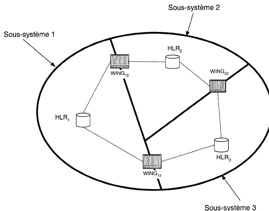
Figure 2.10 Schéma d'interconnexion des HLRs selon l'architecture proposée
