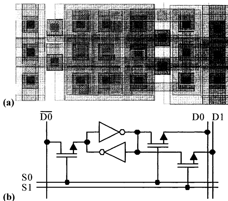
Figure 3.11: Cellule de mémoire statique à deux ports (a) dessin des masques; (b) schéma des transistors.
