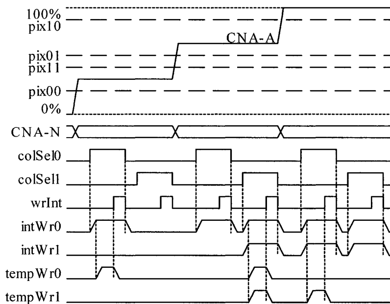
Figure 2.3: Séquence lecture/écriture pour une image.
