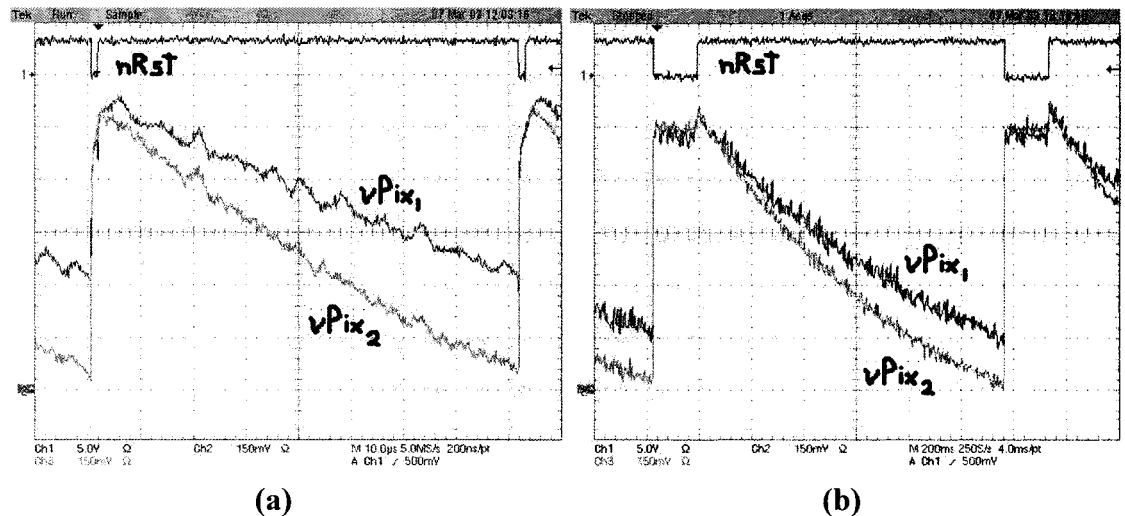
Figure 4.11: Intensité du photo-courant de la photodiode (a) sous forte intensité lumineuse; (b) sous obscurité.
