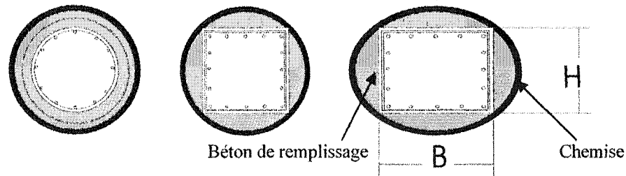
Figure 2.20 – Renforcement à l'aide de chemise
