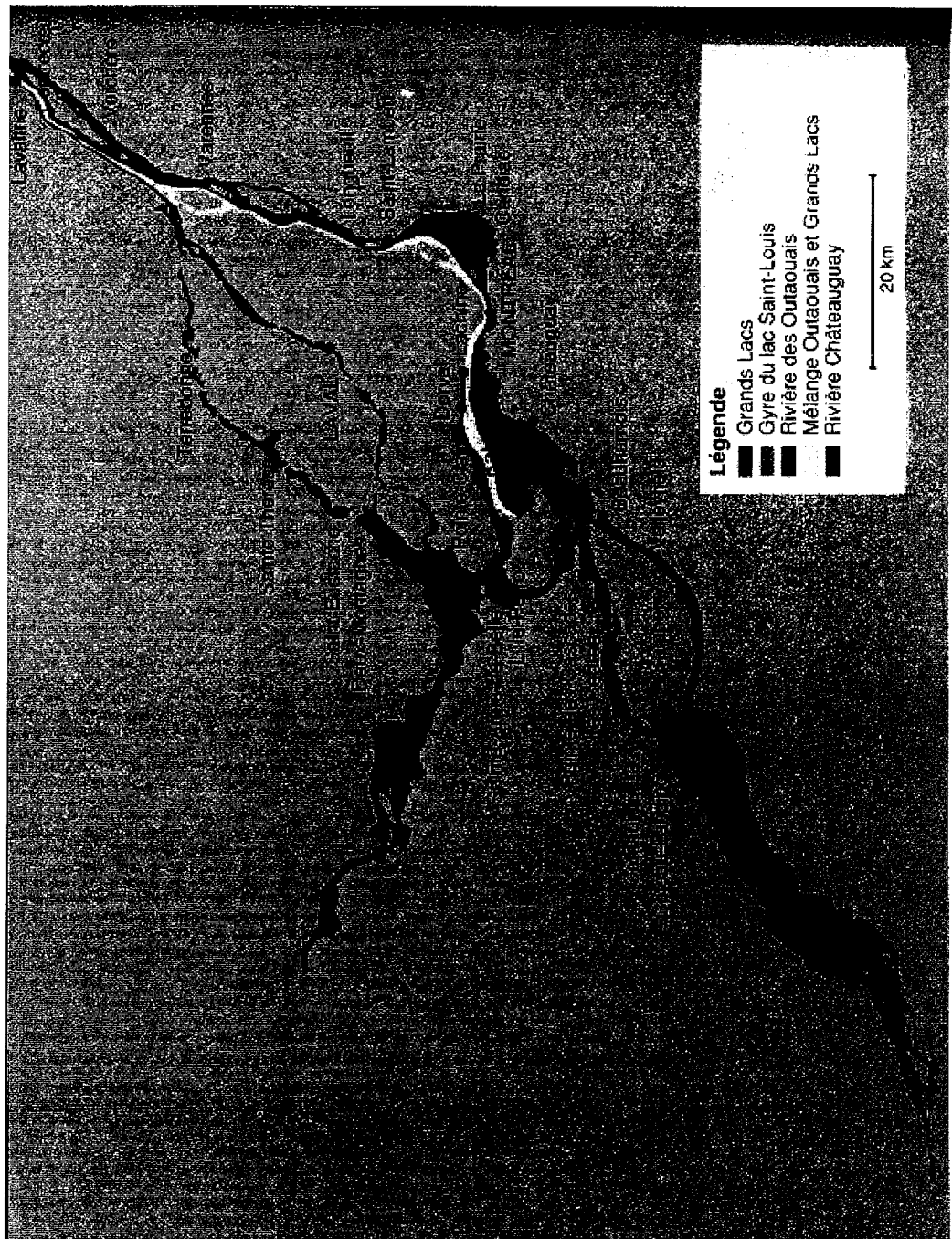
Figure 1-4 : Emplacement des quatre masses d'eau dans l'ensemble du couloir fluvial du lac Saint-François aux îles de Sorel et des prises d'eau dans le fleuve Saint-Laurent, le long du couloir fluvial (Source : Lamarche, 1992)
