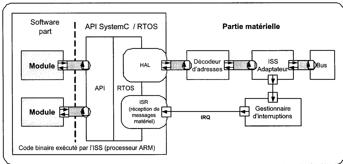
FIGURE 5.11 Fonctionnement de la méthode de réception matérielle
