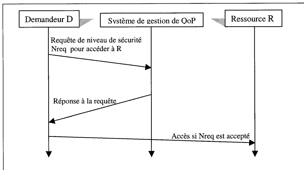
Figure 3.9 Protocole de gestion de QoP
