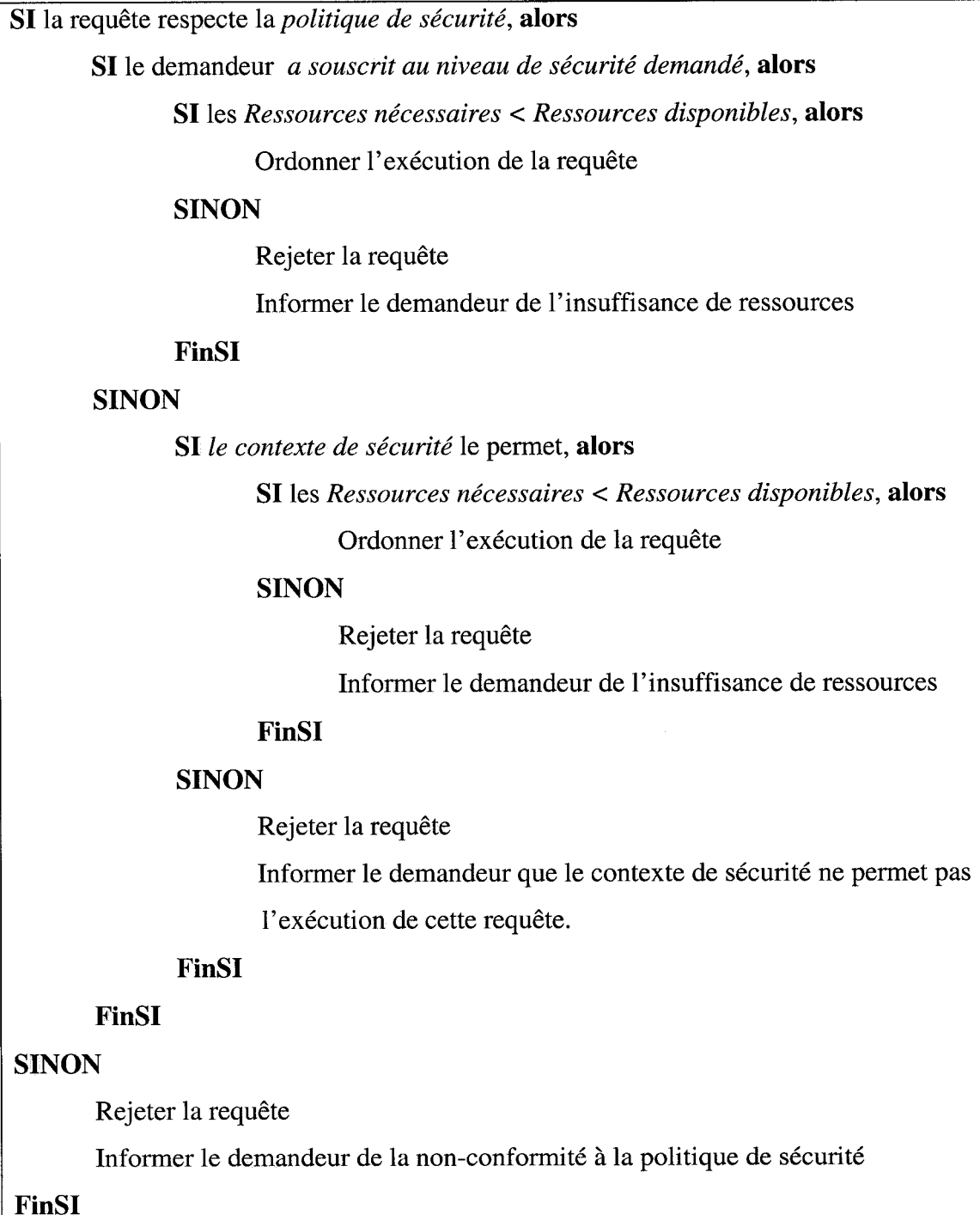
Figure 3.8 Algorithme de décision du niveau de QoP
