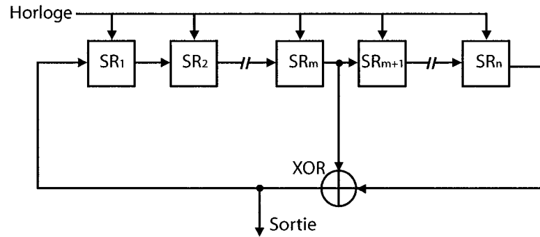
FIG. 2.6 – Génération d'un PRBS.
