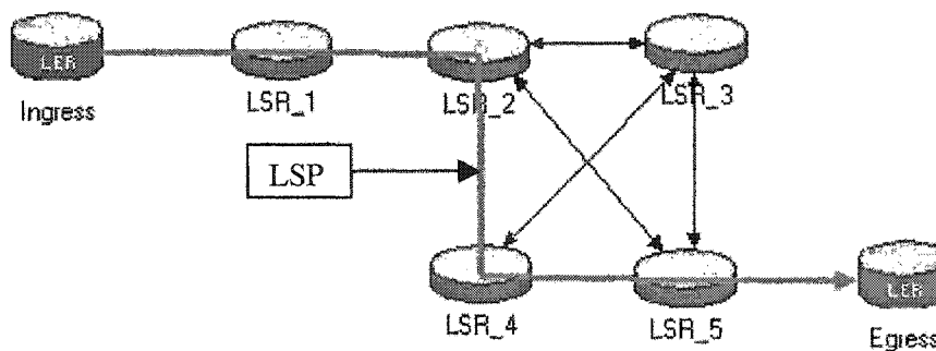
Figure 1.1 Composante d'un réseau MPLS
