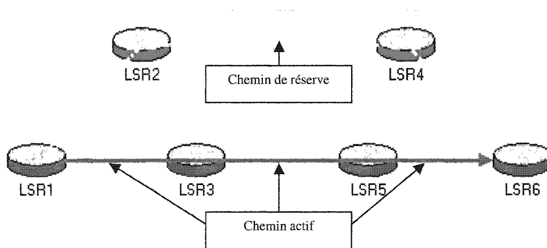
Figure 2.4 Protection Globale (Protection par commutation)
