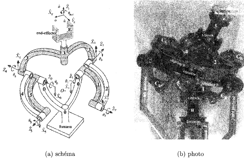
FIGURE 0.9 – Le manipulateur de WIITALA et STANIŠIĆ (2000)
