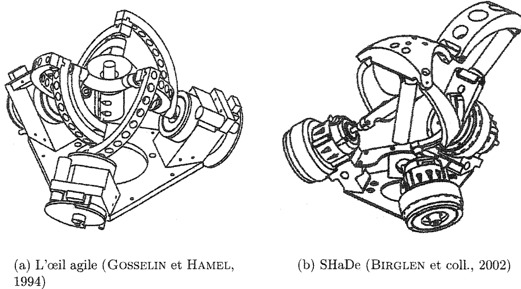
FIGURE 0.8 – Deux réalisations concrètes : l'œil agile et SHaDe.
