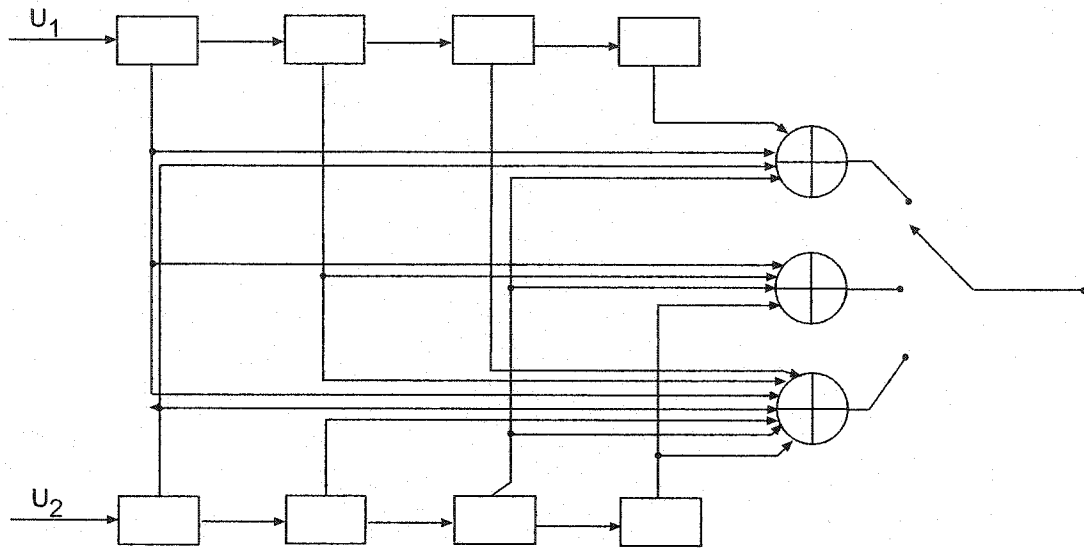
Figure 3.5: Codeur convolutionnel de taux 2/3 : K = 8 , n = 3 , b = 2
