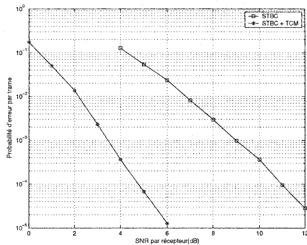
Figure II.22: Comparaison du système STBC et du système STBC concaténé pour une efficacité spectrale de 1 bit/s/Hz; 3 récepteurs; évanouissements rapides
