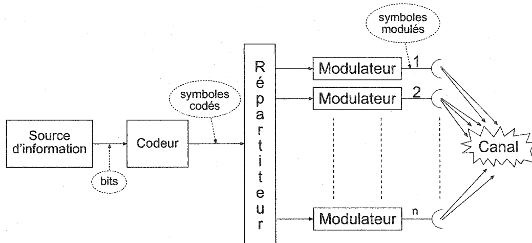
Figure 4.2: Codeur spatio-temporel
