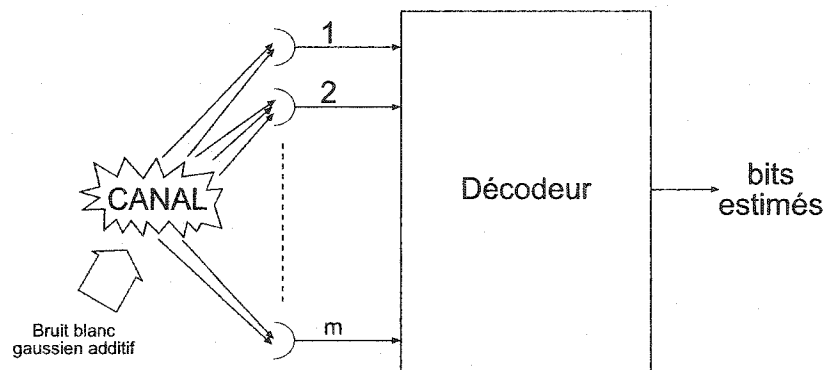
Figure 4.3: Décodeur spatio-temporel
