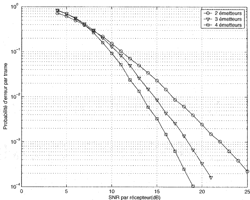
Figure 5.1: Influence du nombre d'émetteurs pour une efficacité spectrale de 1 bit/s/Hz; codes G_2 , G_3 et G_4 ; 1 récepteur; évanouissements quasi-statiques
