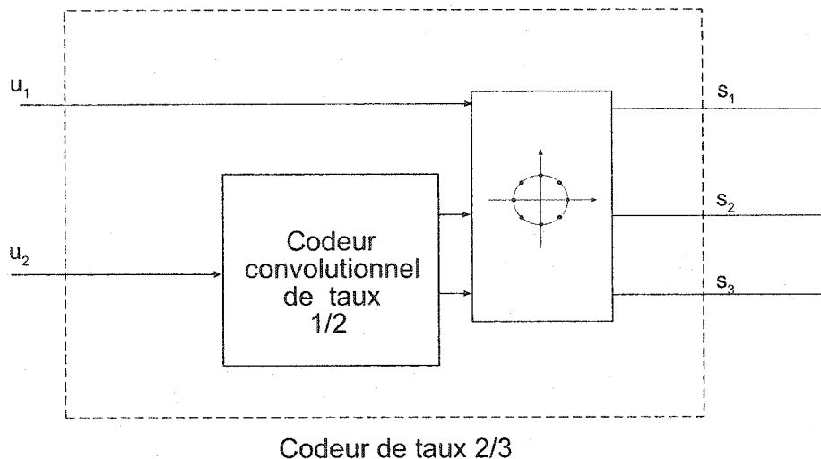
Figure 5.18: Codeur pragmatique de taux 2/3
