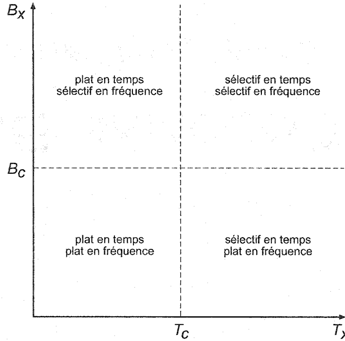
Figure 2.5: Classification des différent types de canaux à évanouissements
