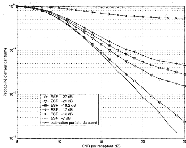
Figure II.14: Erreur d'estimation additive; 2 émetteurs, 1 récepteur, code G_2 ; efficacité spectrale 1 bit/s/Hz; évanouissements rapides
