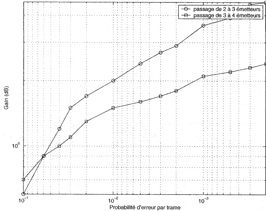
Figure 5.4: Gain en réception pour une efficacité spectrale de 1 bit/s/Hz; code G_2 ; évanouissements quasi-statiques
