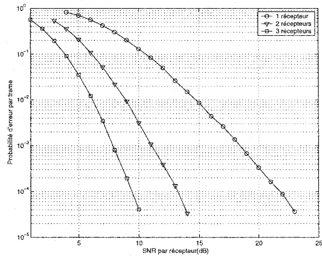
Figure II.6: Influence du nombre de récepteurs pour une efficacité spectrale de 1 bit/s/Hz; code G_3 ; évanouissements quasi-statiques
