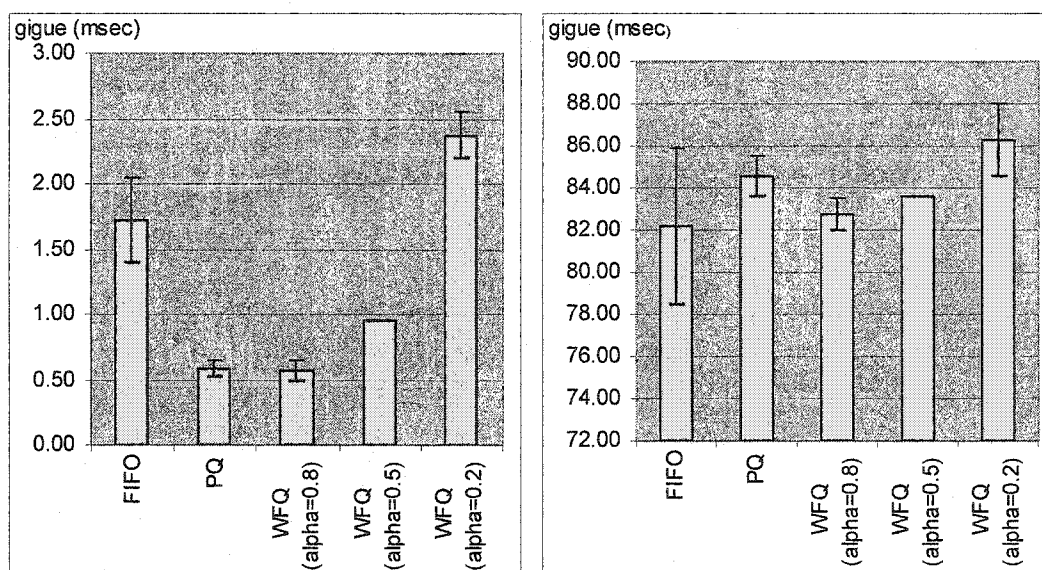
a) Gigue de la voix
