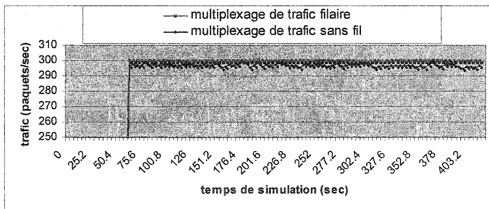
Figure 4.5 Impact de l'accès radio de l'UMTS sur l'agrégation du trafic de voix
