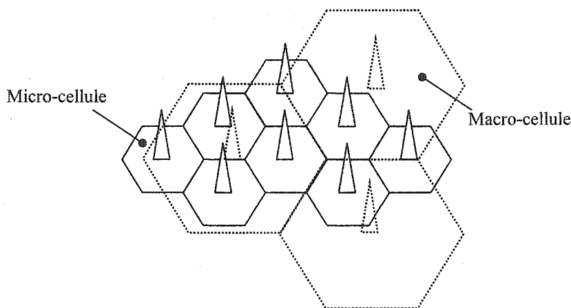
Figure 1.1 Décomposition de la couverture en cellules de différentes tailles
