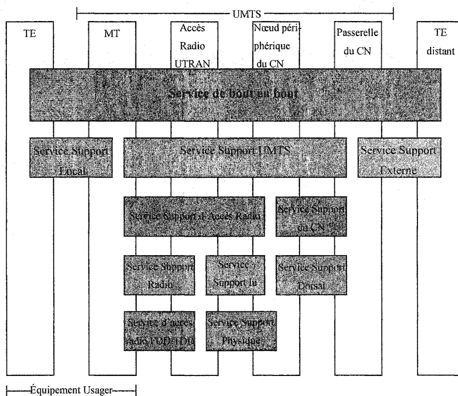
Figure 2.1 Architecture fonctionnelle de la QoS UMTS
