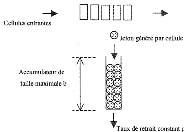
Figure I.2 Filtre en seau percé pour les cellules
