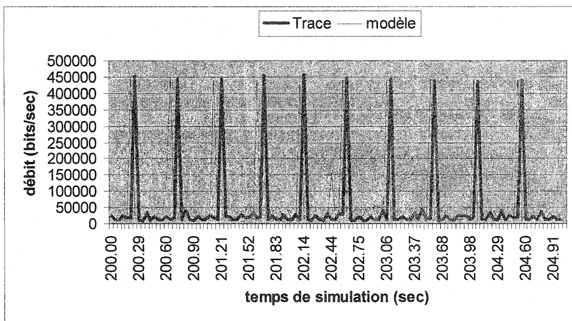
Figure 4.16 Validation du modèle implémenté avec une trace
