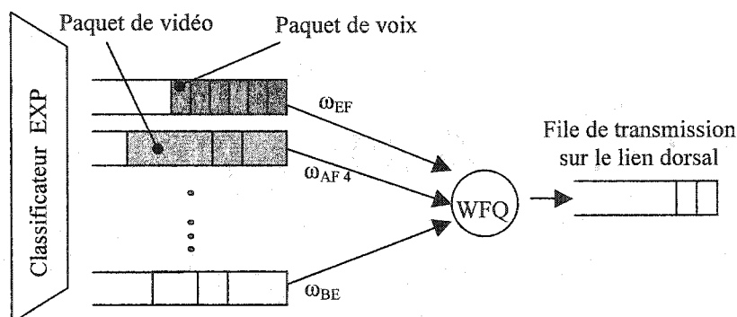
Figure 3.12 Ordonnancement par partage équitable pondéré entre voix et vidéo
