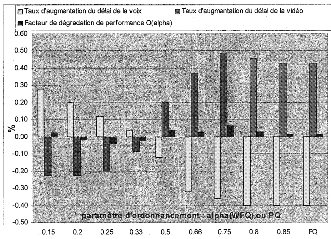
Figure 4.10 Performances attendues en délais en fonction de l'ordonnancement
