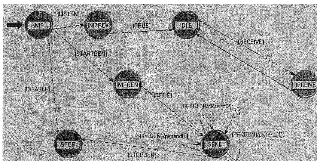
Figure 4.6 MEF d'une source/puits de trafic vidéo
