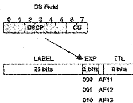
Figure 2.7 Utilisation du champ EXP pour déterminer le PHB
