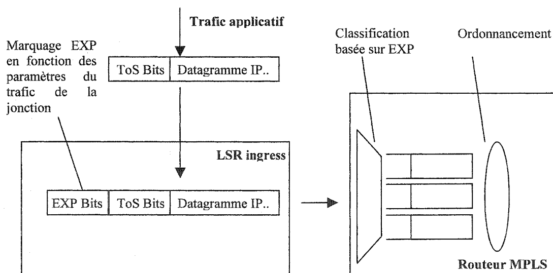
Figure 4.3 Modèle DiffServ sur MPLS
