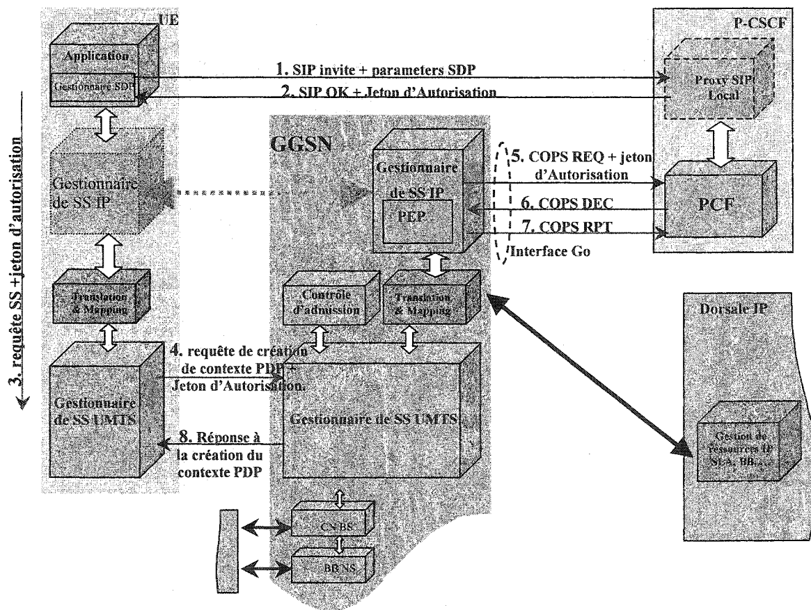
Figure 2.8 Architecture d'inter-fonctionnement du contrôle de QoS de bout en bout
