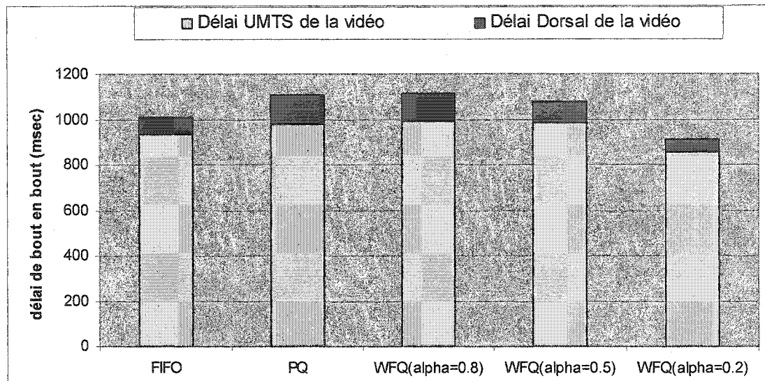
Figure 4.14 Délai Dorsal vs. Délai UMTS du trafic de vidéo téléphonie
