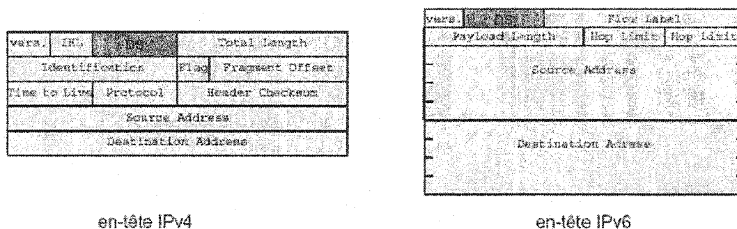
Figure 2.4 Champ DiffServ dans l'entête IP
