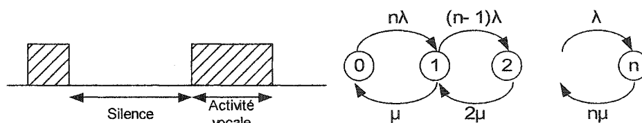
a) Modèle ON/OFF d'un appel simple b) Modèle d'appels multiples
