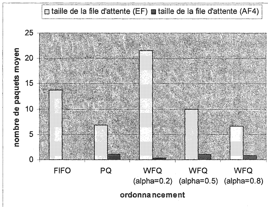
Figure 4.12 Occupation des files d'attente EF et AF4
