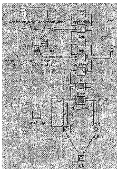
Figure 4.7 Intégration de la téléphonie multimédia dans une station UMTS
