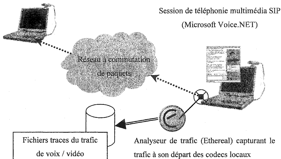
Figure 3.1 Capture des paquets IP d'une session de téléphonie multimédia
