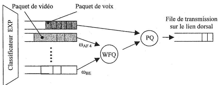
Figure 3.11 Ordonnancement par priorité donnée au trafic de voix
