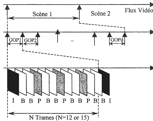
Figure 3.16 Modèle vidéo MPEG
