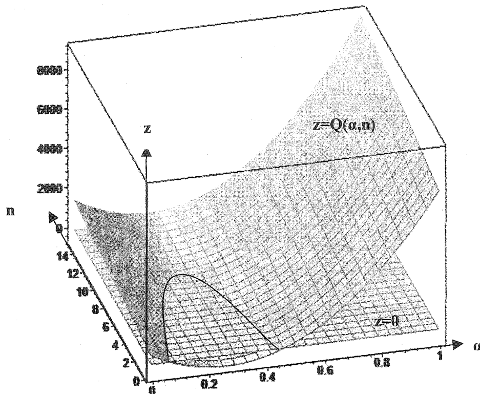
Figure 3.13 Facteur de dégradation de performance Q à minimiser
