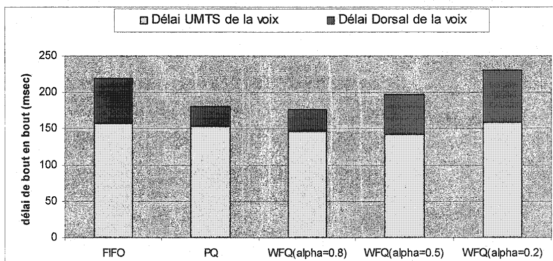
Figure 4.13 Délai Dorsal vs. Délai UMTS du trafic de voix
