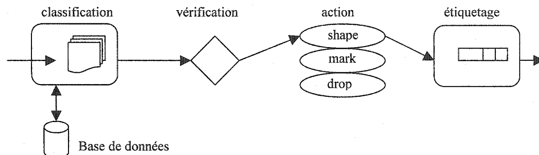
Figure 2.6 Modules d'un routeur d'entrée DiffServ
