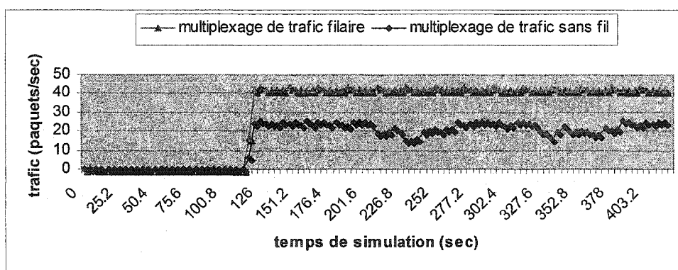
Figure 4.4 Impact de l'accès radio de l'UMTS sur l'agrégation du trafic de vidéo
