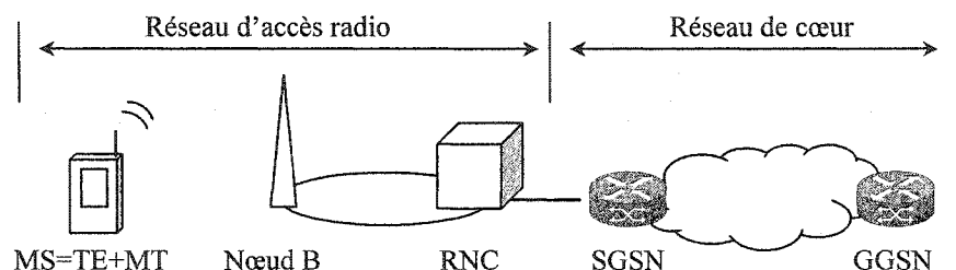
Figure 1.2 Architecture d'un réseau d'accès UMTS
