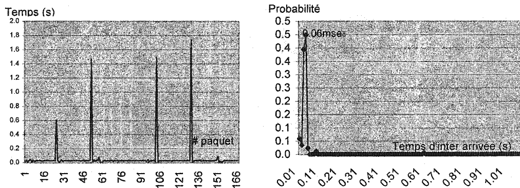
a) Inter-arrivée des paquets de voix
