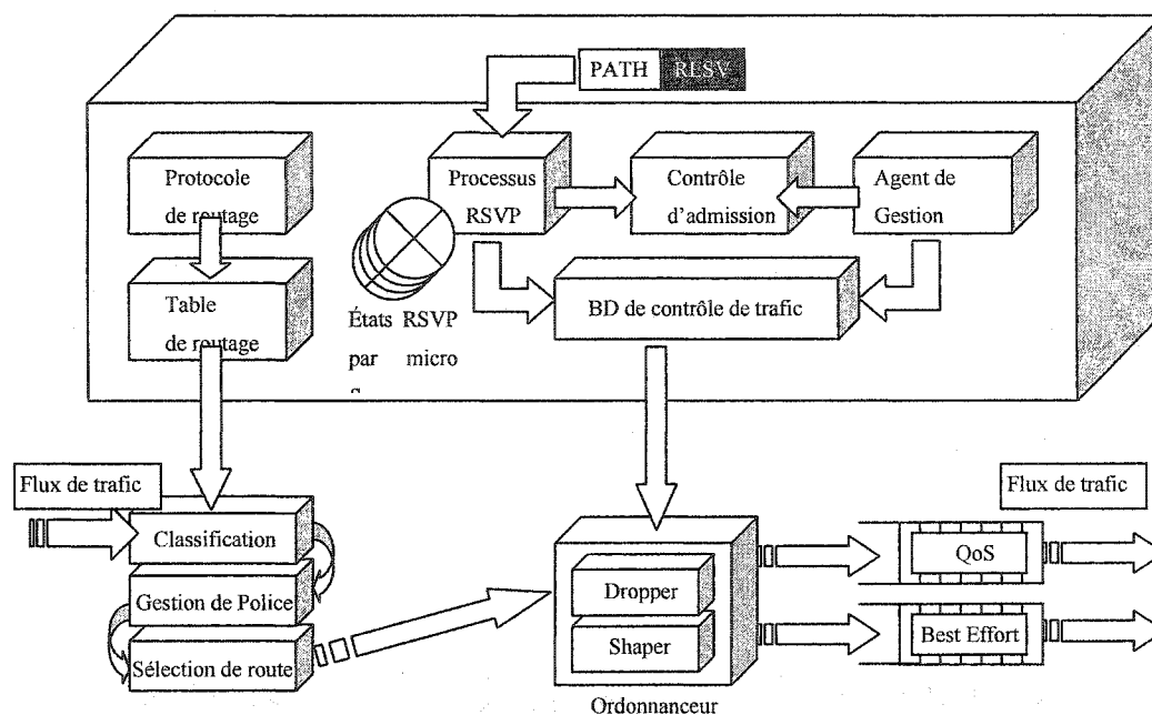
Figure 2.3 Modules d'un routeur IntServ/RSVP
