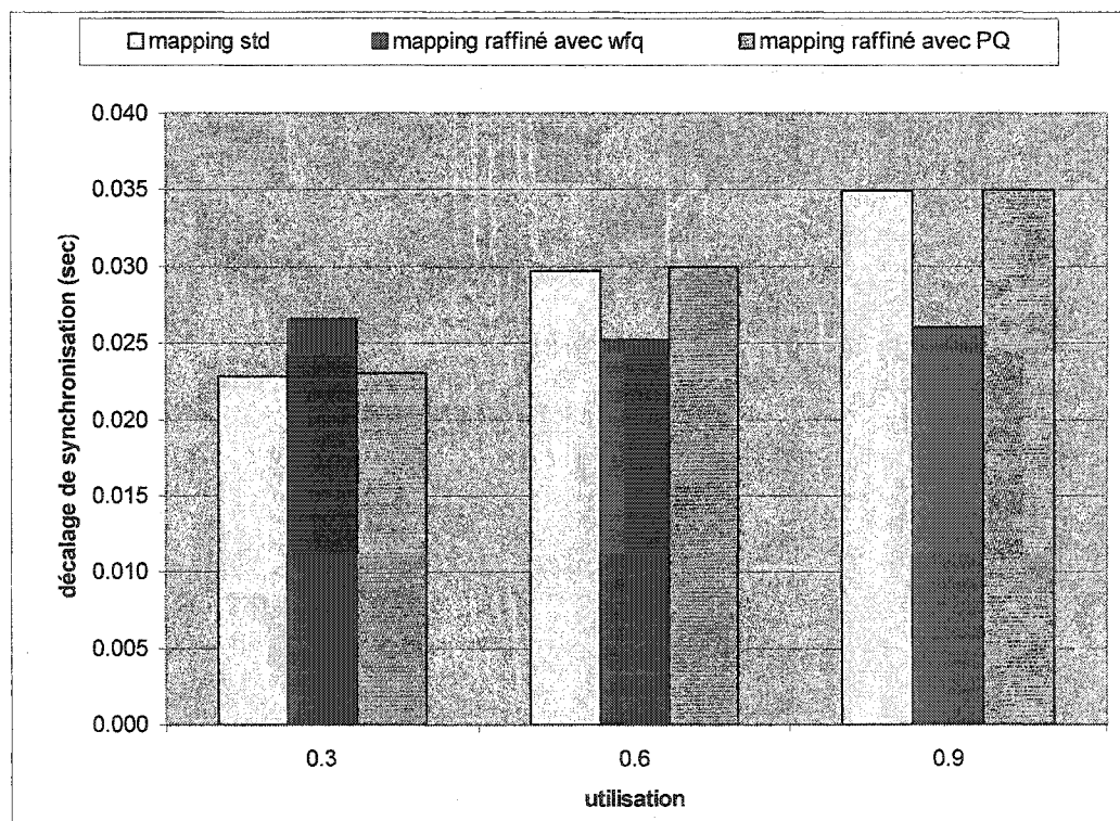
Figure 4.15 Décalage de synchronisation entre voix et vidéo
