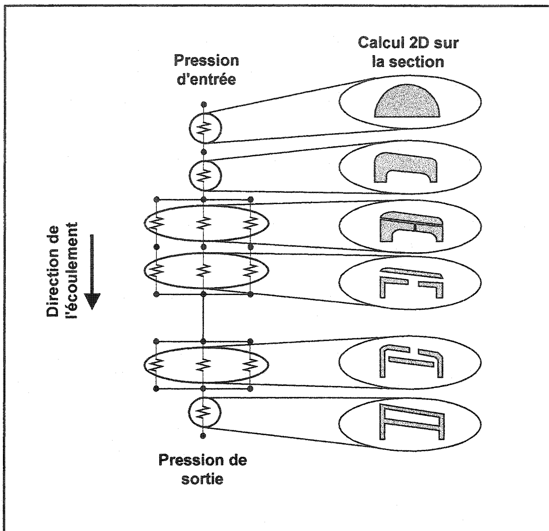
Figure 1.4 : Schéma du calcul 2 \frac{1}{2} D (Adapté de Svabik et al.).
