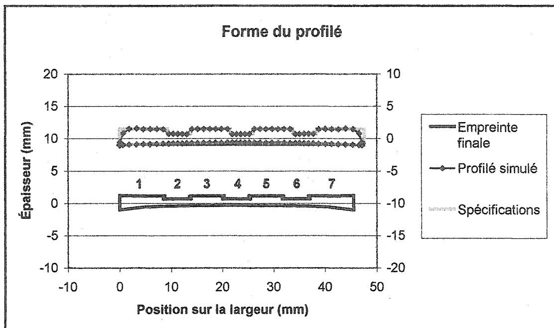
Figure 4.17 : Simulation du profilé final avec la filière conçue initialement.
