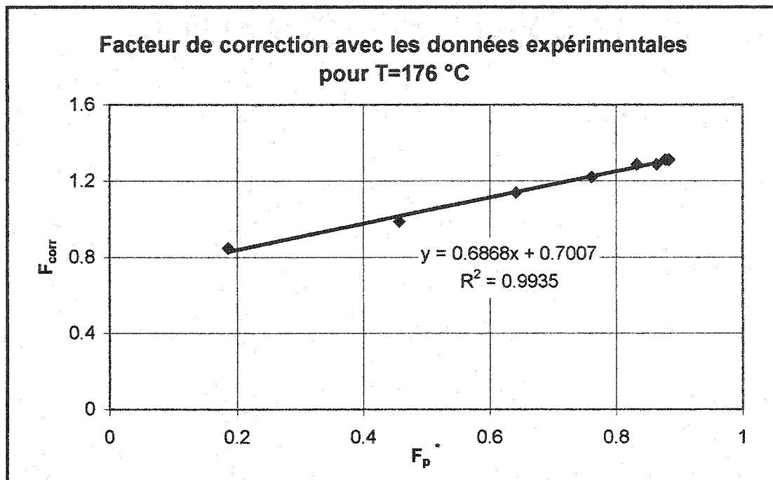
Figure 2.14 : Relation entre F_{corr} et F_p^* , calculé à partir des mesures de l'essai 35.
