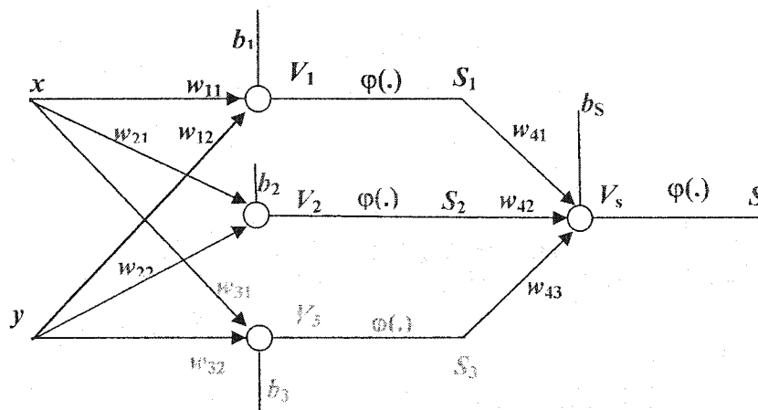
Figure 2.12 Réseau à trois neurones cachés
