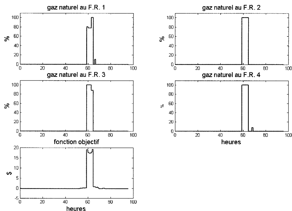
Figure 5.31 : Scénario 2 avec prix du gaz naturel plus bas : gaz naturel aux fours rotatifs et fonction objectif
