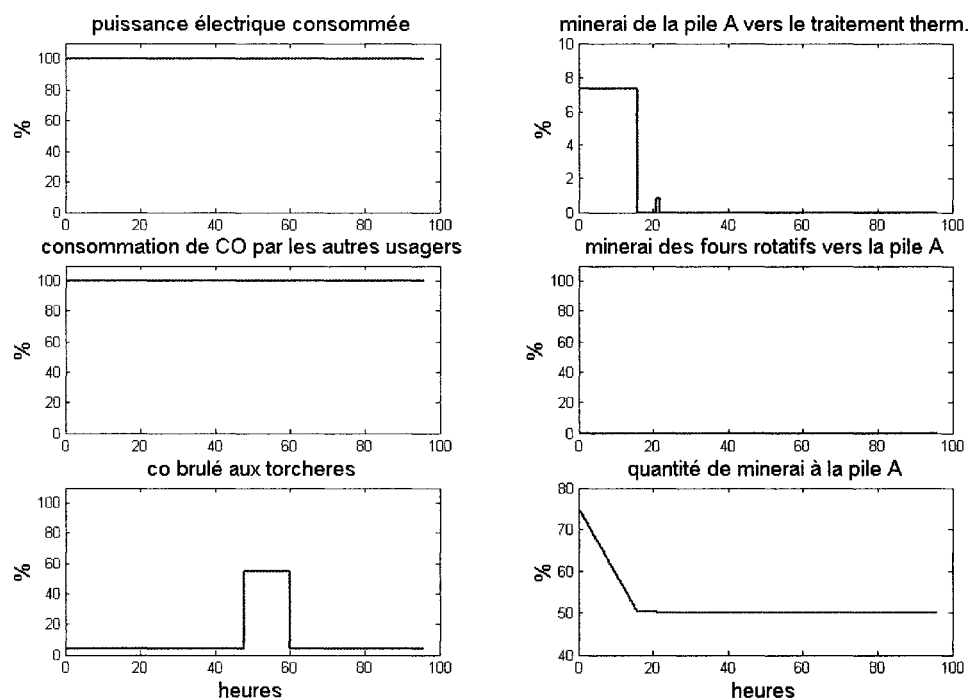
Figure 5.22 : Scénario 1 avec pile B plus basse : puissance disponible, autres usagers de CO, CO aux torchères et pile A
