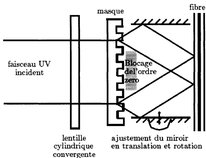
Figure 1.7 : Montage d'écriture à l'aide d'un montage interférométrique utilisant un masque de phase.
