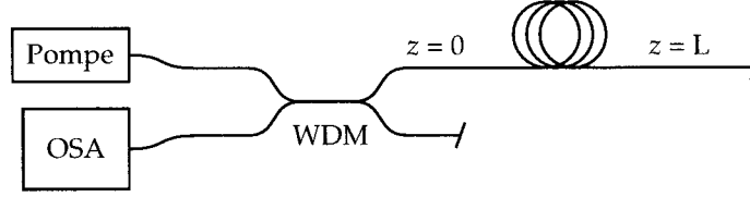
Figure 2.3 : Montage expérimental généralement utilisé lors de la mesure de g_R par la méthode du gain Raman spontané
