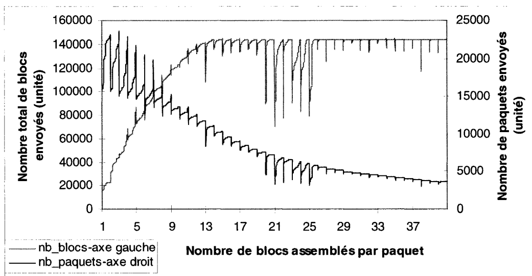
Figure H-2. Variation du nombre de paquets envoyés pour un taux de 30 images/s
