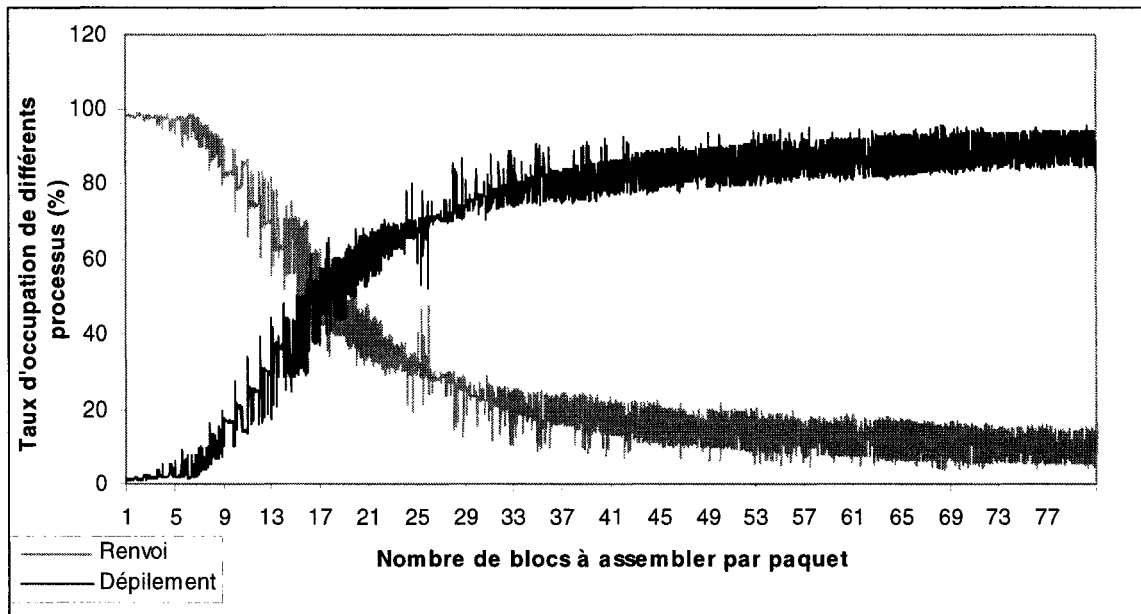
Figure 4-14. Variation de l'occupation des processus de la conversion
