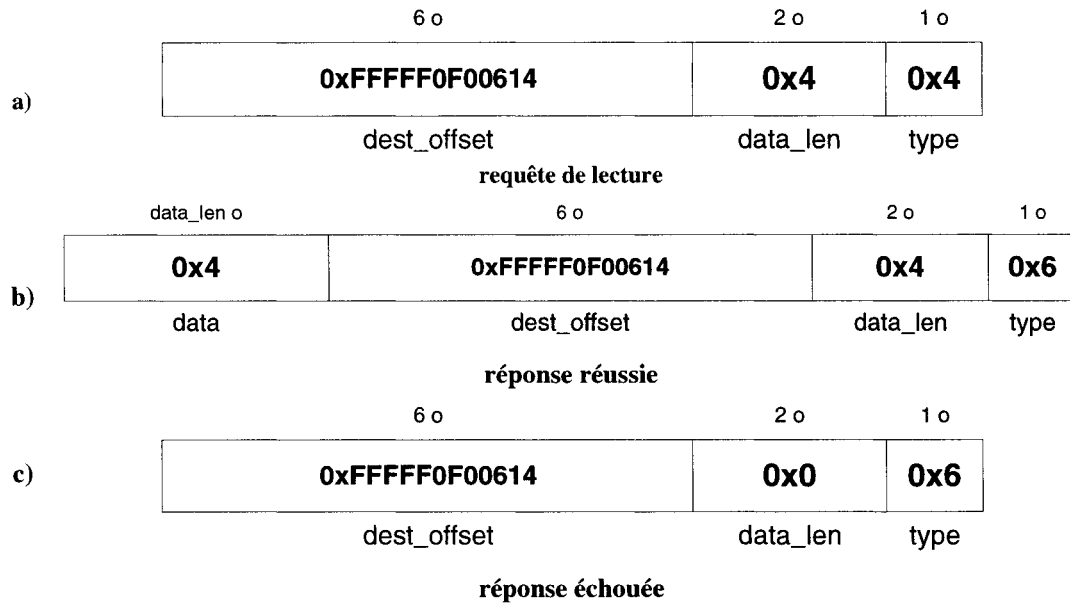
Figure F-3. Contenus de l'entête FireoverIP pour une transaction de lecture
