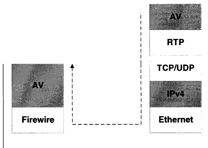
Figure 4-2. Empilement de protocoles d'une caméra numérique à un PC
