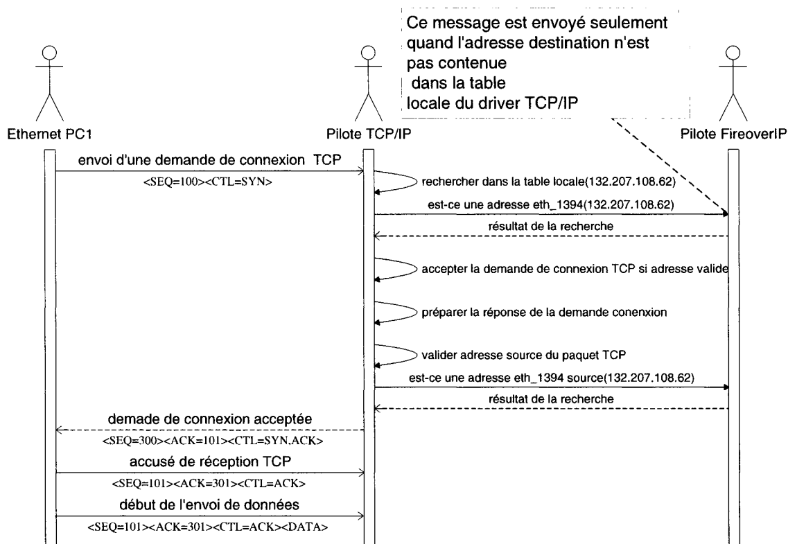
Figure E-5. Séquence d'opérations après la réception d'une demande d'ouverture de session TCP
