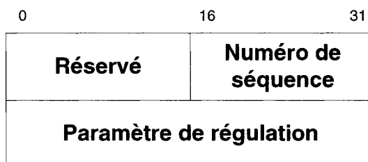
Figure 2-12. Format de l'entête proposé par Ogawa et al. (1999)
