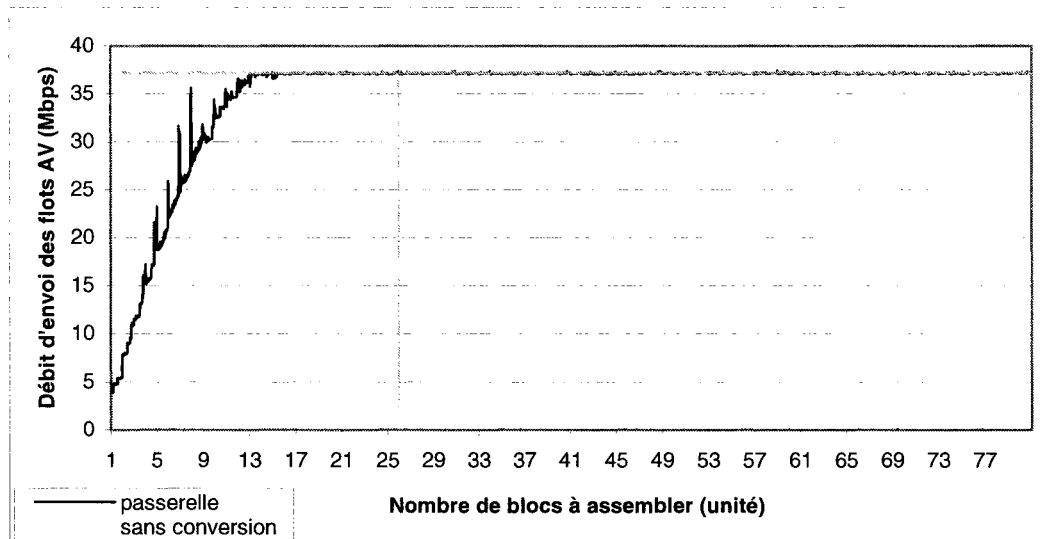
Figure 4-16. Variation de la vitesse moyenne d'envoi des flots AV pour 15 im/s
