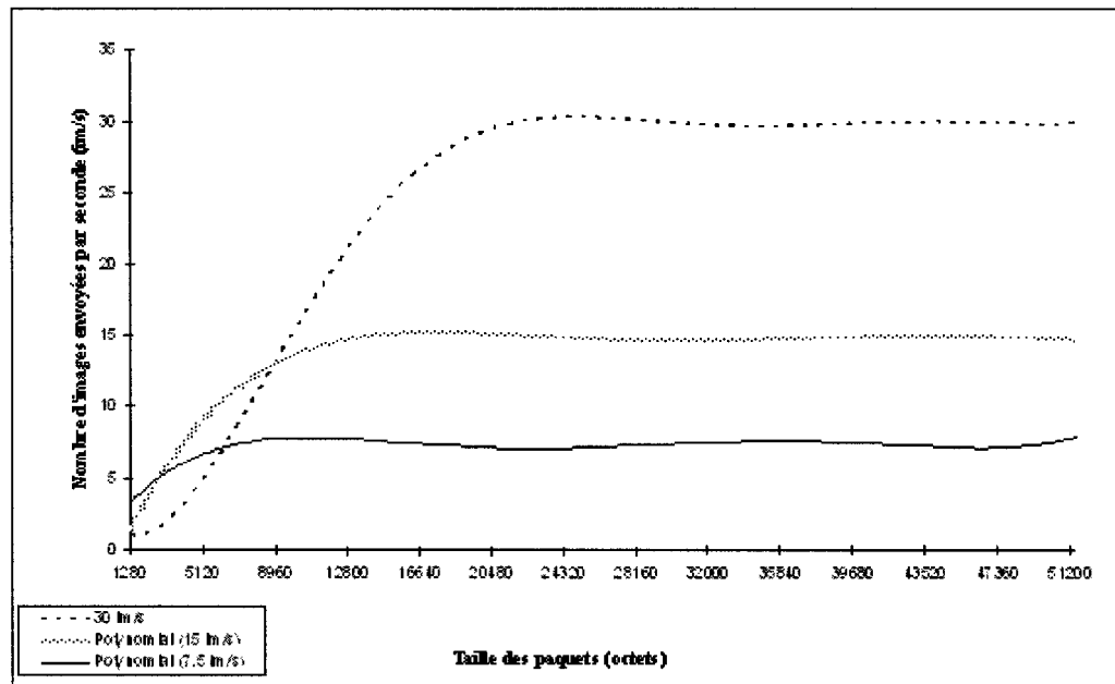
Figure 4-18. Évolution du nombre d'images envoyées
