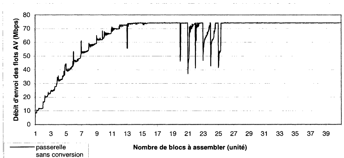
Figure H-4. Variation de la vitesse moyenne d'envoi des flots AV pour 30 im/s
