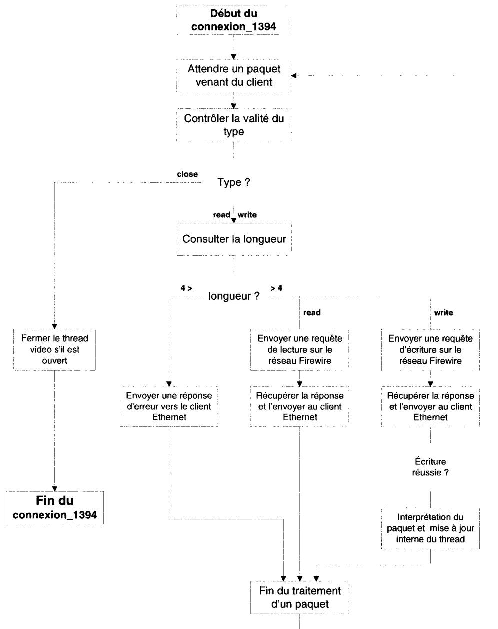
Figure F-2. Organigramme du thread conn_1394
