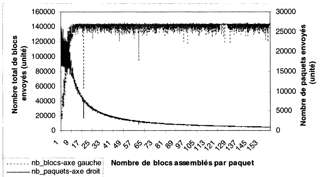
Figure H-1. Variation du nombre de paquets envoyés pour un taux de 7.5 images/s
