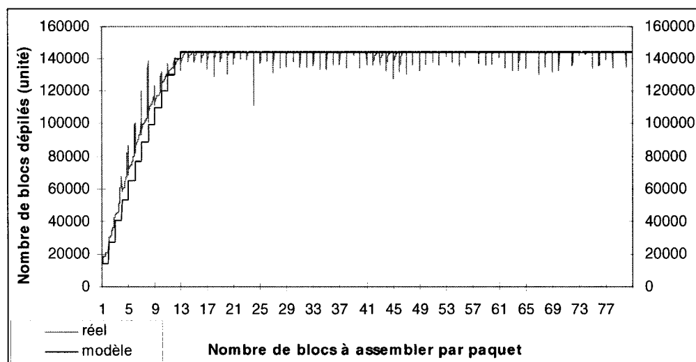
Figure 4-20. Variation du nombre des blocs dépilés
