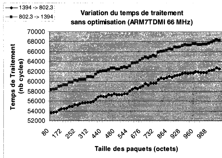
Figure 3-13. Temps de traitement de la solution non-optimisée
