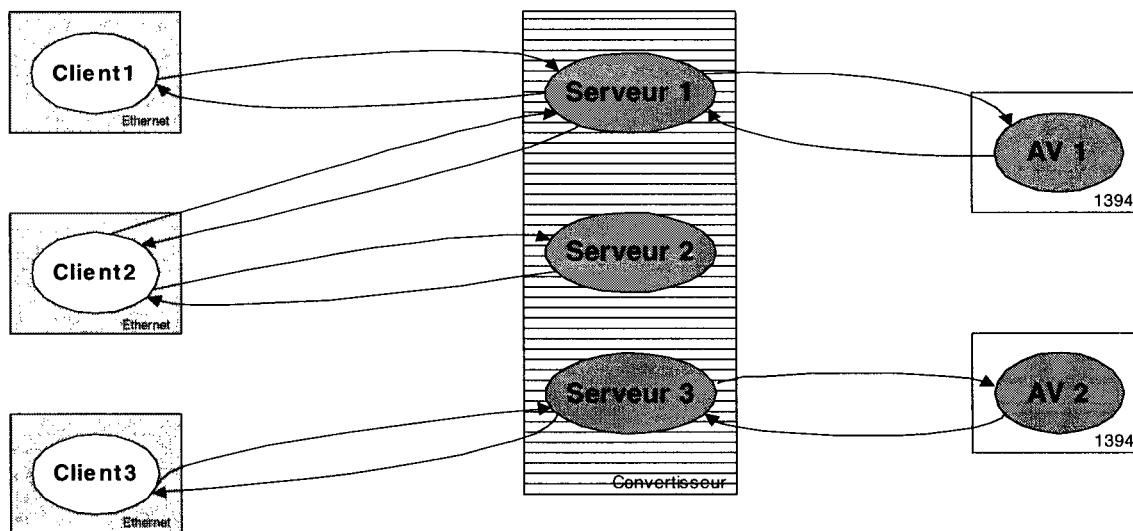
Figure 4-9. Architecture du système pour le transport de données AV
