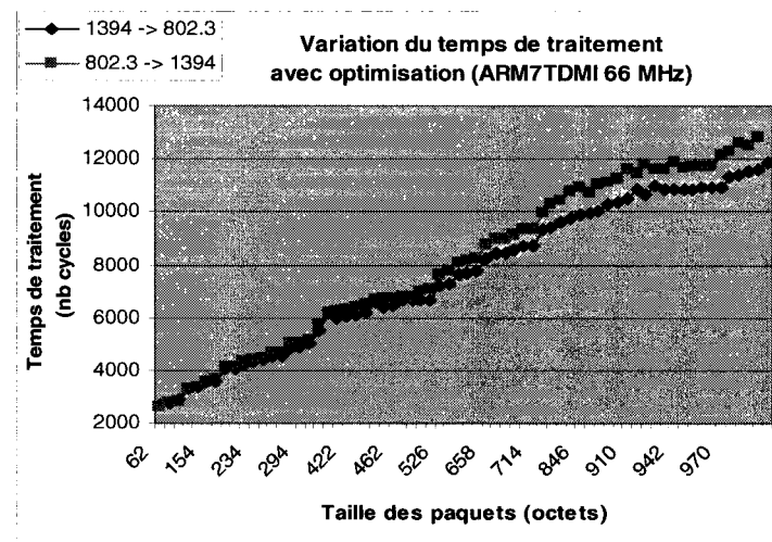
Figure 3-14. Temps de traitement de la solution optimisée
