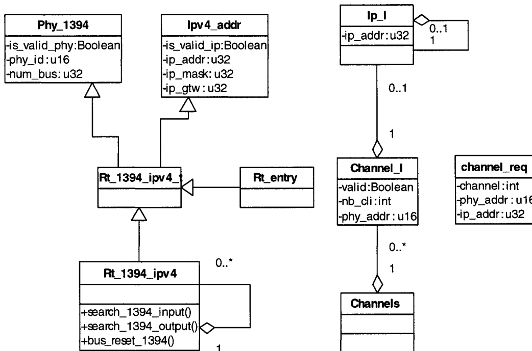
Figure E-6. Diagramme de structures du module de routage FireoverIP
