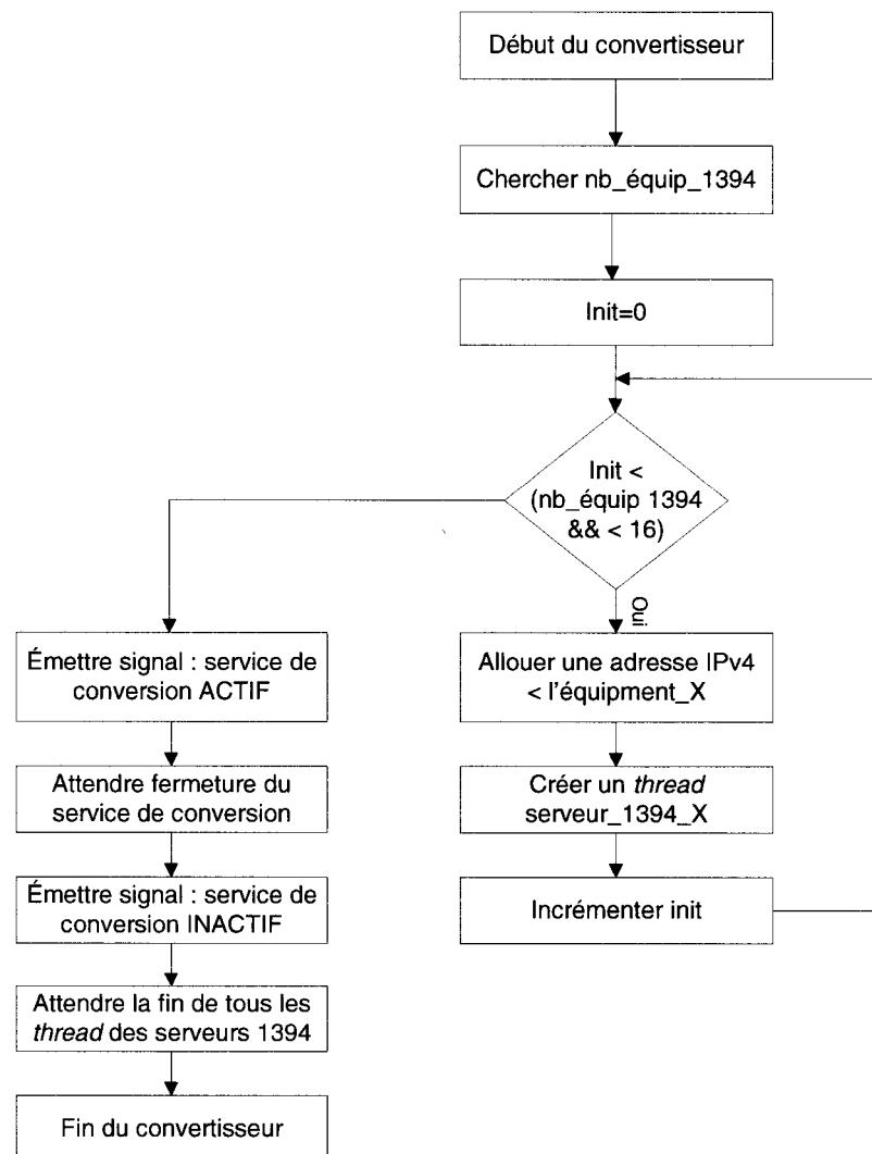
Figure 4-10. Organigramme de la passerelle
