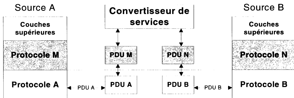
Figure 2-2. Cas d'une conversion de services
