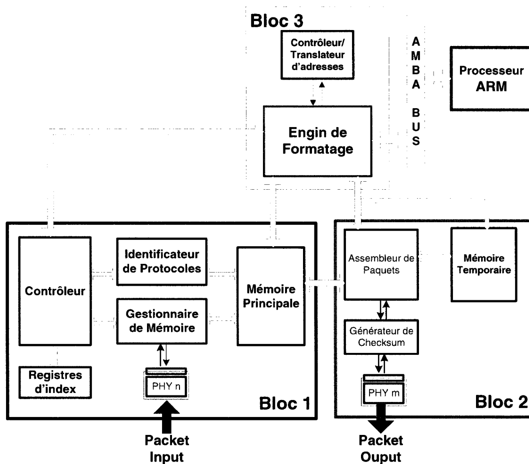
Figure 3-17. Architecture d'une plate-forme SOC pour la conversion de protocoles
