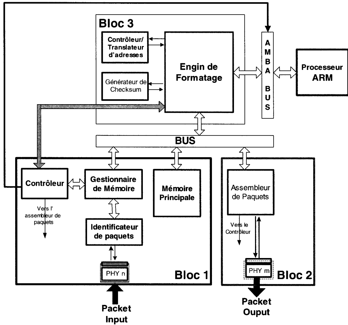
Figure 3-21. Proposition d'une nouvelle architecture pour la conversion de protocoles
