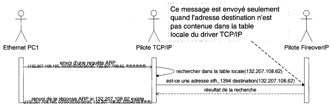
Figure E-4. Séquence d'opérations après la réception d'une requête ARP **caractères trop petits dans les échanges de gauche **
