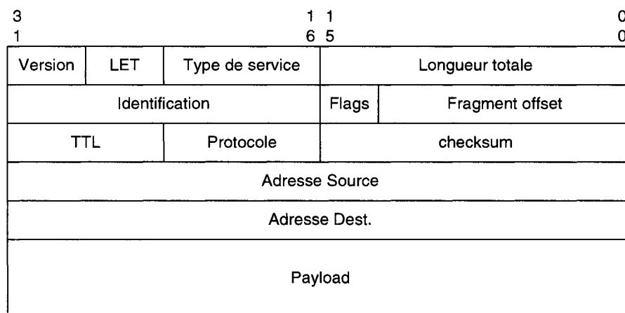
Figure B-1. Format de l'entête d'un paquet IP
