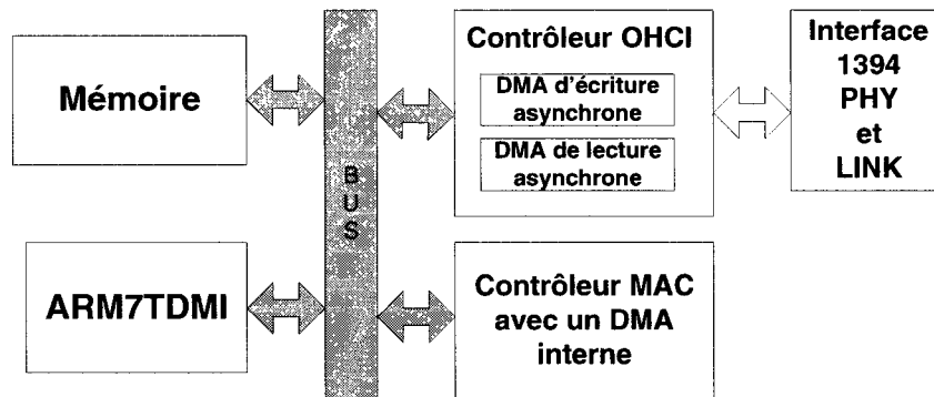
Figure 3-15. Architecture de la solution logicielle
