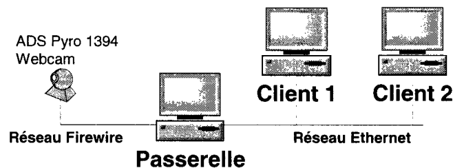
Figure 4-11. Environnement de test de la passerelle
