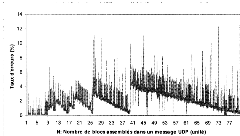
Figure 4-17. Variation du pourcentage d'octets perdus
