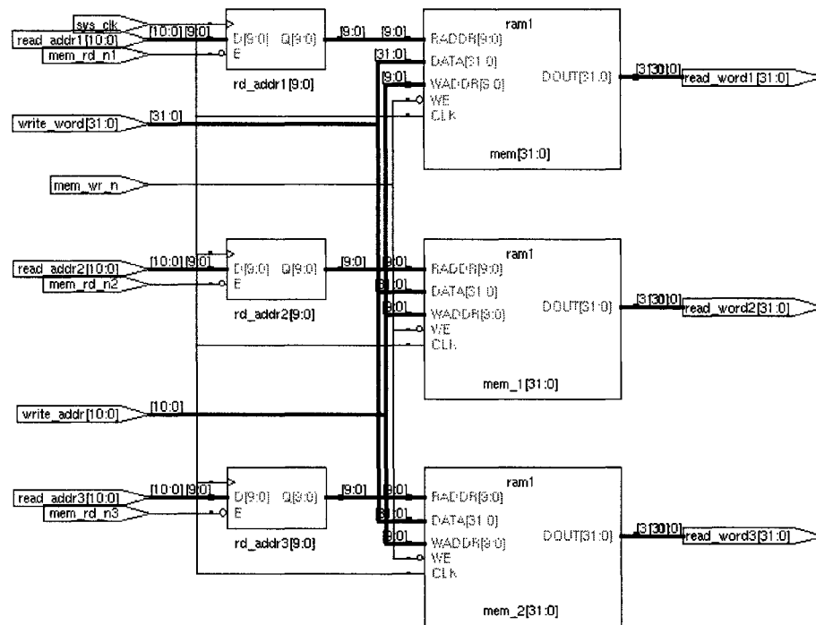
Figure 3-18. Mémoire principale générée par Synplify
