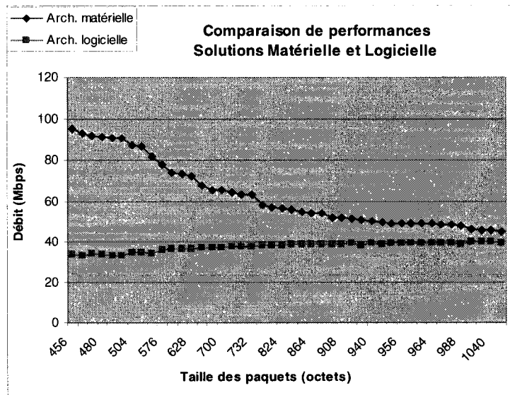
Figure 3-20. Variation du débit de l'architecture matérielle
