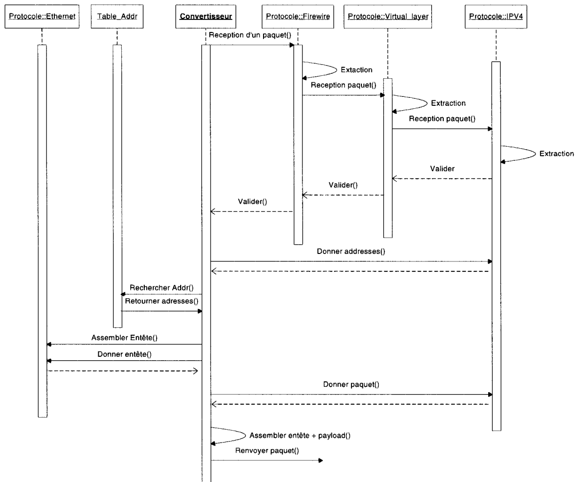
Figure 3-10. Diagramme de séquence de la conversion Firewire / Ethernet
