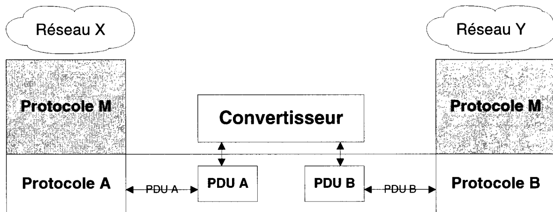
Figure 2-5. Cas d'une conversion de protocoles
