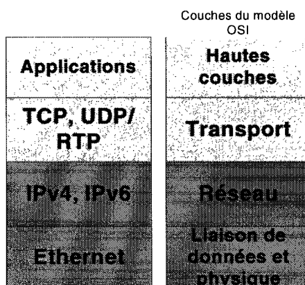
Figure 2-9. Empilements de protocoles au-dessus de Ethernet
