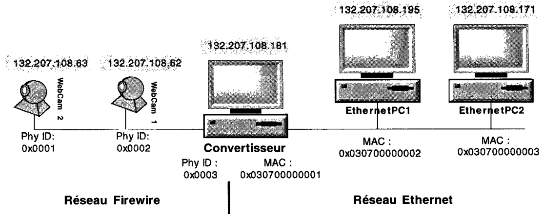
Figure E-3. État des réseaux après l'étape d'initialisation
