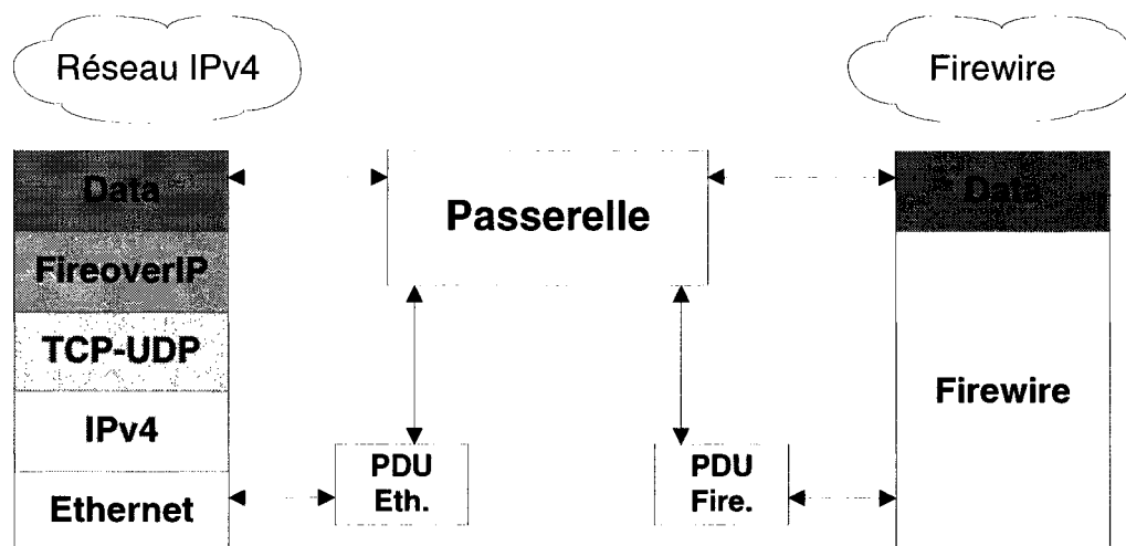
Figure 4-7. Protocoles présents durant l'interconnexion de LAN TCP/IP et Firewire
