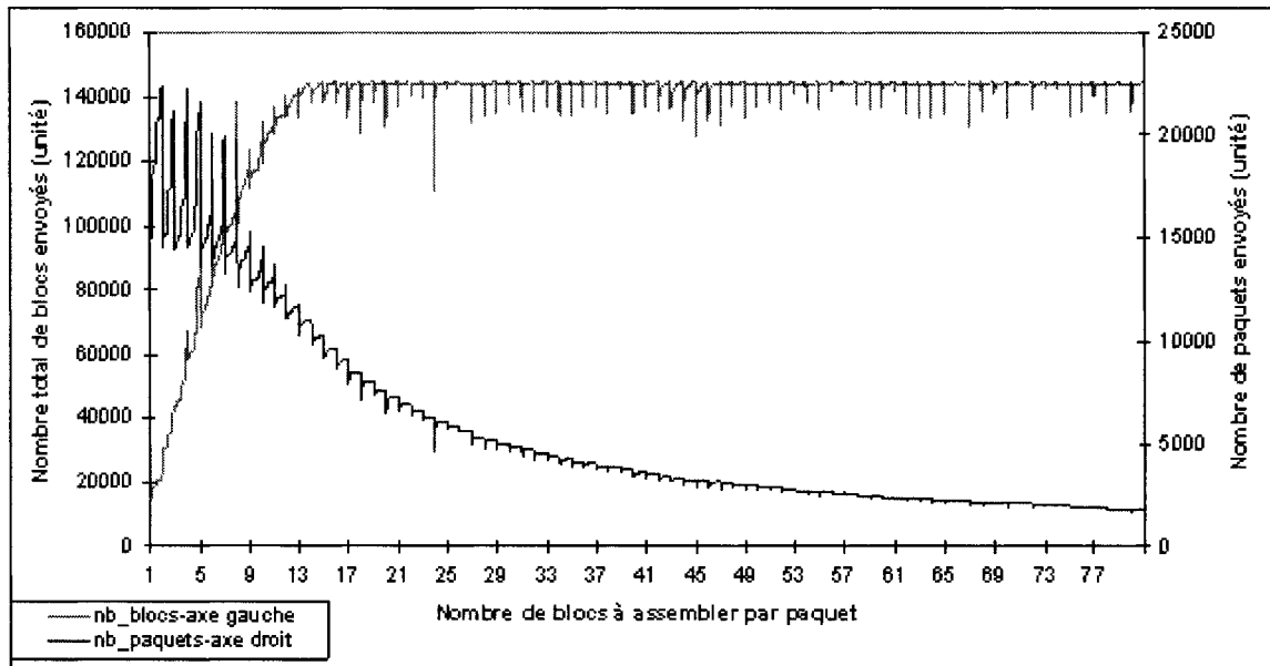
Figure 4-13. Variation du nombre de paquets envoyés pour un taux de 15 images/s
