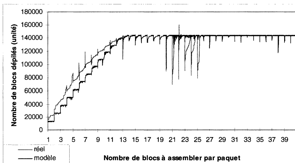
Figure I-2. Variation du nombre des blocs dépilés pour un taux de 30 im/s
