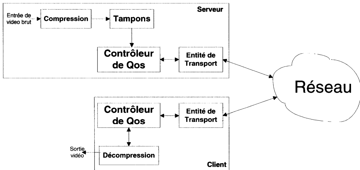
Figure 2-10. Architecture générale d'un système d'envoi de flots vidéo
