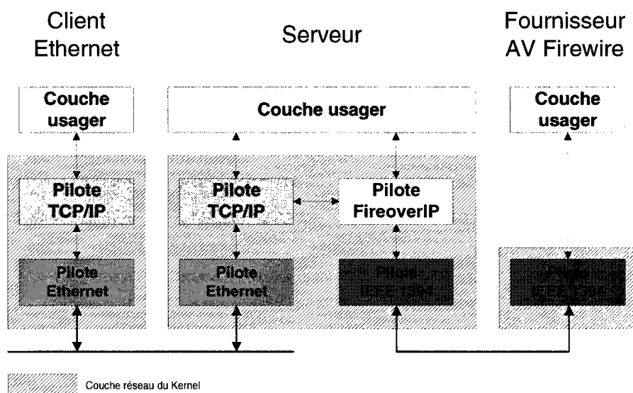
Figure 4-4. Place de la passerelle dans l'architecture d'un système d'exploitation
