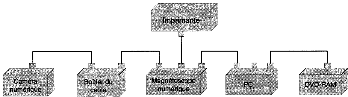
Figure 2-6. Topologie d'un réseau Firewire
