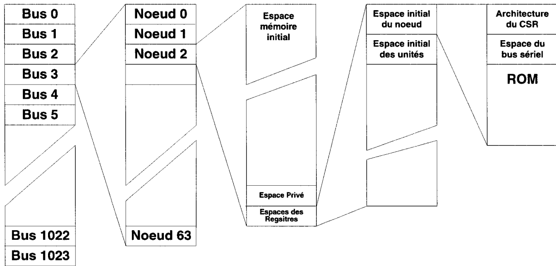
Figure 2-7. Système d'adressage de Firewire ( IEEE Std 1394-1995, 1995 )
