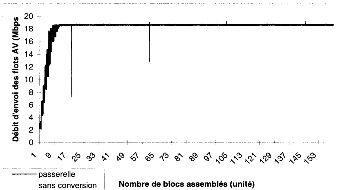
Figure H-3. Variation de la vitesse moyenne d'envoi des flots AV pour 7.5 im/s
