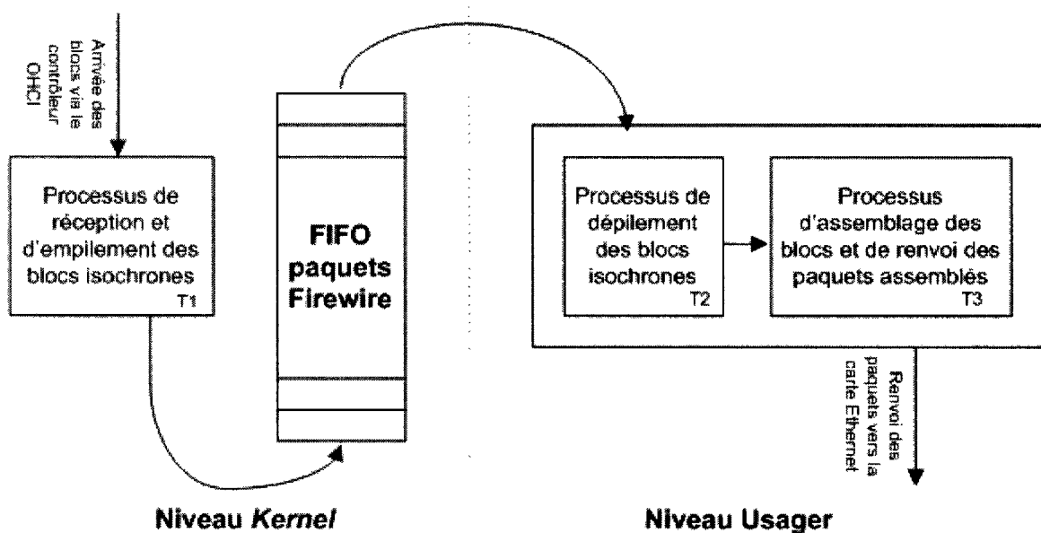
Figure 4-12. Processus de traitements des blocs isochrones
