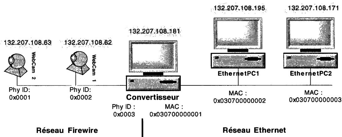
Figure 4-5. État des réseaux après l'étape d'initialisation
