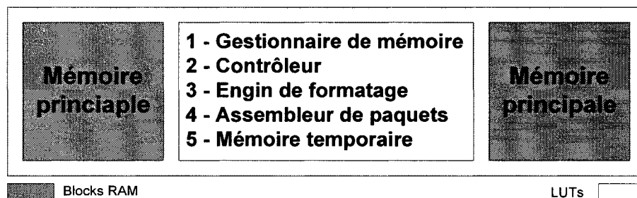
Figure 3-19. Placement des modules dans le FPGA Xilinx Virtex XCV1000
