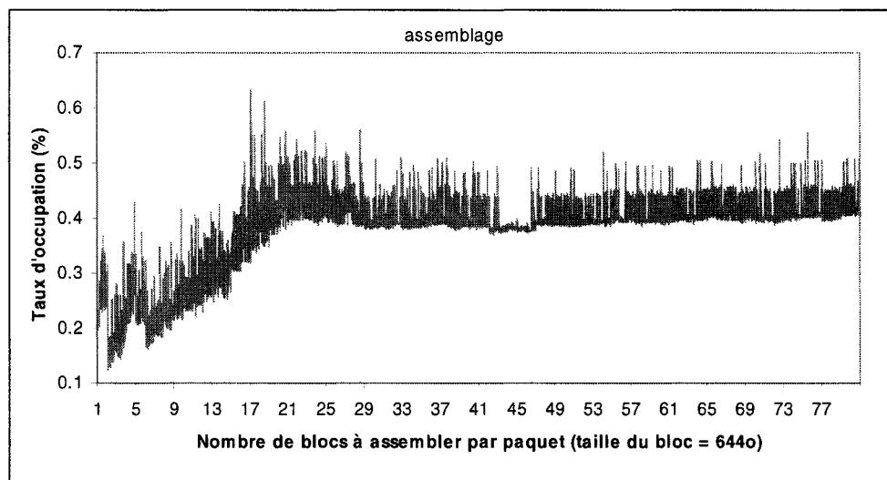
Figure 4-15. Variation de l'occupation du temps d'assemblage
