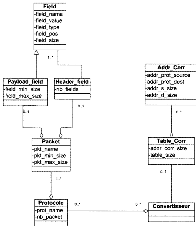
Figure 3-9. Diagramme de classes du convertisseur semi-générique
