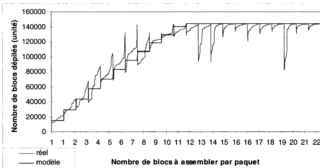
Figure I-1. Variation du nombre des blocs dépilés pour un taux de 7.5 im/s
