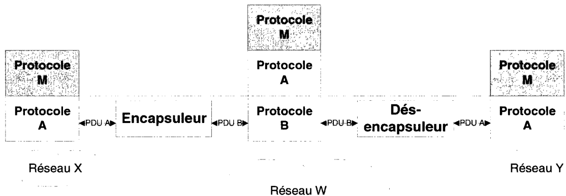
Figure 2-3. Cas d'une encapsulation de protocoles
