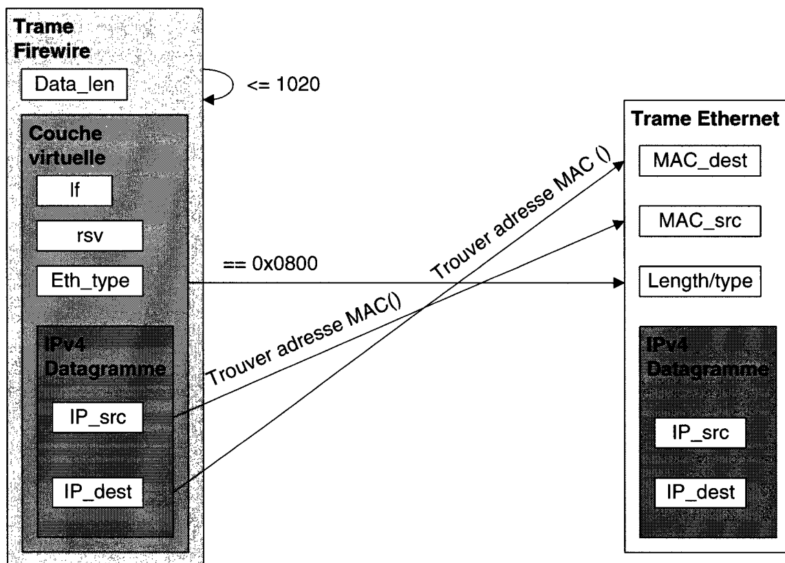
Figure 3-12. Correspondances entre les champs
