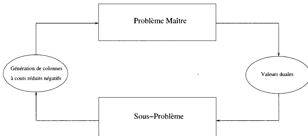
Figure 2.1: Une itération de la technique de génération de colonnes
