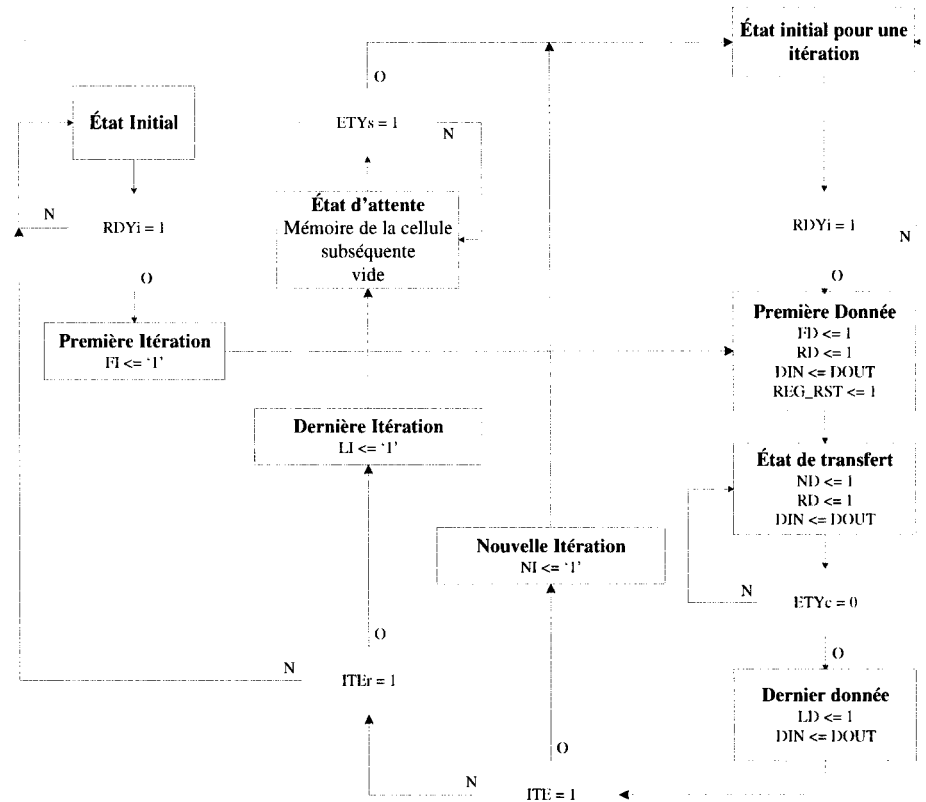
Figure 5.5 – Diagramme d'état du contrôleur de la cellule itérative.
