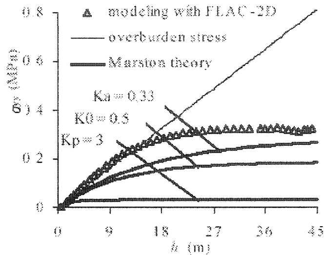
Figure 6.2. Comparaison de l'effet d'arche obtenu par simulations numériques à l'aide de l'approche analytique de Martson (d'après Li et al. 2003).
