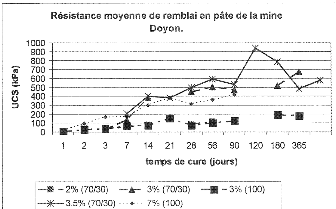
Figure 2.6. Évolution comparative des cinq recettes de remblai de la mine Doyon.
