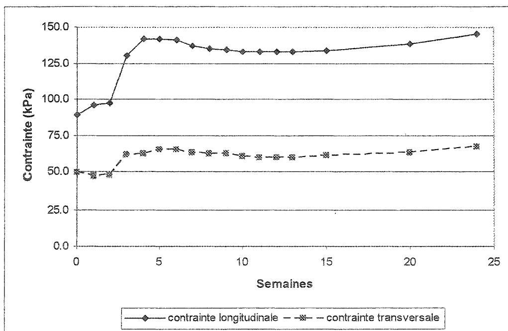
Figure 5.2. Variation à moyen terme des contraintes au plancher du petit chantier après la fin du remblayage
