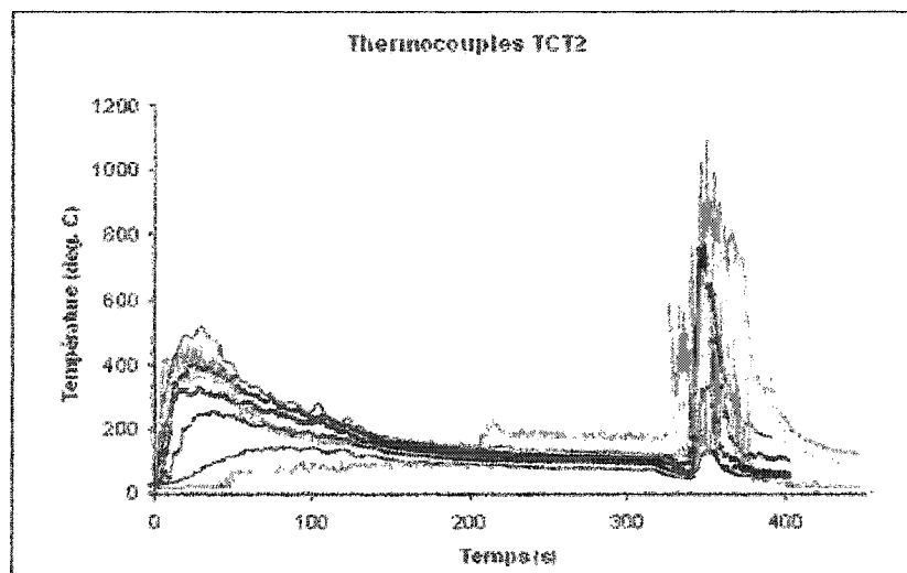
Figure 5.12 : Comparaison des températures pour le maillage grossier (avec fuites)
