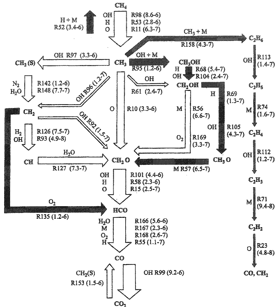
Figure 6.1 : Diagramme du cheminement de la réaction de combustion du méthane à basse température ( <1500\text{K} )
