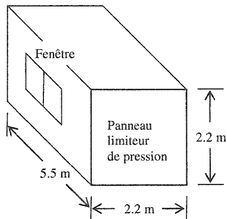
Figure 4.1 : Dimensions du conteneur utilisé
