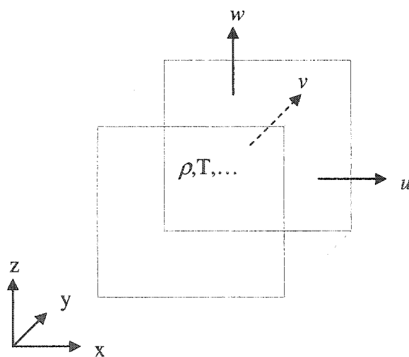
Figure 2.5 : Volume de contrôle et assignation des variables
