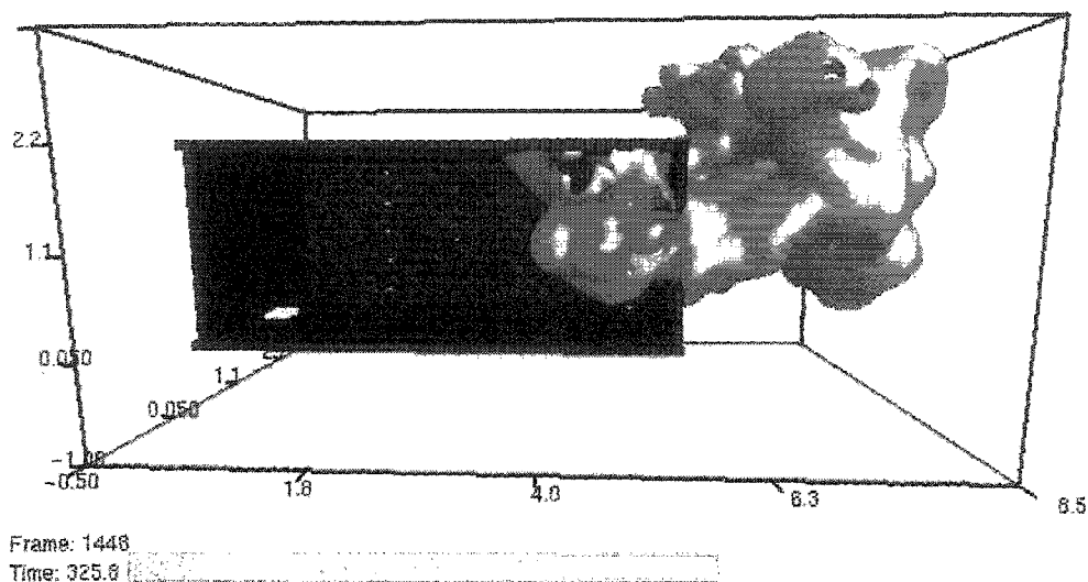
Figure 5.10 : Surface estimée de la flamme à 325,8 secondes (sans fuites)
