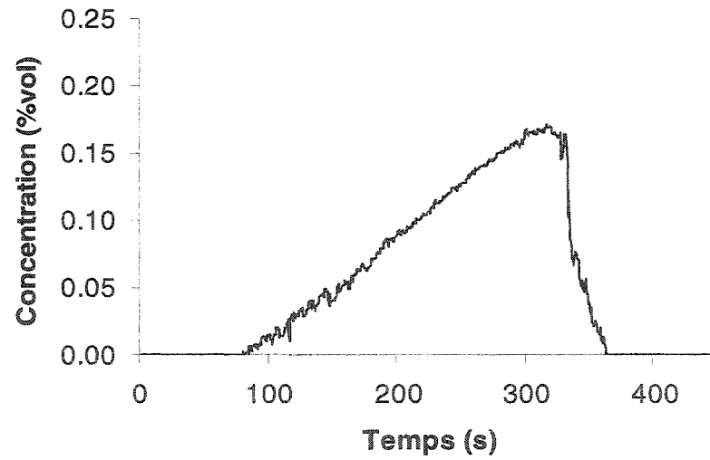
Figure 6.14 : Valeurs simulées de la concentration en méthane (simulation C-4)
