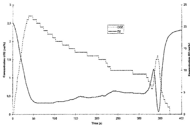
Figure 5.3 : Mesures expérimentales des concentrations
