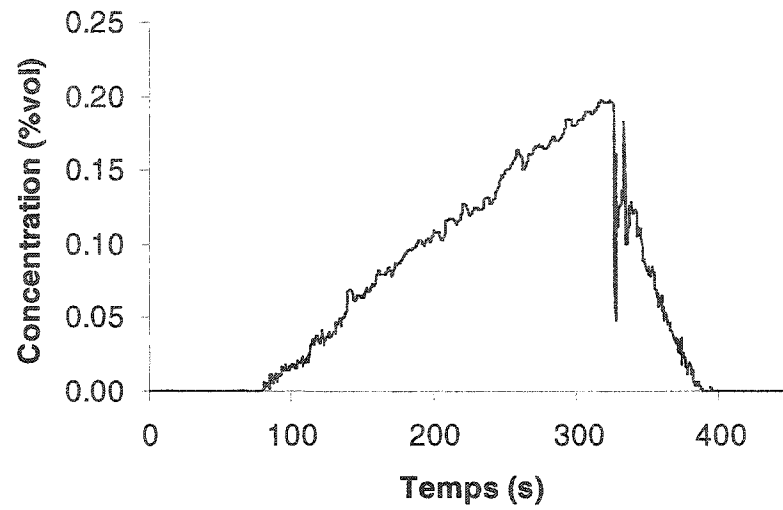
Figure 6.13 : Valeurs simulées de la concentration en méthane (simulation C-3)
