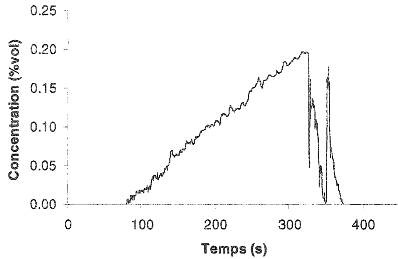
Figure 6.11 : Valeurs simulées de la concentration en méthane (simulation C-1)
