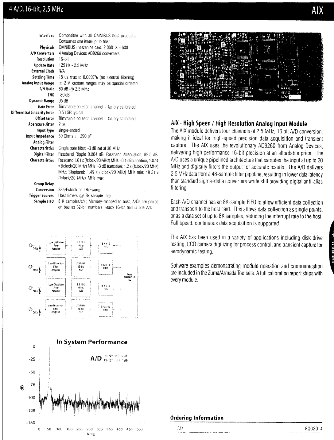
Figure A6.1 : Fiche descriptive de la carte d'acquisition de données (innovative Integration, 2003)
