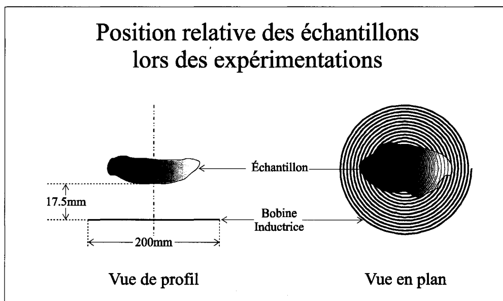
Figure 3.11: Représentation de la position relative des échantillons lors des expérimentations. L'échantillon est centré avec l'axe de la bobine.
