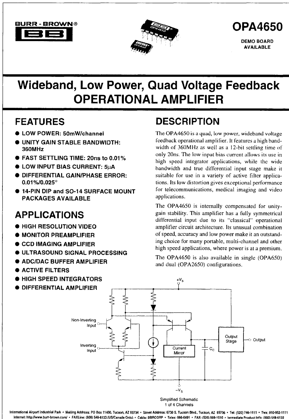
Figure A9.2 : Fiche descriptive de l'amplificateur différentiel utilisé. Première page du feuillet de 13 pages servant d'aide technique (Texas Instruments, 2003)
