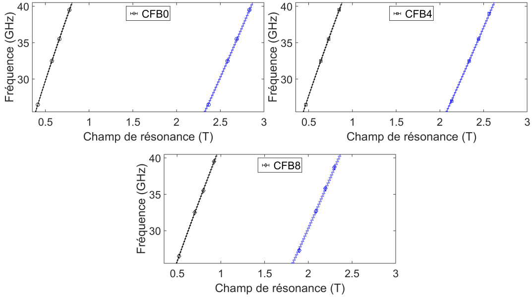
FIGURE 4.10 Résultats des régressions sur la condition de résonance à température ambiante pour l'orientation parallèle (noir) et perpendiculaire (bleu) qui prend en compte l'angle du champ externe.
