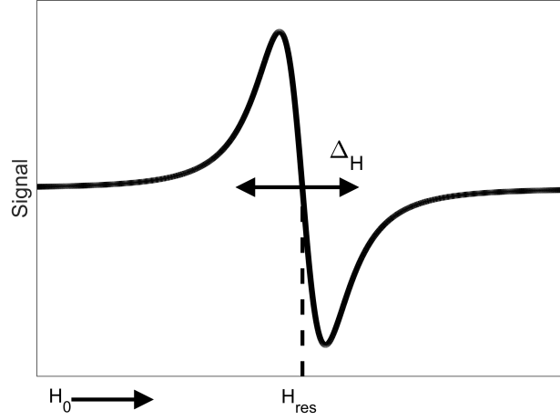
FIGURE 2.2 Schéma d'un signal typique de résonance ferromagnétique.
