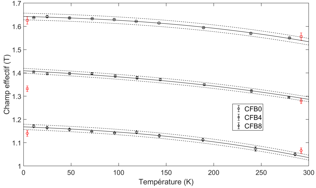
FIGURE 4.21 Résultats des régressions non linéaires sur le champ effectif interne en fonction de la température en considérant l'aimantation à saturation comme une loi de puissance et la constante d'anisotropie de surface comme une droite pour les 3 échantillons.
