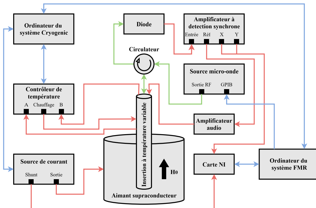
FIGURE 3.2 Schéma du montage complet où les instruments, les composants RF et les connexions sont représentés. Les connexions sont séparés en trois catégories, soit les câbles coaxiaux 2.92 mm acheminant les micro-ondes (vert), les câbles coaxiaux BNC acheminant des voltages continus ou à très basse fréquence (rouge) et les câbles de communication acheminant les commandes (bleu).
