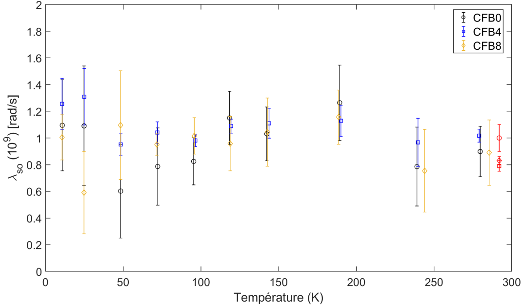
FIGURE 4.22 Taux de relaxation magnétique en fonction de la température pour les 3 échantillons.
