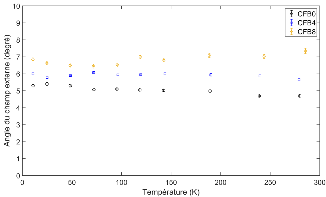
FIGURE 4.14 Angle entre le champ externe et la normale de la couche mince en fonction de la température lors des mesures perpendiculaires pour les 3 échantillons.
