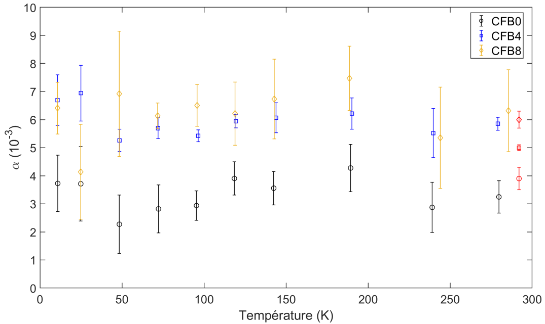
FIGURE 4.15 Constante de Gilbert en fonction de la température pour les 3 échantillons.
