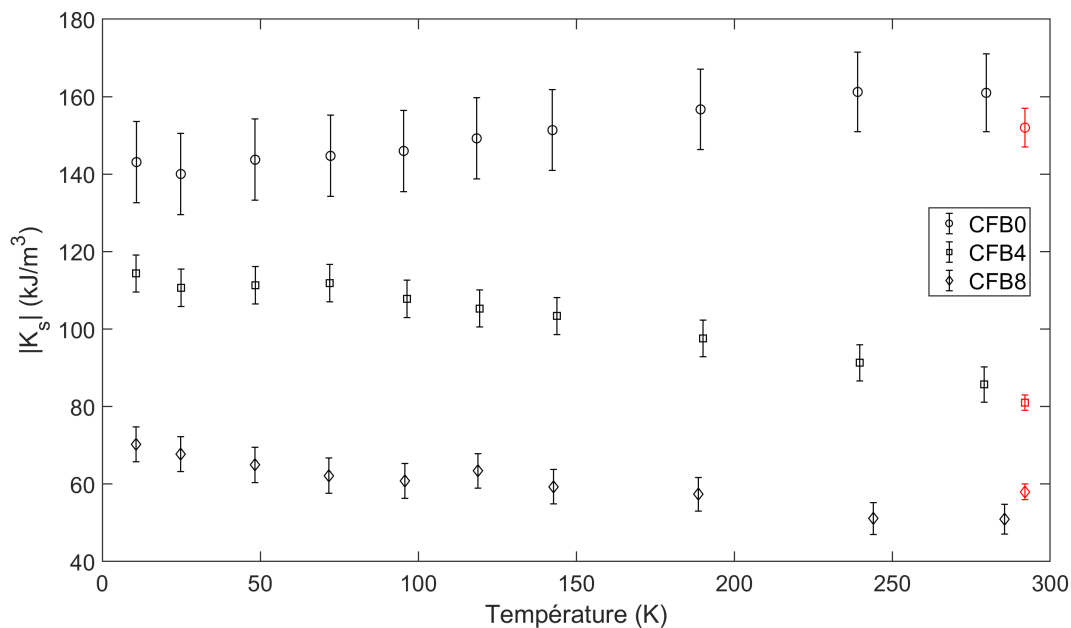
FIGURE 4.20 Constante d'anisotropie de surface en fonction de la température pour les 3 échantillons.
