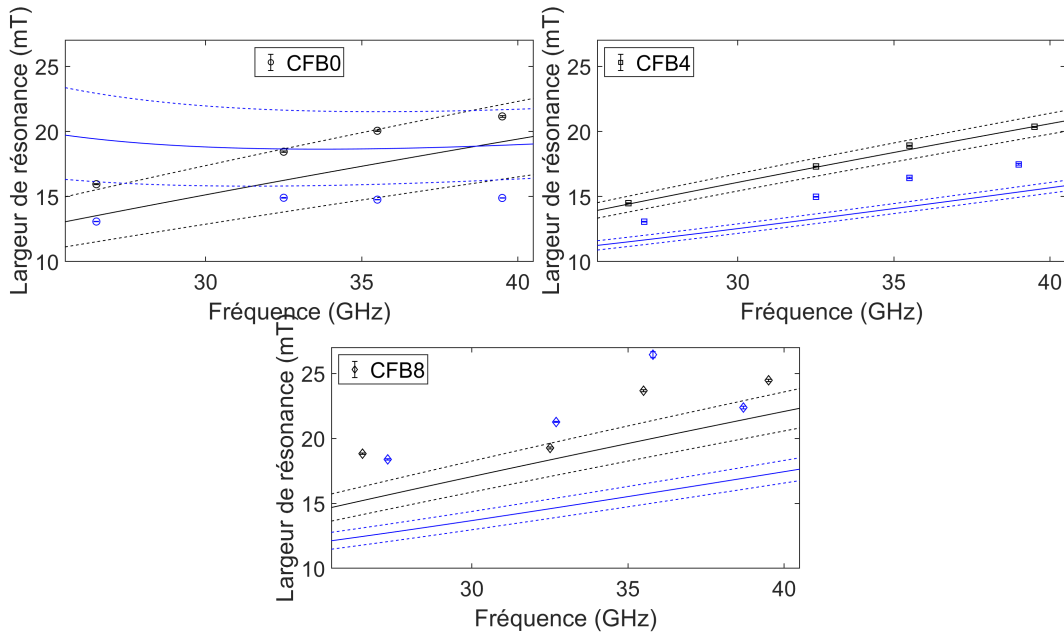
FIGURE 4.11 Comparaison entre les largeurs de résonance mesurées en fonction de la fréquence (points) et celles prédites par les paramètres de l'article de C. Lacroix (courbes) à température ambiante pour l'orientation parallèle (noir) et perpendiculaire (bleu) [5].
