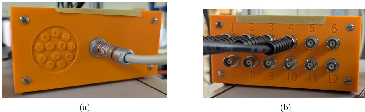
FIGURE 3.6 (a) Premier côté de la boîte de transfert avec le connecteur à 12 broches Fischer où le numéro des broches est indiqué. (b) Deuxième côté de la boîte de transfert avec les 12 connecteurs BNC où le numéro de la broche correspondante est indiqué.
