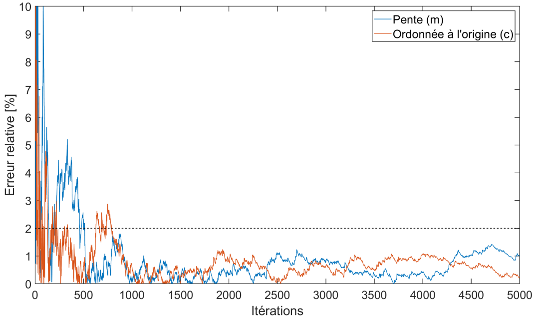
FIGURE B.1 L'erreur relative de l'incertitude de la pente et de l'ordonnée à l'origine en fonction du nombre d'itérations Monte Carlo.
