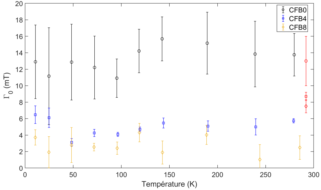
FIGURE 4.16 Constante de D2M en fonction de la température pour les 3 échantillons.
