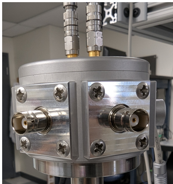
FIGURE 3.11 Les connecteurs hermétiques BNC permettant d'alimenter la bobine ainsi que les plaques d'aluminium permettant de les installer à l'interface de l'insertion.
