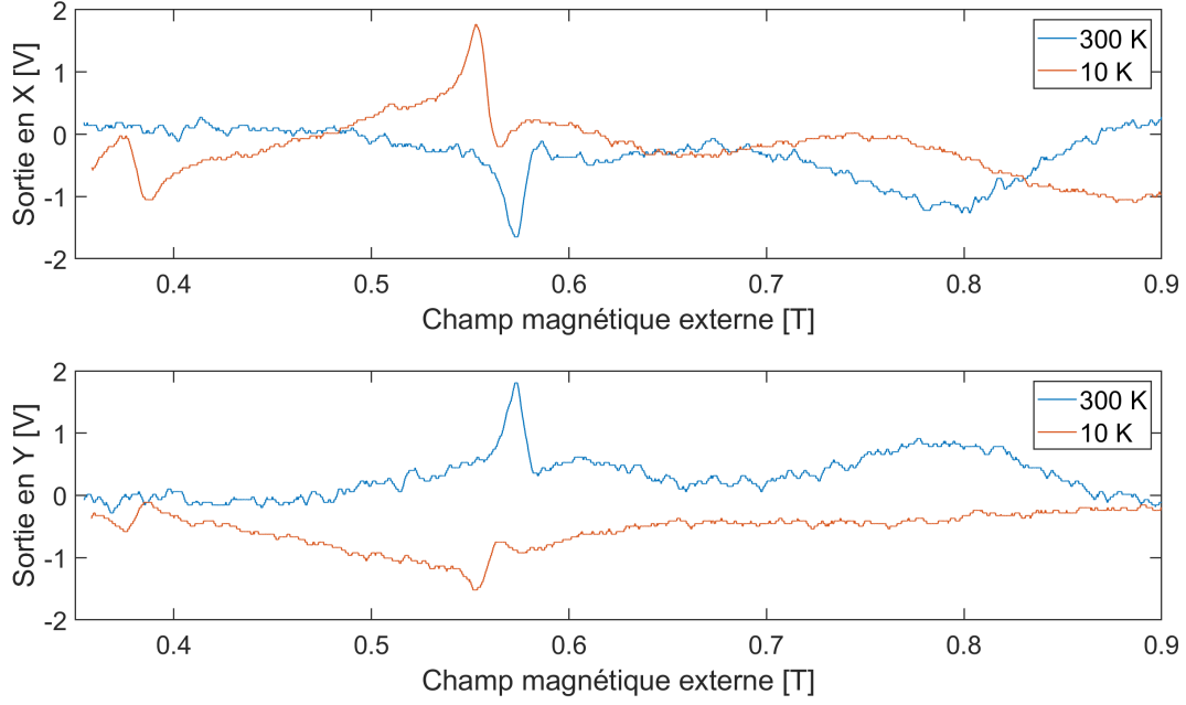
FIGURE 4.1 Exemple de signaux de sortie du LIA bruts en fonction du champ magnétique externe pour deux températures pour l'échantillon CFB0 à 32.5 GHz avec le champ magnétique parallèle à la couche mince.
