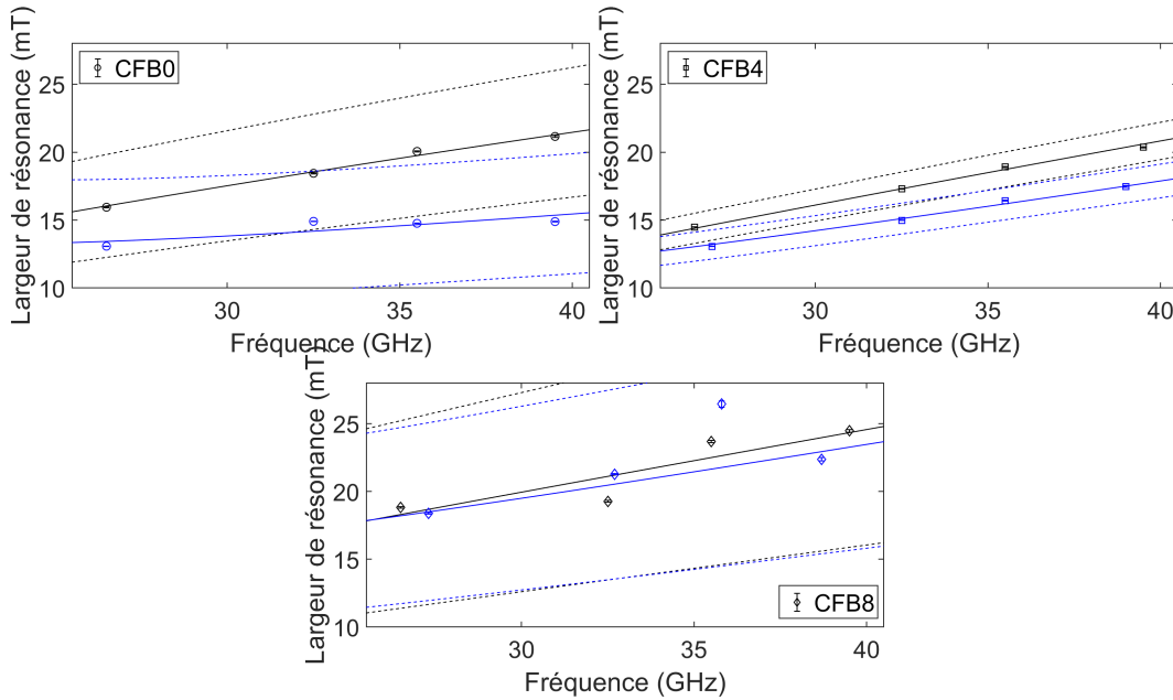
FIGURE 4.12 Résultats des régressions sur les largeurs de résonance en fonction de la fréquence à température ambiante pour l'orientation parallèle (noir) et perpendiculaire (bleu).
