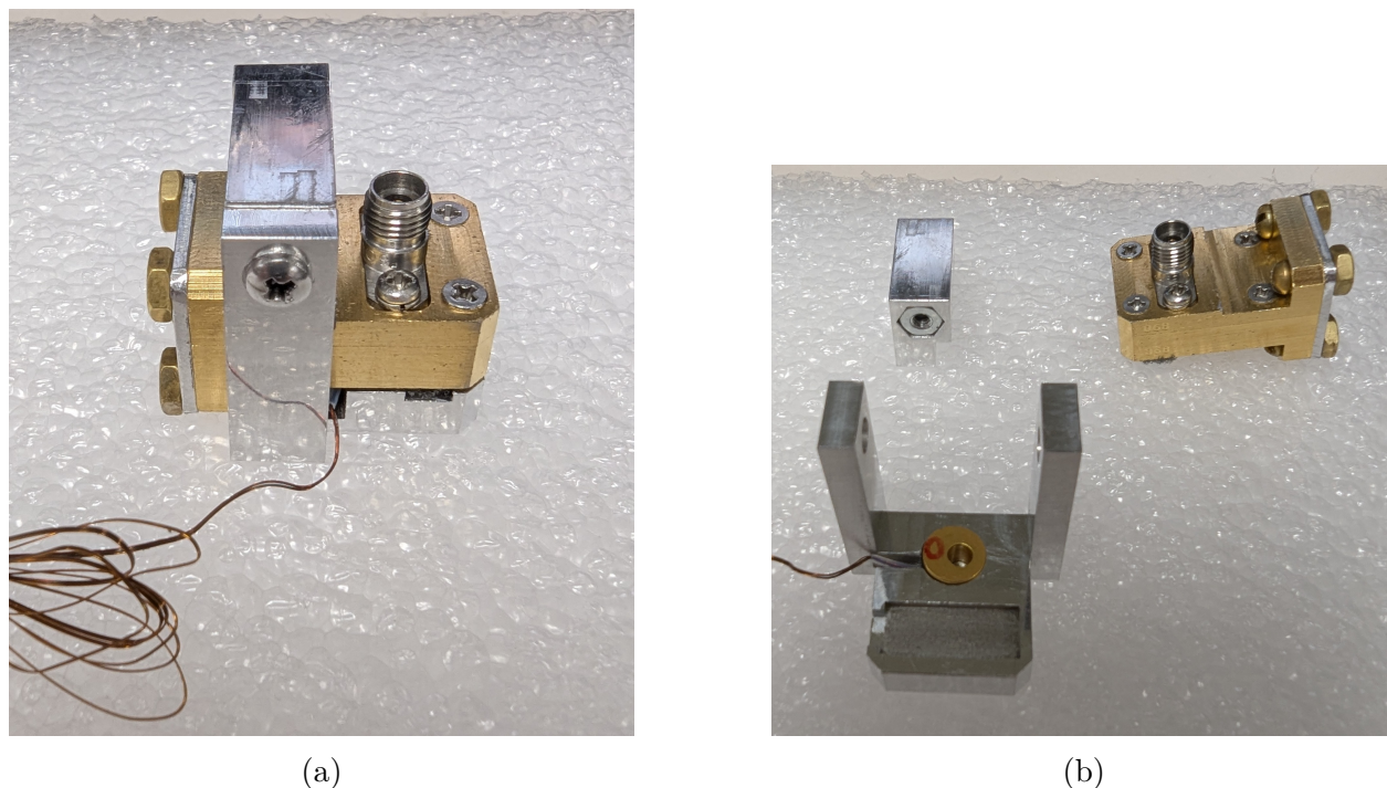
FIGURE 3.5 (a) Le support de capteur de température installé sur l'adaptateur avec les fils d'alimentation et de mesure du capteur Cernox sortant du côté. (b) Les mêmes composantes désinstallées afin d'observer l'emplacement du capteur de température Cernox .
