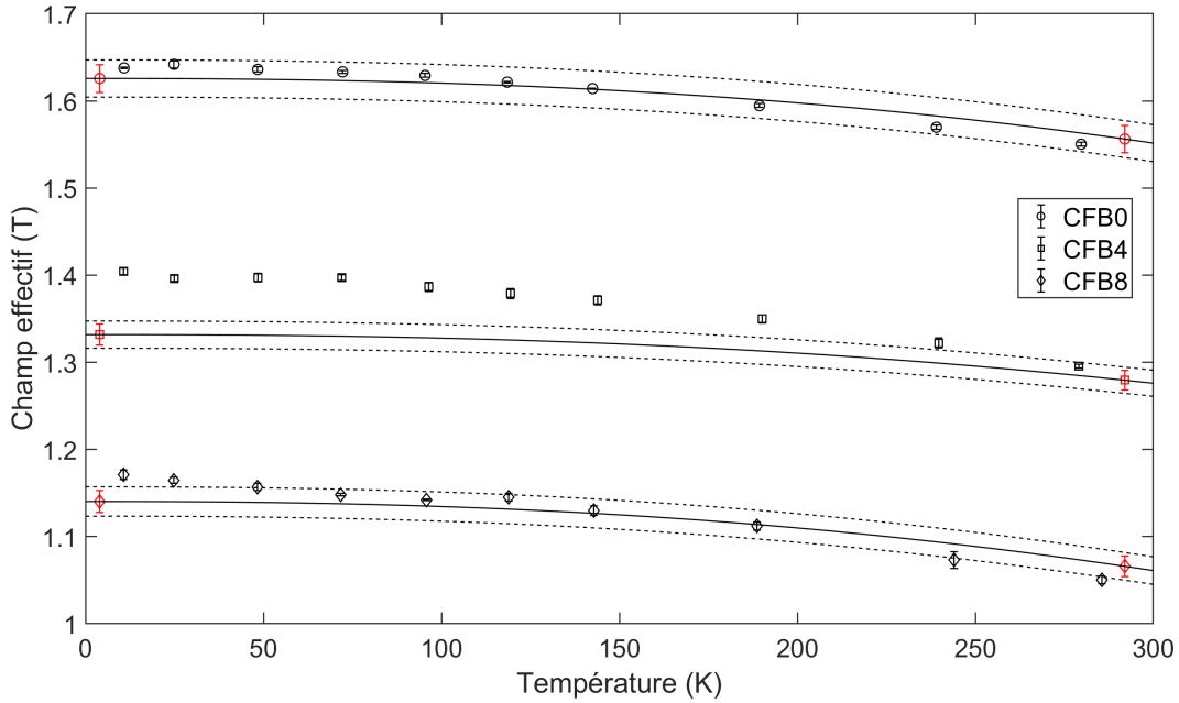
FIGURE 4.19 Comparaison entre les points expérimentaux de champ effectif interne et les courbes de champ effectif interne prédites par les lois de puissance d'aimantation à saturation en fonction de la température pour les 3 échantillons.
