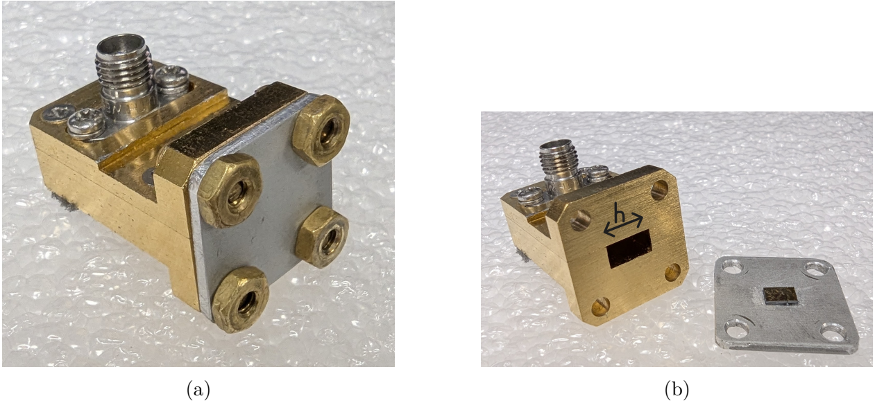
FIGURE 3.7 (a) L'adaptateur coaxial-guide d'onde avec la plaque d'aluminium installée au bout de la partie guide d'onde. (b) Les mêmes composantes désinstallées afin d'observer l'échantillon installé sur la face intérieur de la plaque d'aluminium. L'orientation du champ magnétique alternatif micro-onde \mathbf{h} est aussi représenté.
