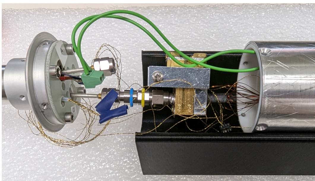
FIGURE 3.9 La disposition de l'adaptateur, du support de capteur de température et du câble coaxial à l'intérieur du cylindre allant au fond de l'insertion au cœur de l'aimant pour l'orientation du champ magnétique continu parallèle à la couche mince.
