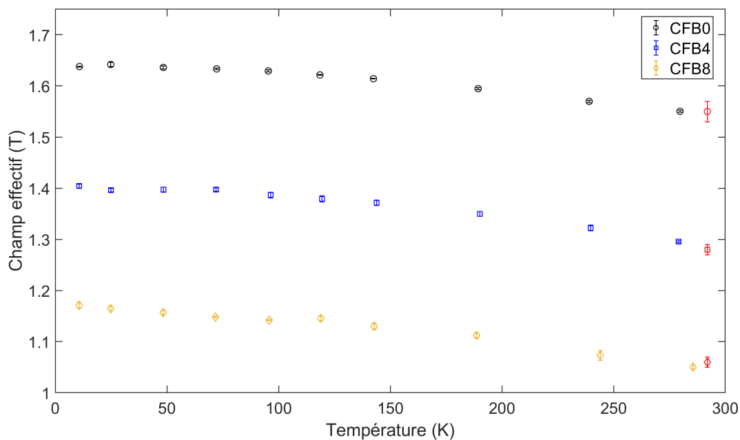
FIGURE 4.13 Champ effectif interne en fonction de la température pour les 3 échantillons.
