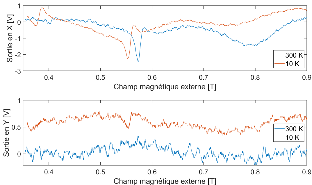
FIGURE 4.2 Exemple de signaux de sortie du LIA combinés en fonction du champ magnétique externe pour deux températures pour l'échantillon CFB0 à 32.5 GHz avec le champ magnétique parallèle à la couche mince.
