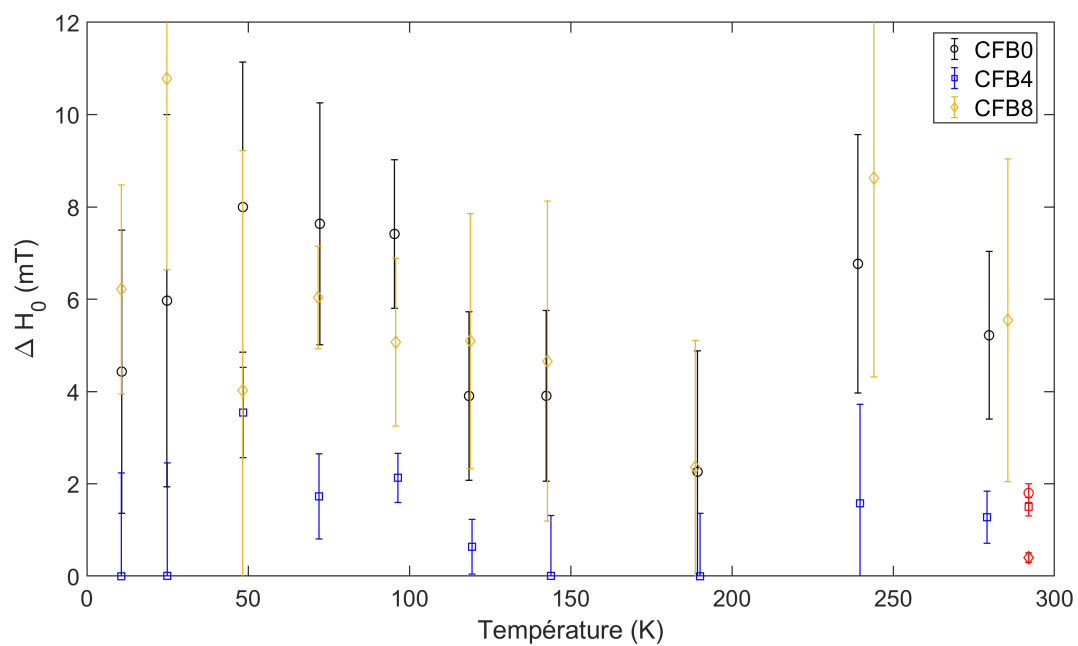
FIGURE 4.18 Largeur de résonance autre en fonction de la température pour les 3 échantillons.
