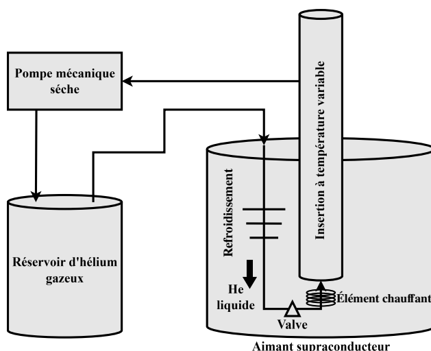
FIGURE 3.4 Schéma simplifié du circuit en boucle fermée d'hélium refroidi servant à contrôler la température de l'insertion où la valve, l'élément chauffant, la pompe et le réservoir sont montrés.
