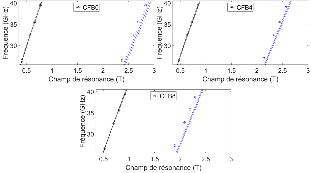
FIGURE 4.9 Comparaison entre les fréquences en fonction des champs de résonance (points) et les conditions de résonance prédites par les paramètres de l'article de C. Lacroix (courbes) à température ambiante pour l'orientation parallèle (noir) et perpendiculaire (bleu) [5].
