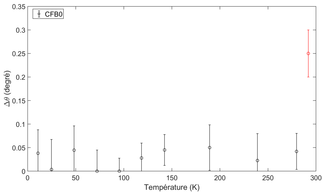
FIGURE 4.17 Constante de variation du champ interne en fonction de la température pour l'échantillon CFB0.
