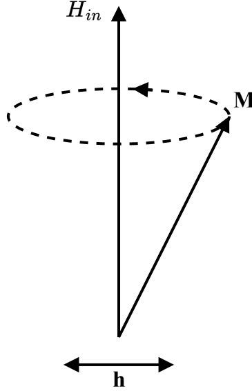
FIGURE 2.1 Précession forcée.
