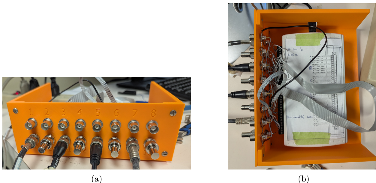
FIGURE 3.12 (a) La face de la boîte de transfert avec les 16 connecteurs BNC et leur numéro d'identification. (b) L'intérieur de la boîte de transfert avec la carte d'acquisition et la feuille indiquant la correspondance entre les broches et les connecteurs BNC.
