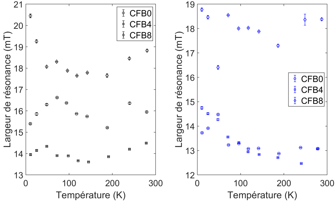
FIGURE 4.8 La largeur de résonance en fonction de la température pour les 3 échantillons et les deux orientations, soit lorsque le champ externe est parallèle (noir) et perpendiculaire (bleu) à la couche mince.
