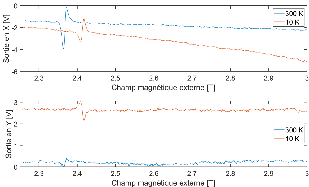
FIGURE 4.3 Exemple de signaux de sortie du LIA combinés en fonction du champ magnétique externe pour deux températures pour l'échantillon CFB0 à 26.5 GHz avec le champ magnétique perpendiculaire à la couche mince.
