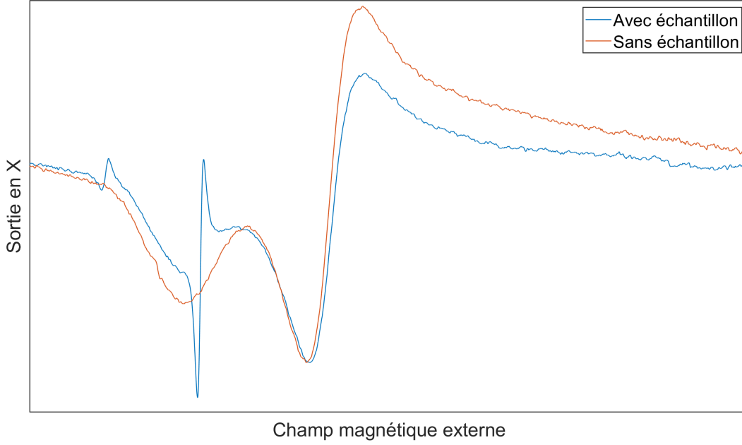
FIGURE 4.4 Comparaison entre une mesure avec et sans l'échantillon à l'intérieur de l'adaptateur.
