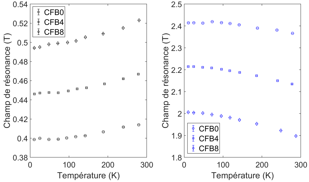
FIGURE 4.7 Le champ de résonance en fonction de la température pour les 3 échantillons et les deux orientations, soit lorsque le champ externe est parallèle (noir) et perpendiculaire (bleu) à la couche mince.
