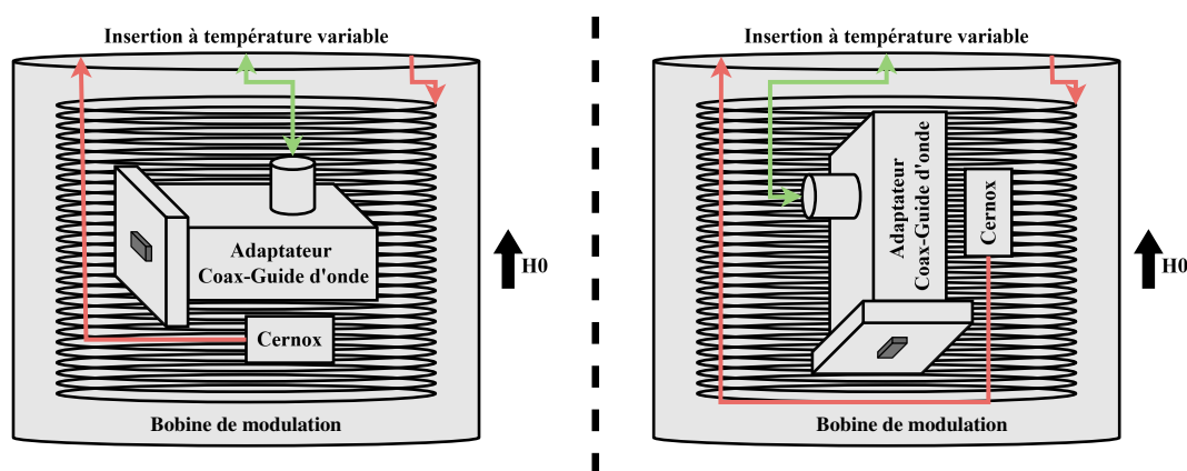
FIGURE 3.3 Schéma de l'intérieur de l'insertion à température variable où l'adaptateur, la bobine de modulation, le capteur de température Cernox et l'échantillon sont représentés. Les connections sont aussi représentées et utilisent la même convention de couleurs que dans la figure 3.2. Les deux orientations de l'échantillon sont représentées, soit lorsque le champ externe est parallèle à l'échantillon (gauche) et lorsque le champ externe est perpendiculaire à l'échantillon (droite).
