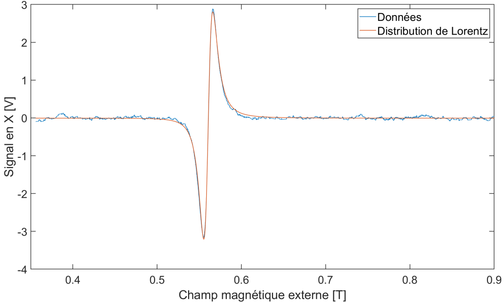
FIGURE 4.6 Résultat de la régression non linéaire sur le pic de résonance de l'échantillon CFB0 à 32.5 GHz et à 125 K avec le champ magnétique parallèle à la couche mince.
