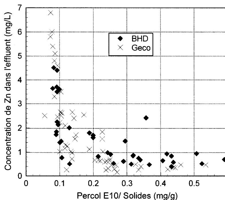
Figure 4.2 : Relation entre le dosage de Percol E10 et la concentration de Zn de l'effluent
