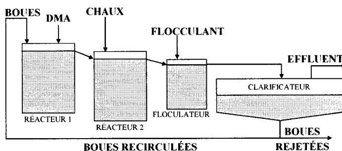
Figure 3.8 : Schéma du procédé Geco modifié tel qu'appliqué au test 7
