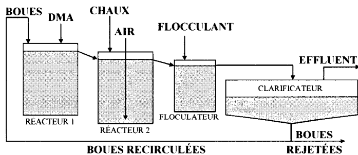
Figure 3.6 : Schéma du procédé Geco tel qu'appliqué lors des tests 4B, 4C, et 4D
