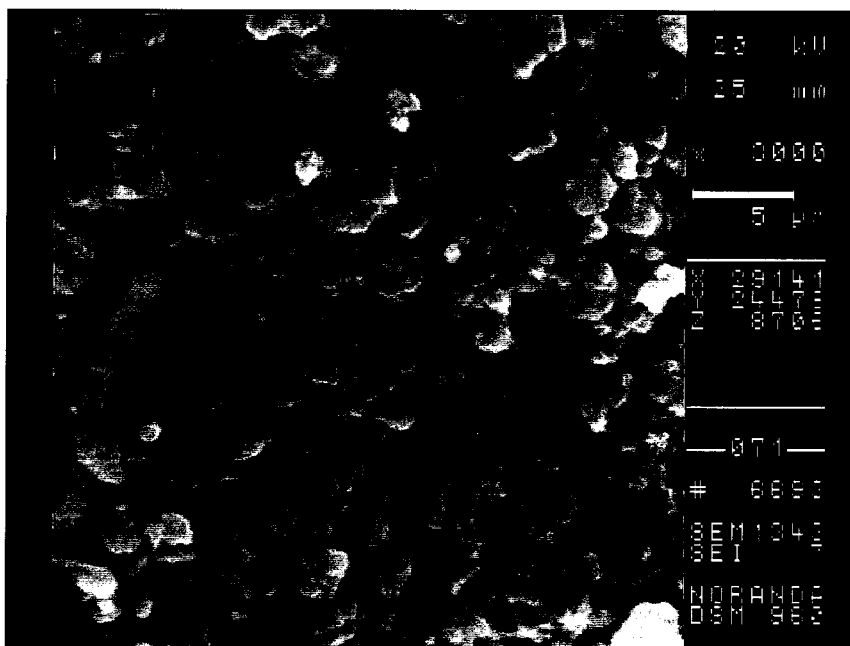
Figure 4.8 : Photo MEB des boues du test 7 avec une magnification de 3 000 fois (Geco - 21% solides)
