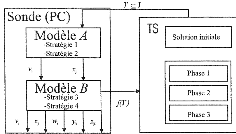
Figure 3.4: Combinaison de la recherche locale et du modèle de PC
