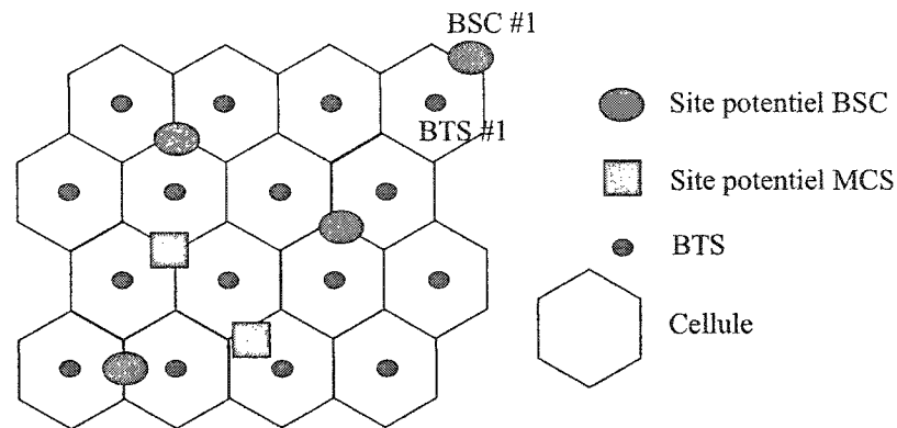
Figure 1.2: Exemple d'un réseau cellulaire typique
