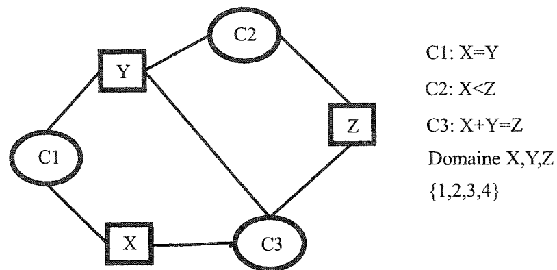
Figure 2.2: Réseau de contraintes
