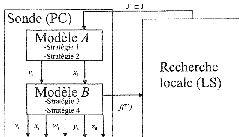
Figure 3.2: Combinaison de la recherche locale et du modèle de PC
