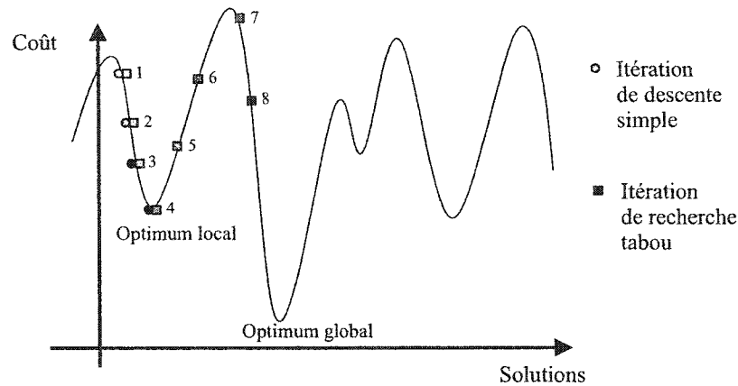
Figure 2.3: Recherche locale à descente simple vs recherche tabou
