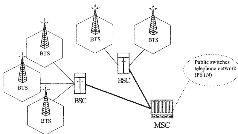
Figure 1.1: Relation entre les composantes d'un réseau cellulaire
