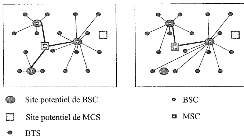
Figure 3.3: Mouvement de la recherche locale : le site de BSC le plus faiblement connecté est enlevé de solution courante
