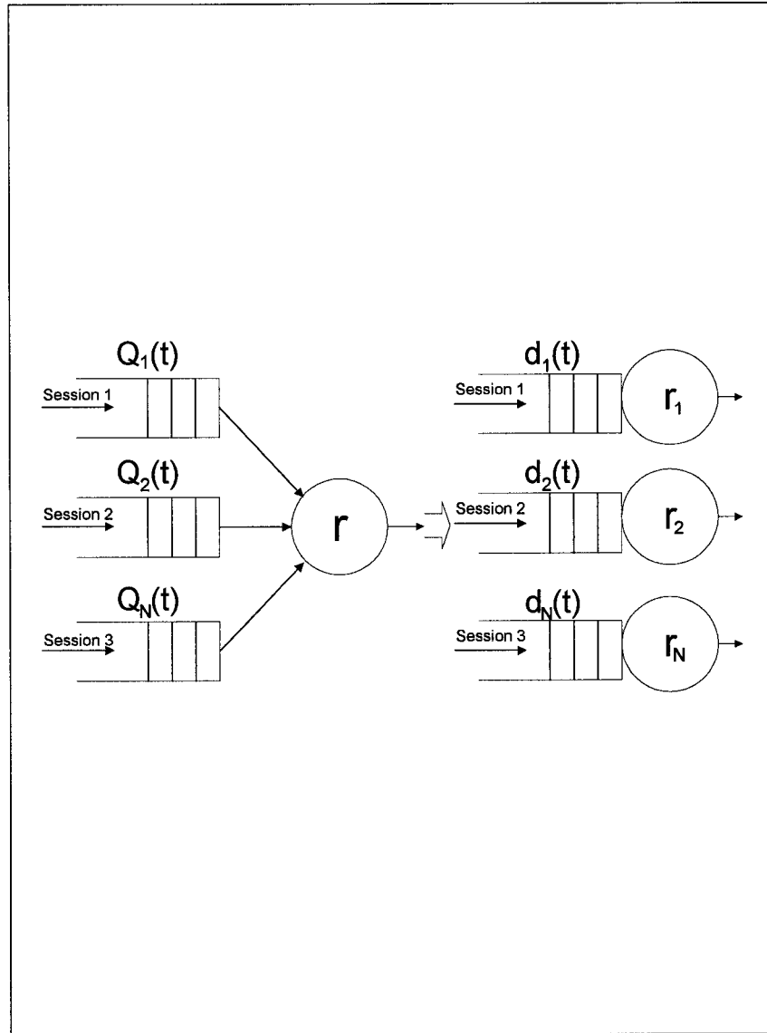
FIG. 2.2 Modèle de l'algorithme de service GPS
