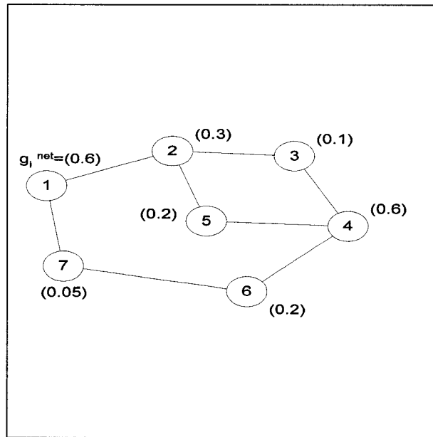
FIG. 4.3 Exemple de solution sous-optimale trouvée par l'algorithme de chemins dis-joints. Les chemins possibles pour aller de 1 à 4 sont: 1-2-3-4, 1-2-5-4 et 1-7-6-4. Si l'algorithme des chemins disjoints trouve le chemin 1-2-3-4 en premier, il devra rejeter le chemin 1-2-5-4, pourtant plus avantageux
