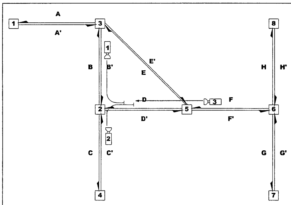
Figure 3.4: Exemple d'un conflit sur un même arc
