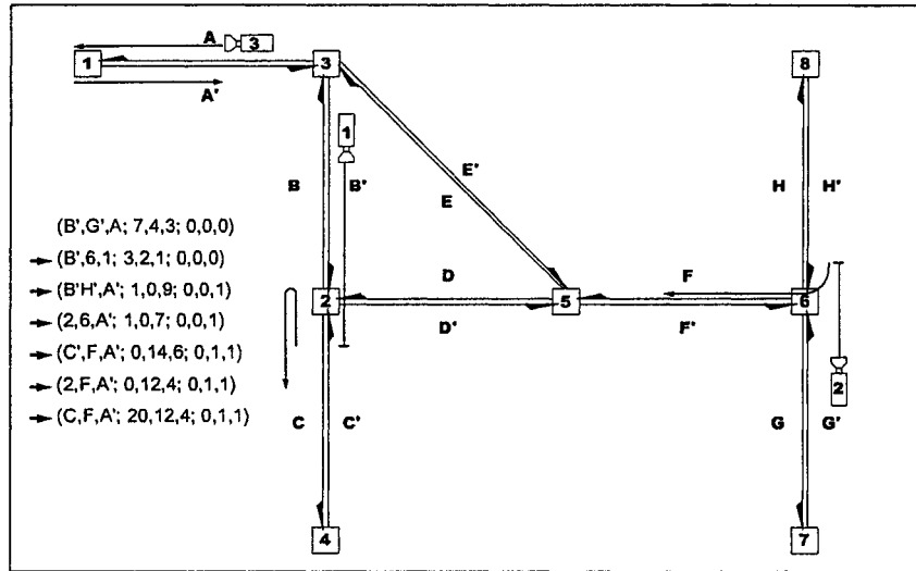
Figure 3.2: Exemples de changements d'orientation
