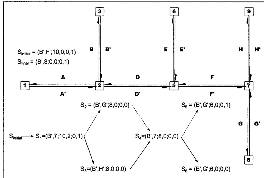
Figure 3.3: Exemple d'un état biaisé
