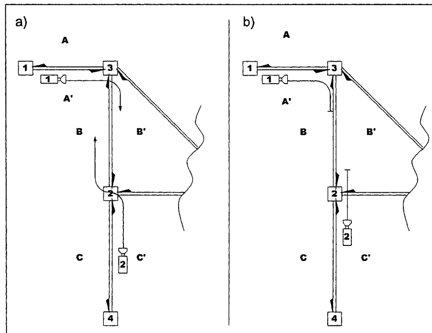
Figure 3.5: Exemples de conflits sur des arcs inverses. (a) Les véhicules traversent leur arc respectif. (b) Les véhicules se positionnent en attente.
