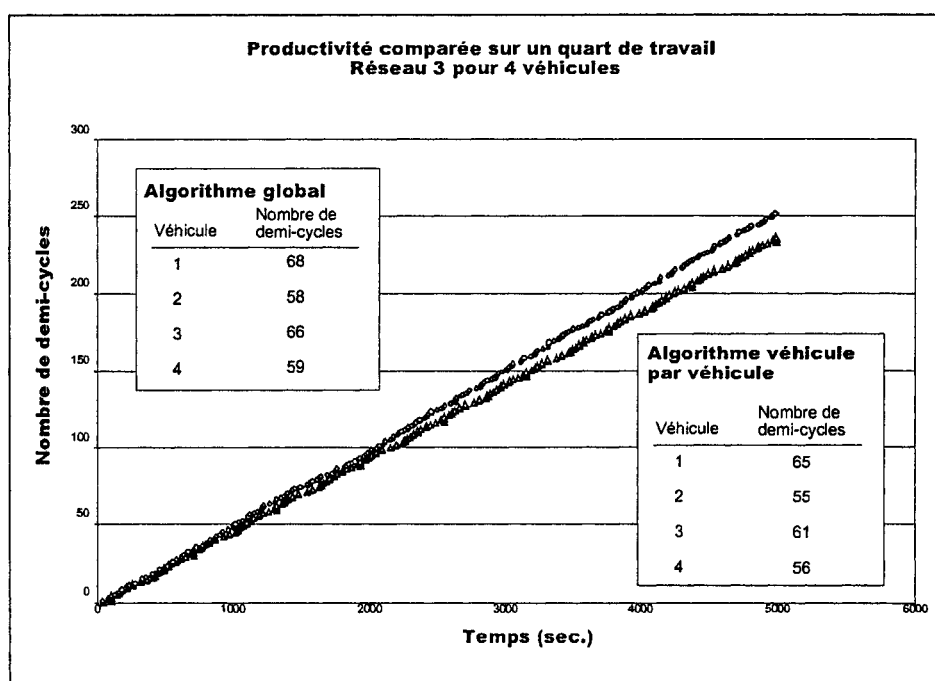
Figure 4.2: Productivité comparée sur un quart de travail, réseau 3 pour 4 véhicules
