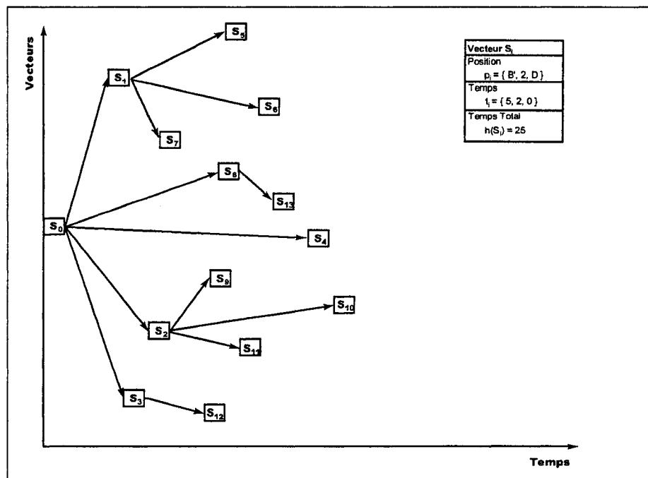
Figure 2.2: Arbre d'énumération
