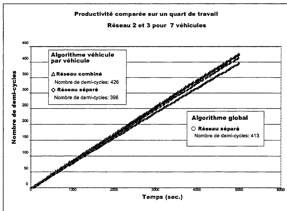
Figure 4.3: Productivité comparée sur un quart de travail, réseau 2 et 3 pour 7 véhicules
