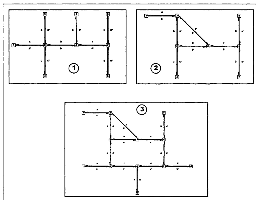
Figure 2.3: Réseaux miniers
