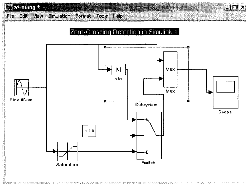
Figure 3.6 : Le modèle de la figure 3.5 une fois éclaté et ramené à un seul niveau. On constate l'absence de la boucle cyclique
