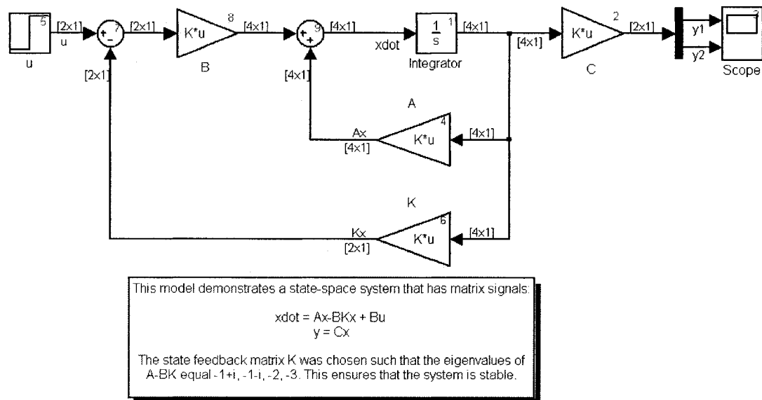
Figure 3.7 : Exemple d'un système rétroactif contenant un cycle.
