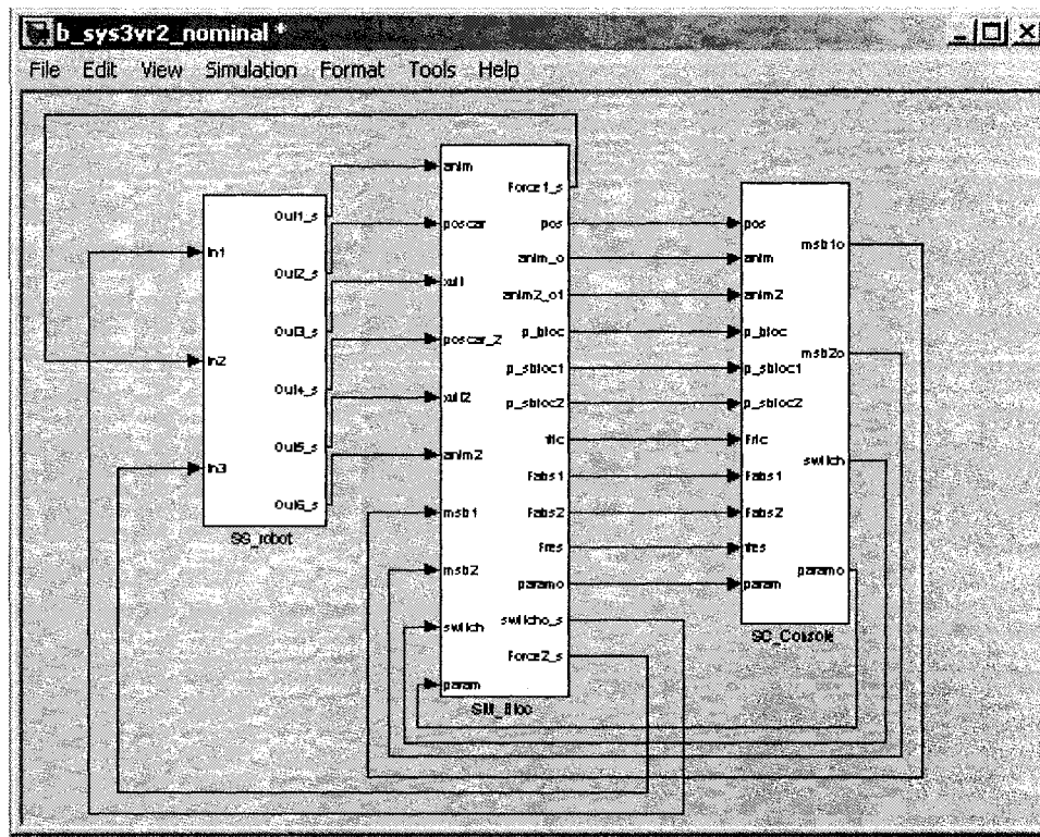
Figure 5.8 : Niveau supérieur du modèle Simulink du robot de la figure 5.7.
