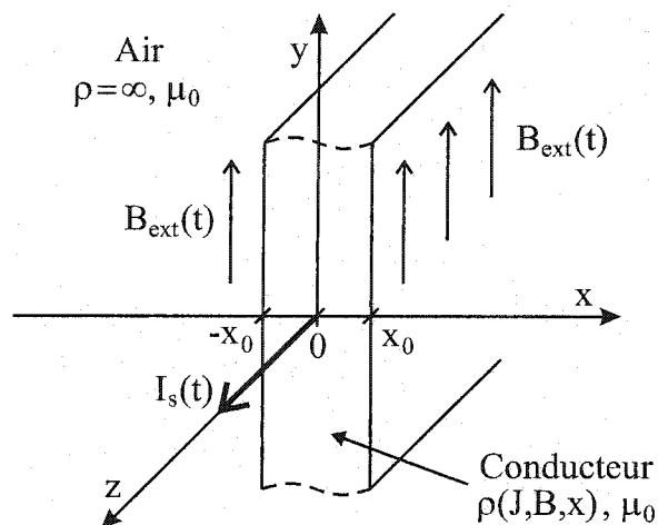
FIG. 7.1 – Géométrie 1D utilisée pour valider les méthodes numériques.
