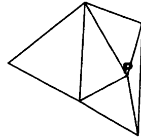
Figure 1.5: Simplexes de B_p construits et ajoutés à la triangulation pour former DT(V_{n+1})
