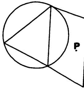
Figure 1.4: Simplexes de C_p détruits
