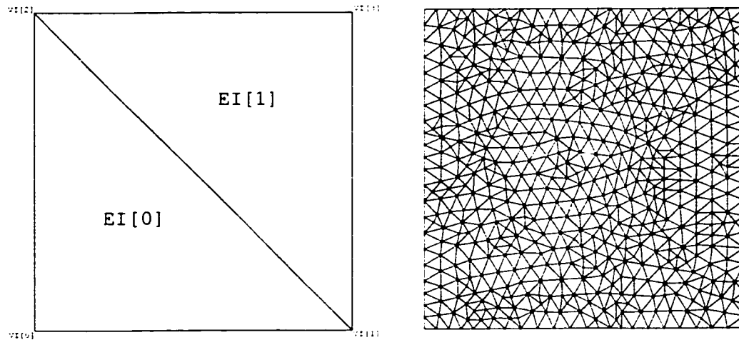
Figure 1 : Maillage d'origine et maillage résultat
