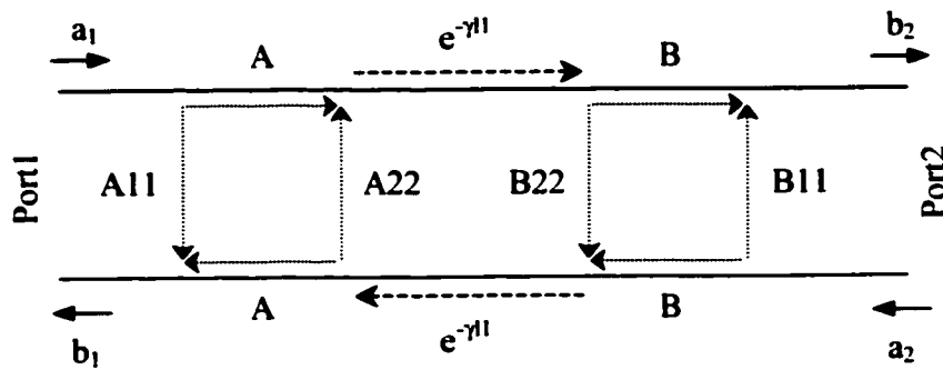
Figure 4.6 Cheminement du signal pour la connexion "THRU".
