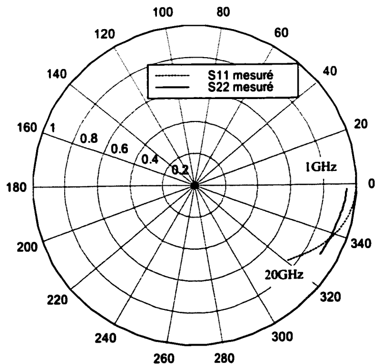
Figure 6.8 Transistor PHEMT en réflexion.
