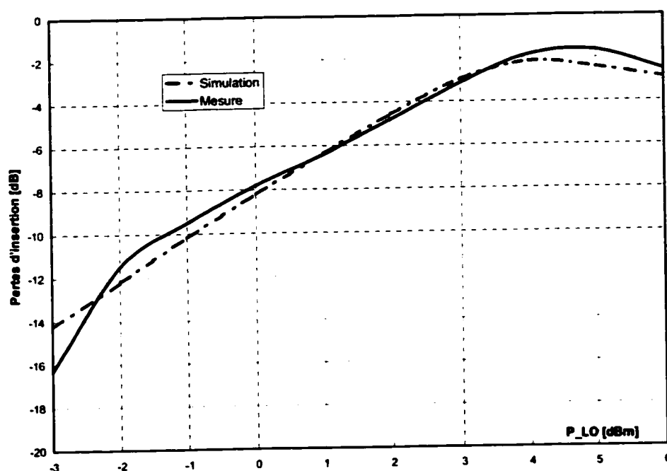
Figure 6.15 Pertes d'insertion
