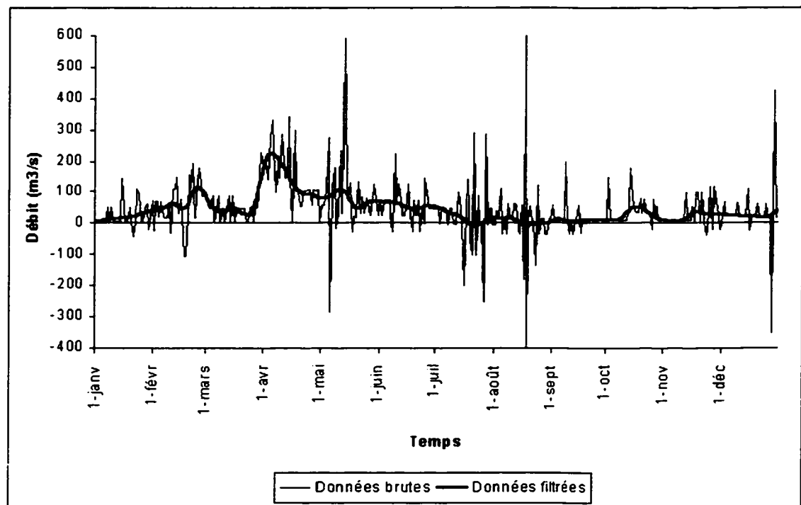
Figure 7.5: Données brutes et données filtrées au réservoir Cabonga
