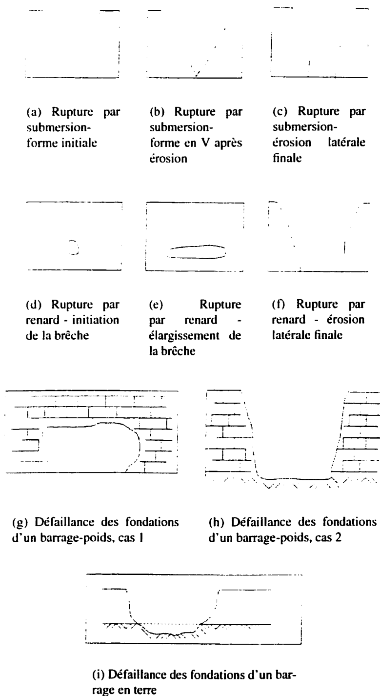
Figure 3.7: Différentes formes de brèche selon le type de rupture (Adapté de Hartford et Kartha, 1995)
