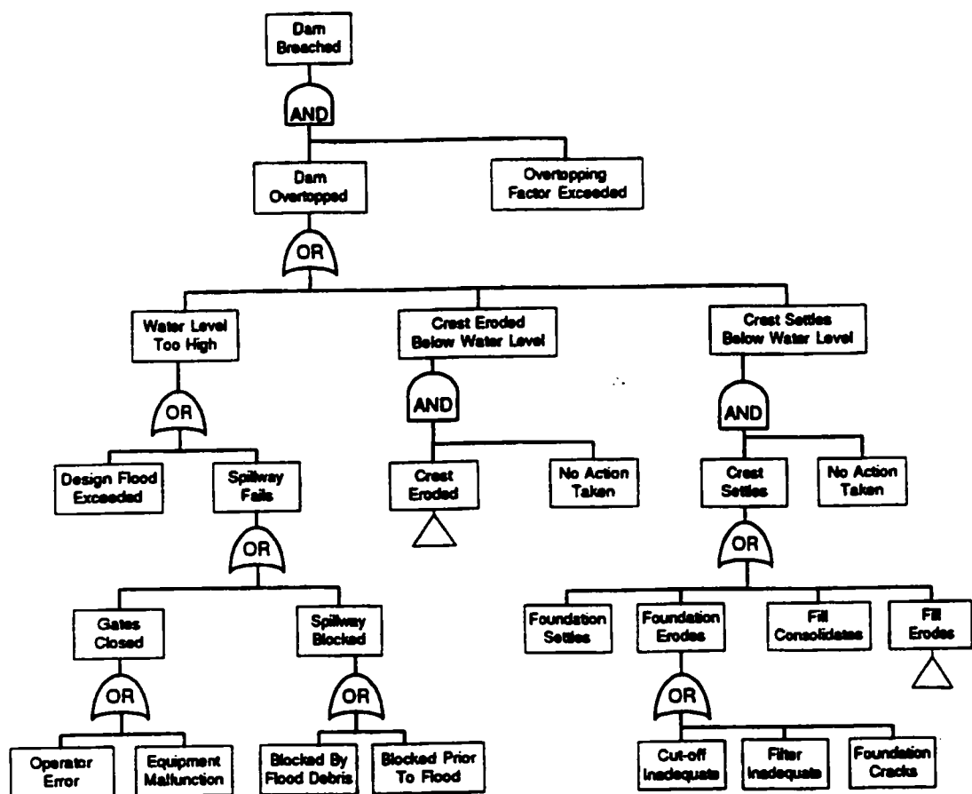
Figure 1.3: Exemple d'arbre de défaillance (Hartford et Kartha, 1995)
