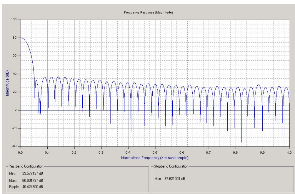
Figure 3.16 Réponse en fréquence des filtres FIR.
