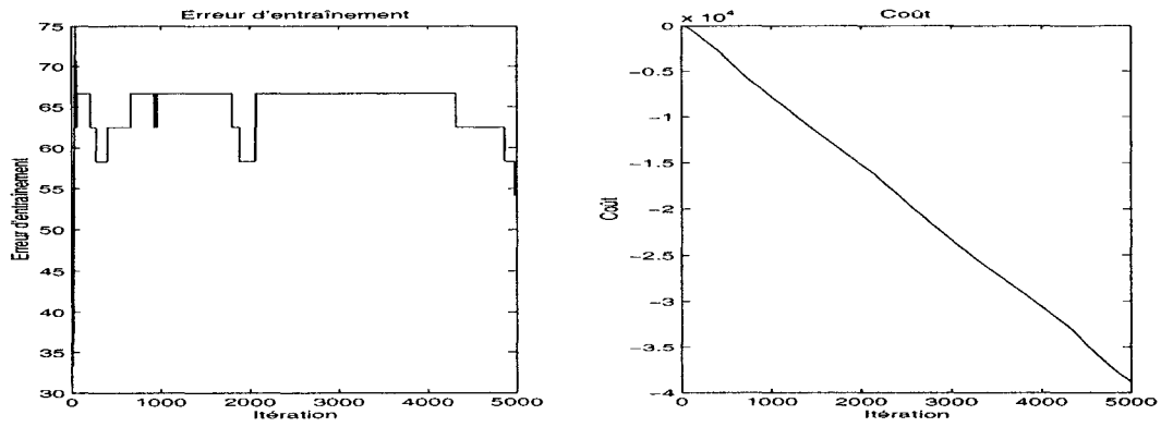
FIG. V.4 – Optimisation : Max(sortie)
