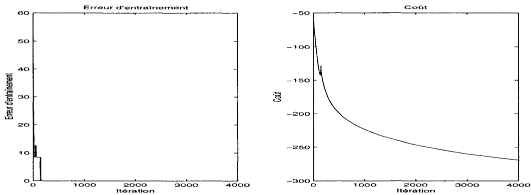
FIG. V.1 – Optimisation standard
