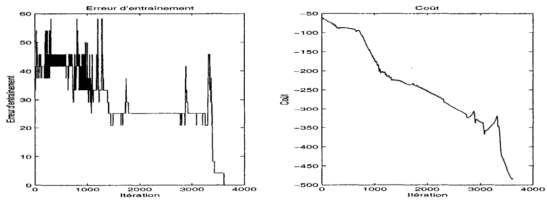
FIG. V.6 – Optimisation : Max(Gradient)
