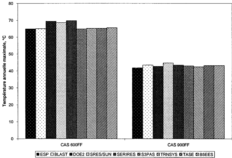
Figure 8.26 : Température annuelle maximale du cas 600FF et du cas 900FF
