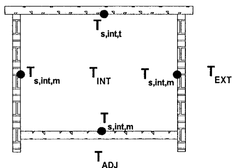
Figure 6.5 : Pièce 1 utilisée pour la validation du calcul des facteurs de forme
