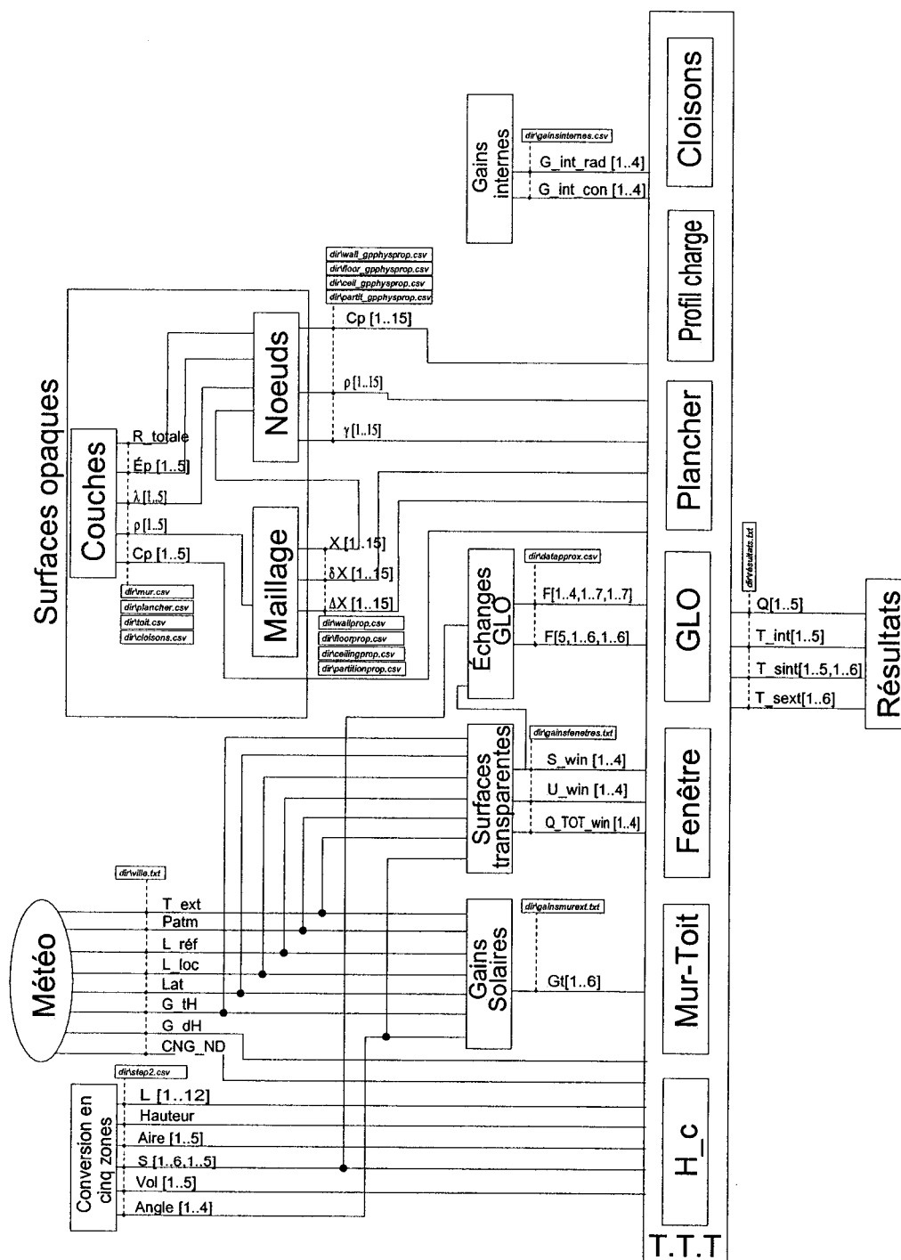
Figure 9.1 : Organisation modulaire du programme B5EES
