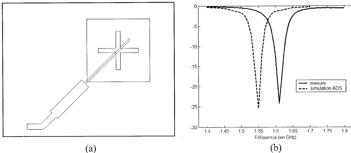
Figure 2.36 – (a) Antenne patch optimisée à 1,55 GHz (b) Coefficient de réflexion (en dB) de l'antenne patch
