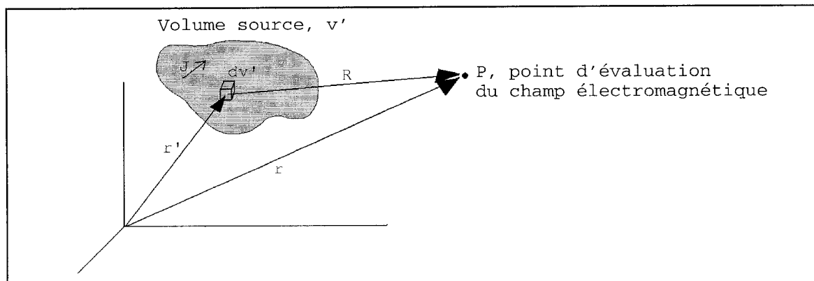
Figure 1.1 – Notations utilisées pour les problèmes de rayonnement
