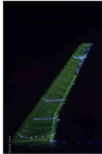
(d) \alpha = 20.7^\circ , oil-flow visualization;
