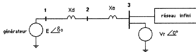
Figure 1.1: Schéma simplifié d'un alternateur connecté au réseau infini
