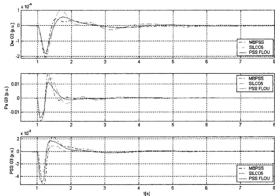
Figure 4.7a: Créneau de 1% sur Vref_G3 – Réseau K1L
