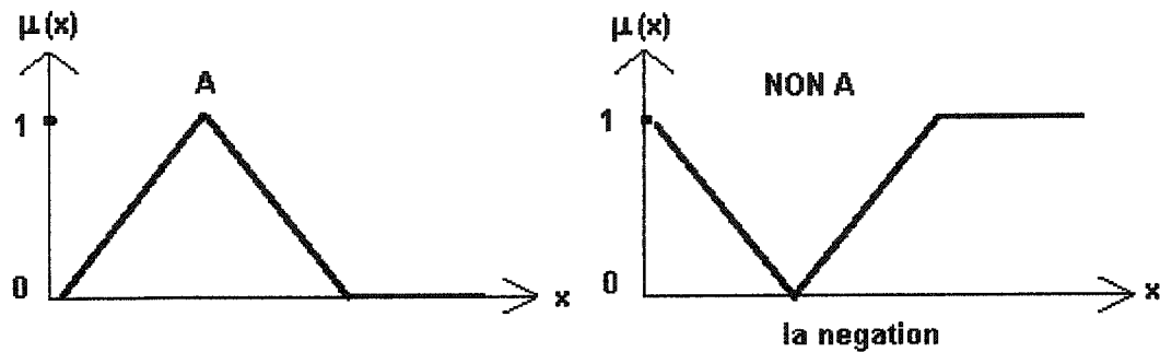
Figure 2.5: L'opérateur NON-ZADEH
